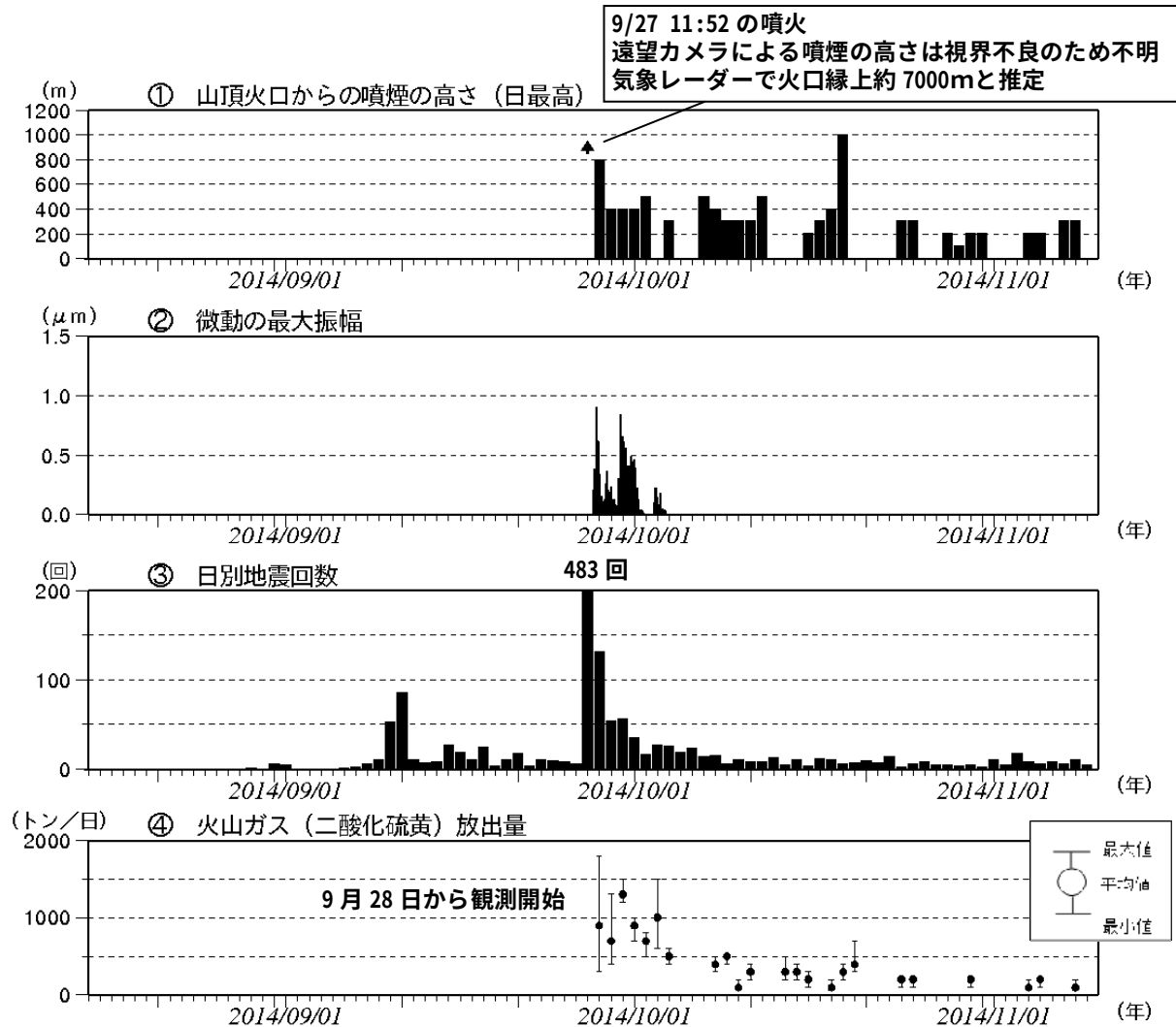
図 3 御嶽山 日別活動状況（2014 年 8 月 15 日～11 月 9 日（速報値含む））
