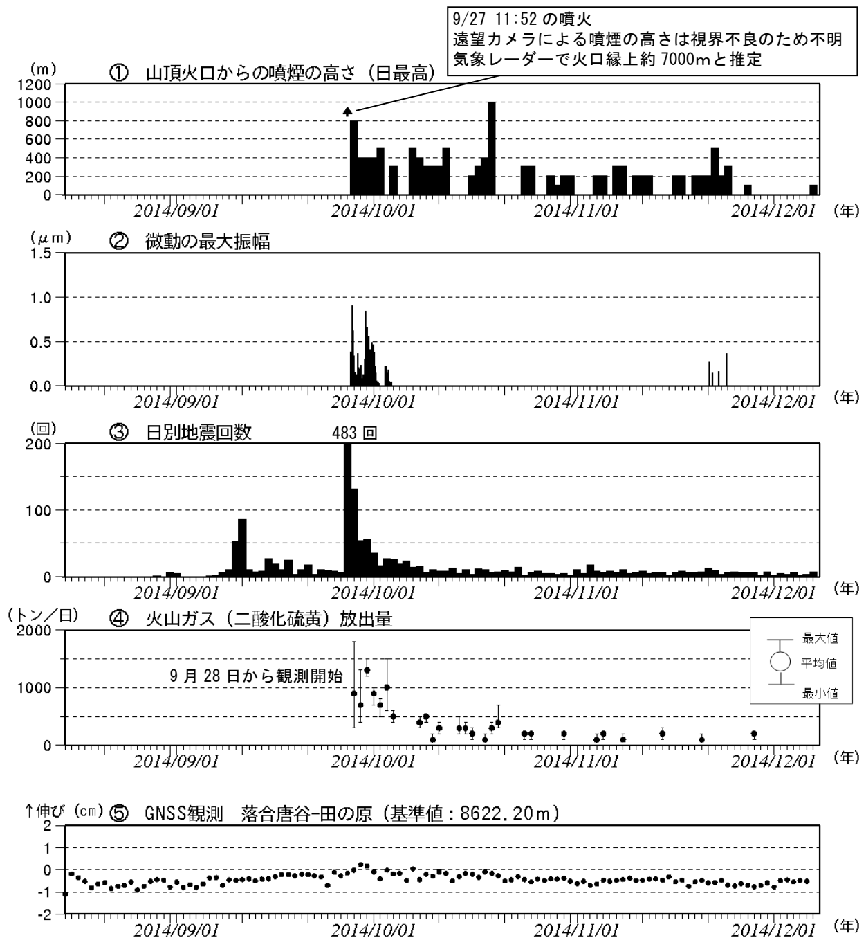
図 2 御嶽山 日別活動状況（2014 年 8 月 15 日～12 月 7 日（速報値含む））
