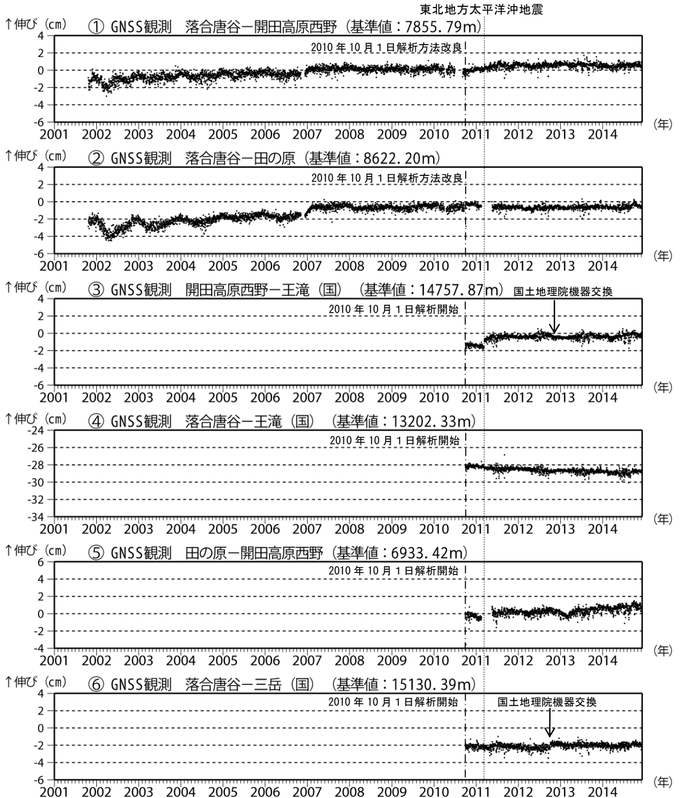
図3 御嶽山 GNSS連続観測による基線長の長期変化 (2001年1月1日~2014年12月6日)
