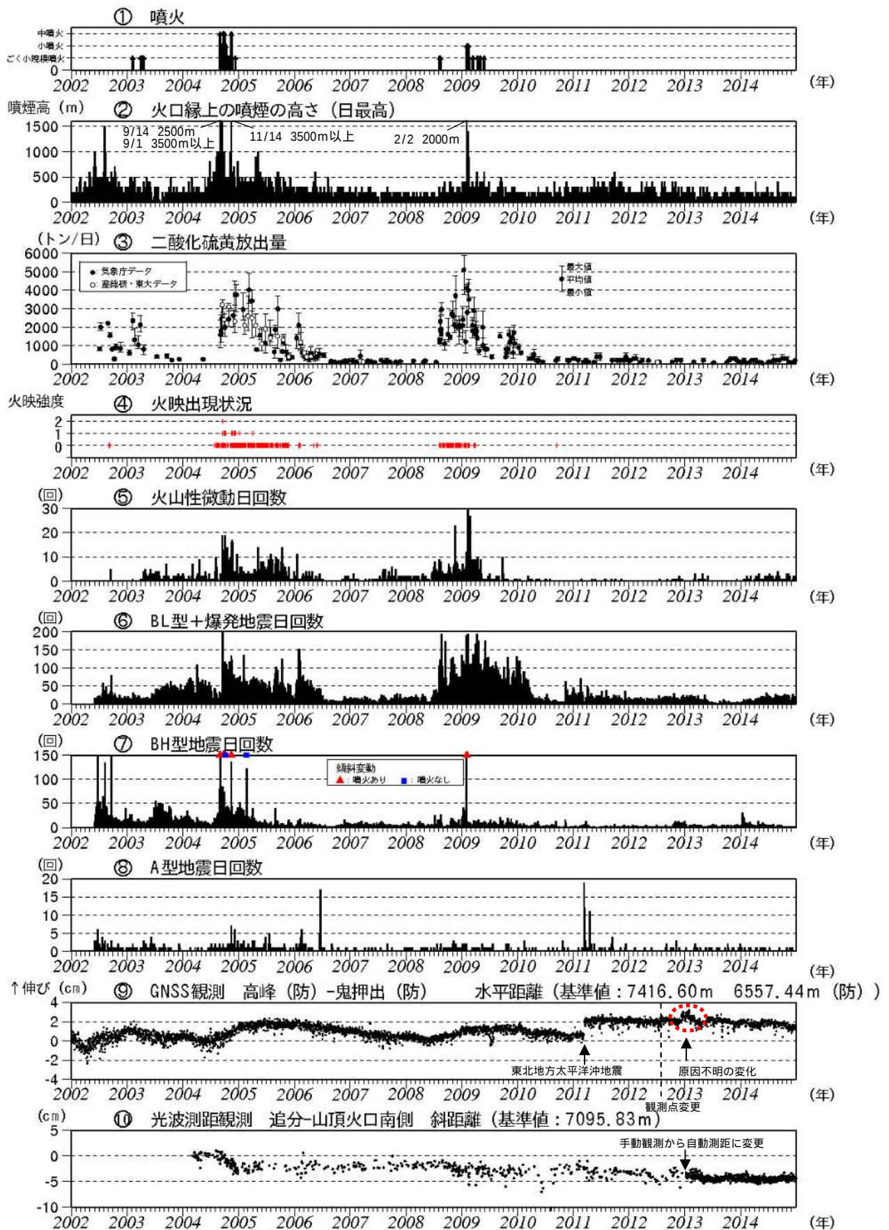
図3 浅間山 火山活動経過図 (2002年1月1日～2014年12月31日)
