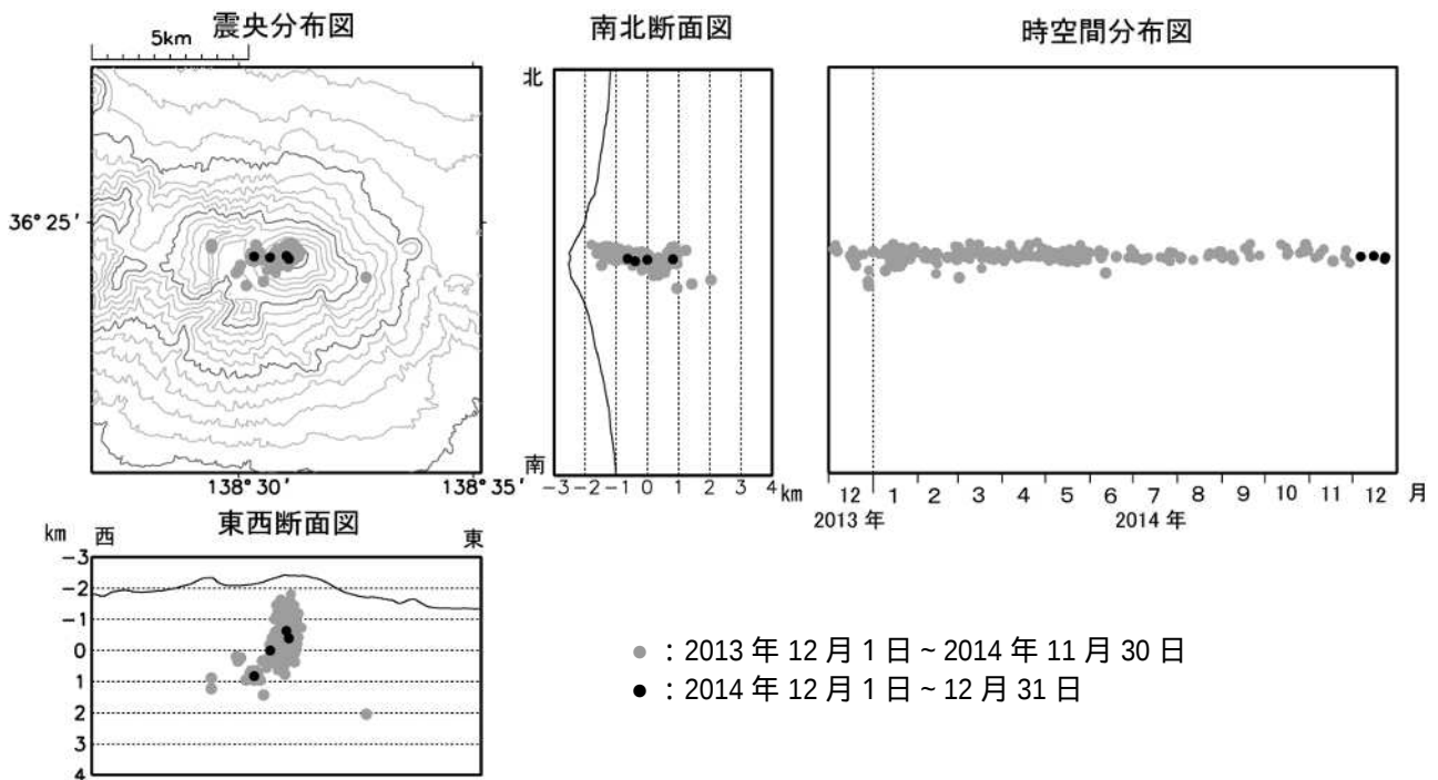
図 4 浅間山 震源分布図（2013 年 12 月 1 日～2014 年 12 月 31 日）
