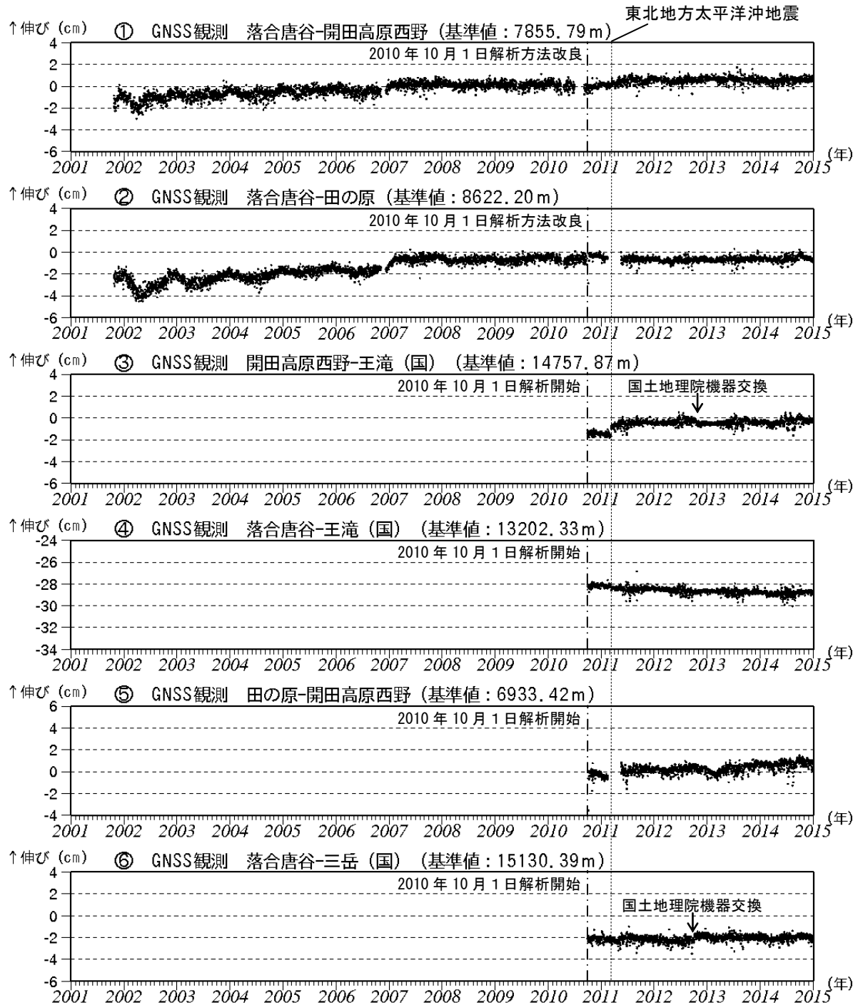
図3 御嶽山 GNSS 連続観測による基線長の長期変化 (2001 年 1 月 1 日～2015 年 1 月 3 日)
