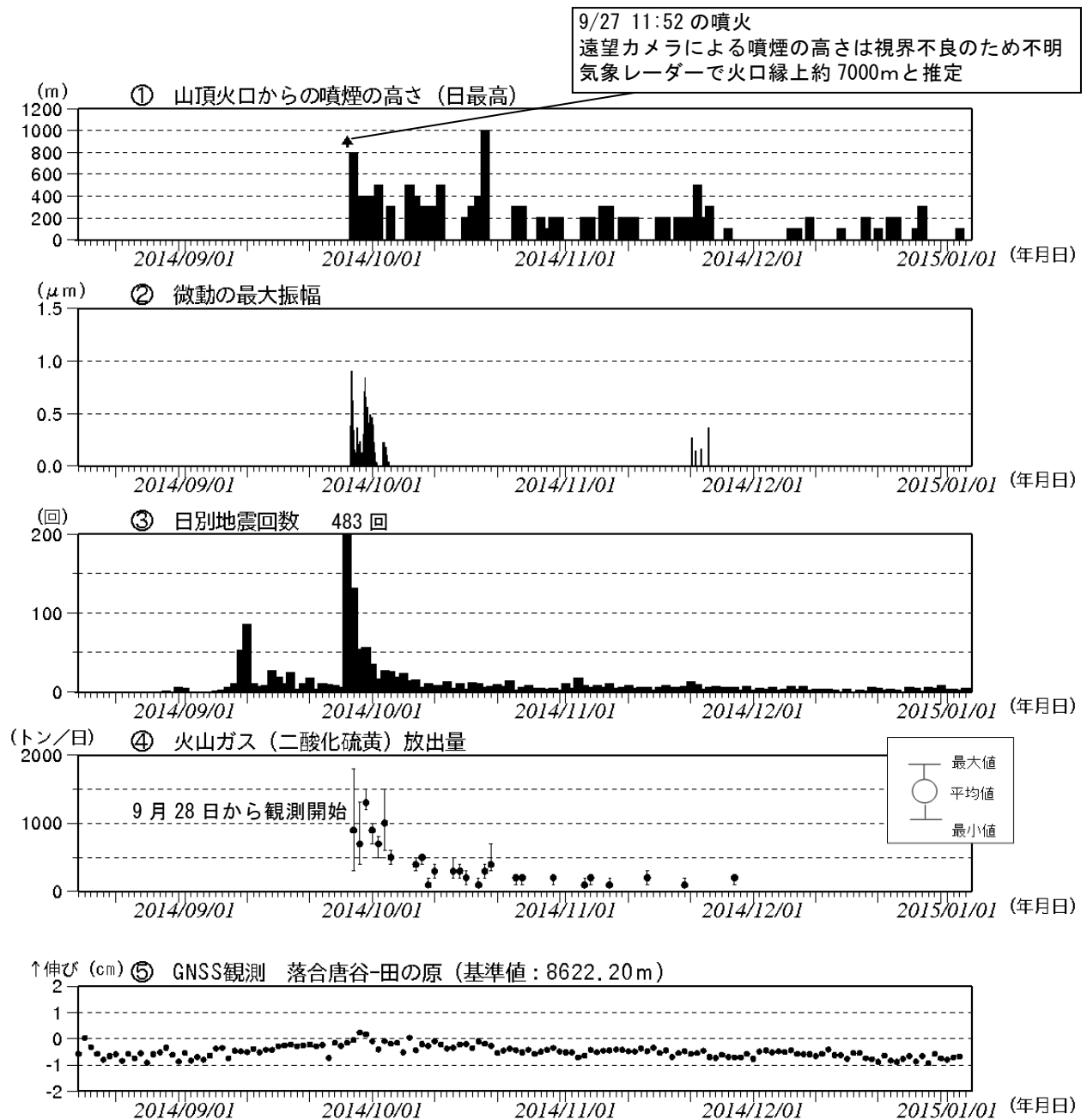
図 2 御嶽山 日別活動状況（2014 年 8 月 15 日～2015 年 1 月 4 日（速報値含む））
