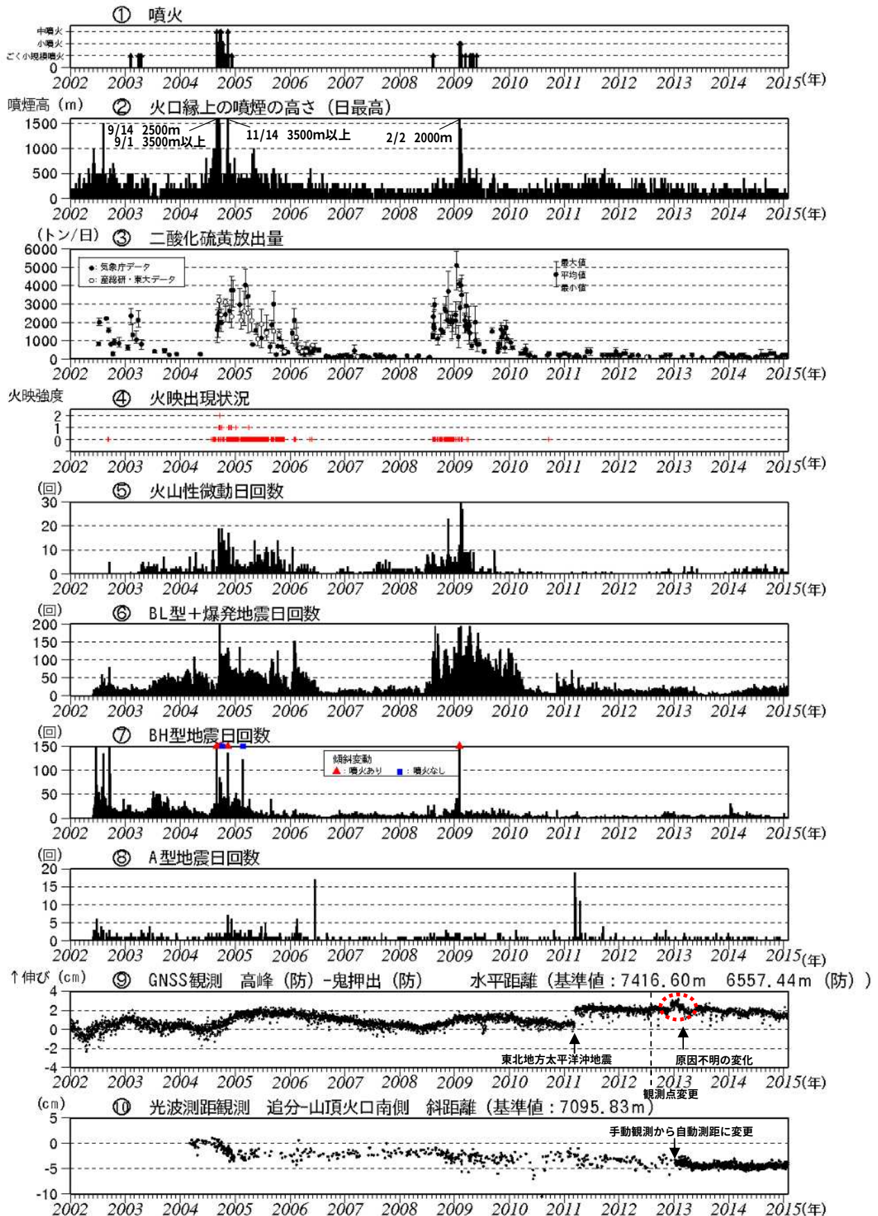
図3 浅間山 火山活動経過図 (2002年1月1日～2015年1月31日)
