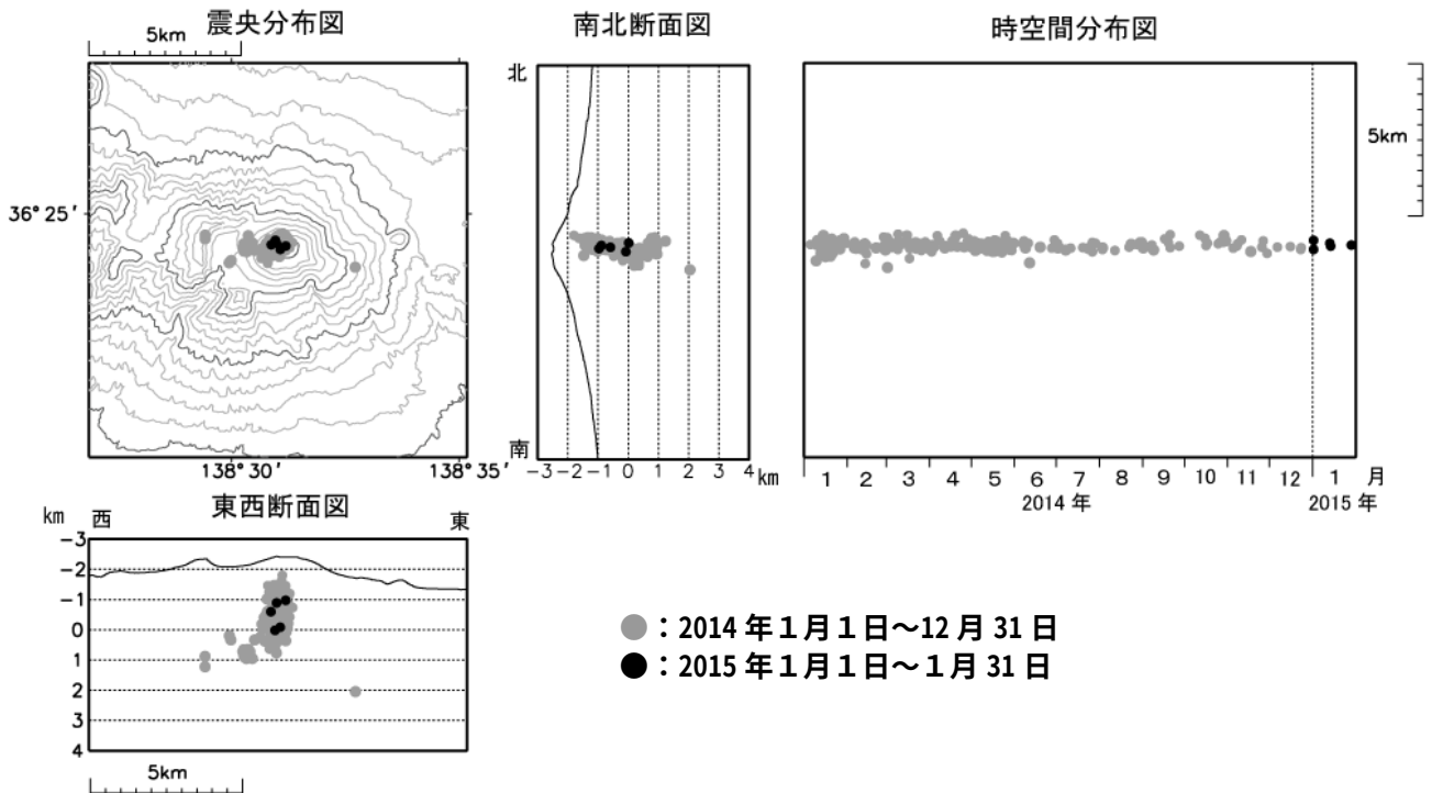
図 4 浅間山 震源分布図（2014 年 1 月 1 日～2015 年 1 月 31 日）
