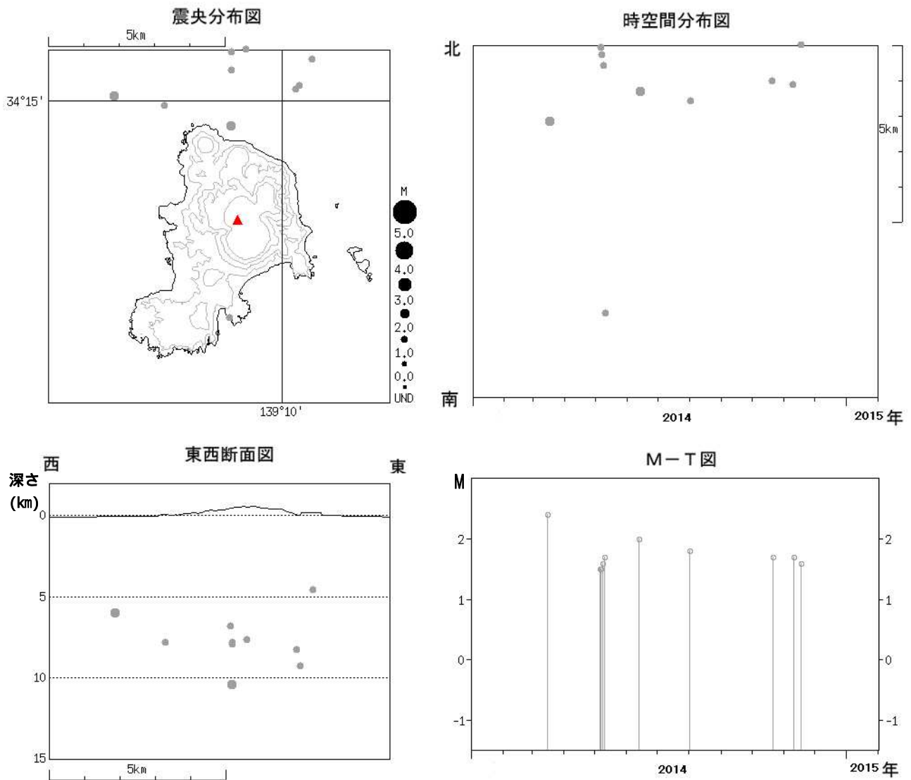
図 4 神津島 広域地震観測網による山体・周辺の地震活動（2014 年 1 月 1 日～2015 年 1 月 31 日）
