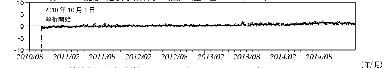
図 3 神津島 火山活動経過図(2010 年 8 月 2 日～2015 年 1 月 31 日)
