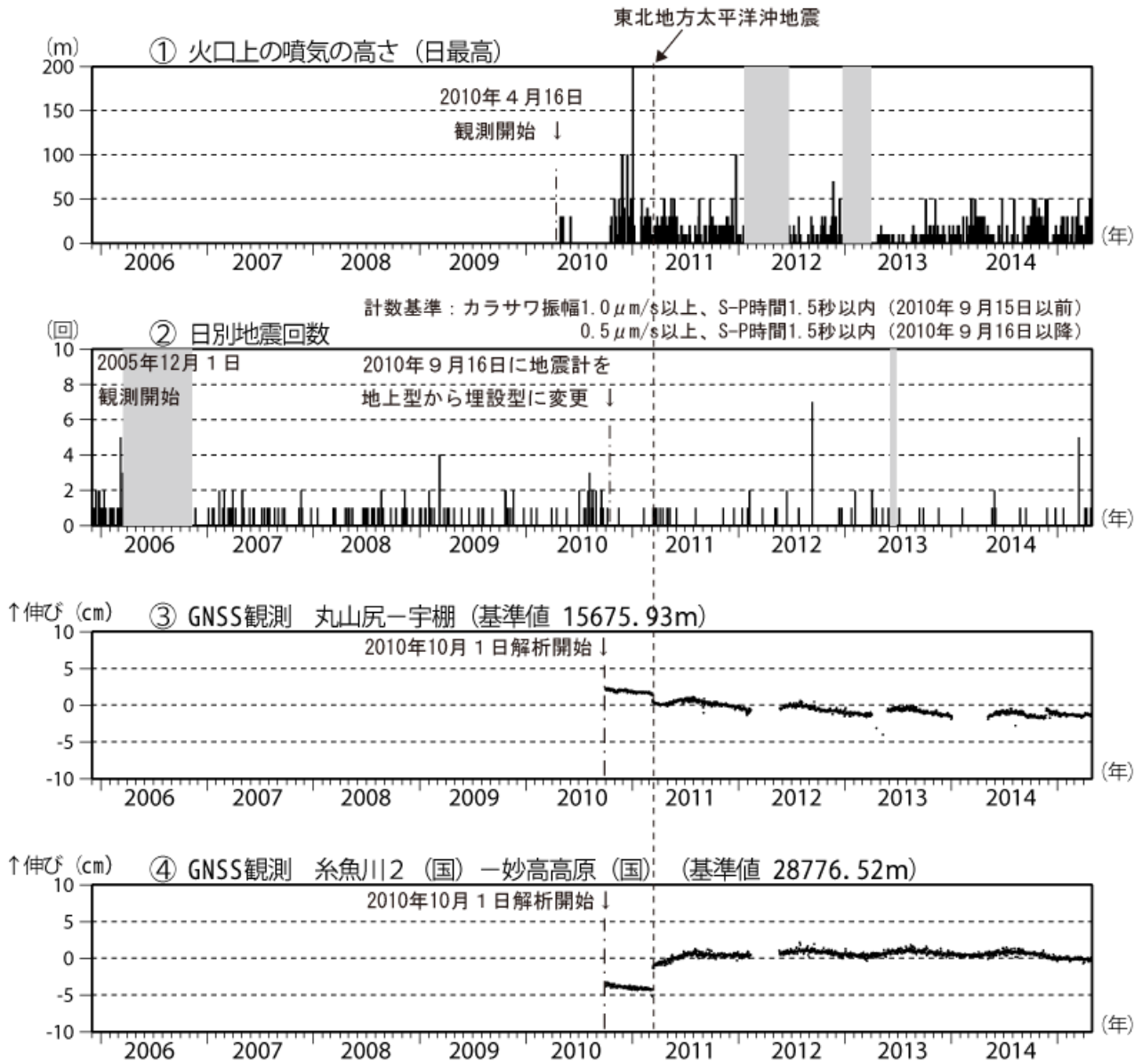
図3 新潟焼山 火山活動経過図（2005年12月1日～2015年4月30日）
