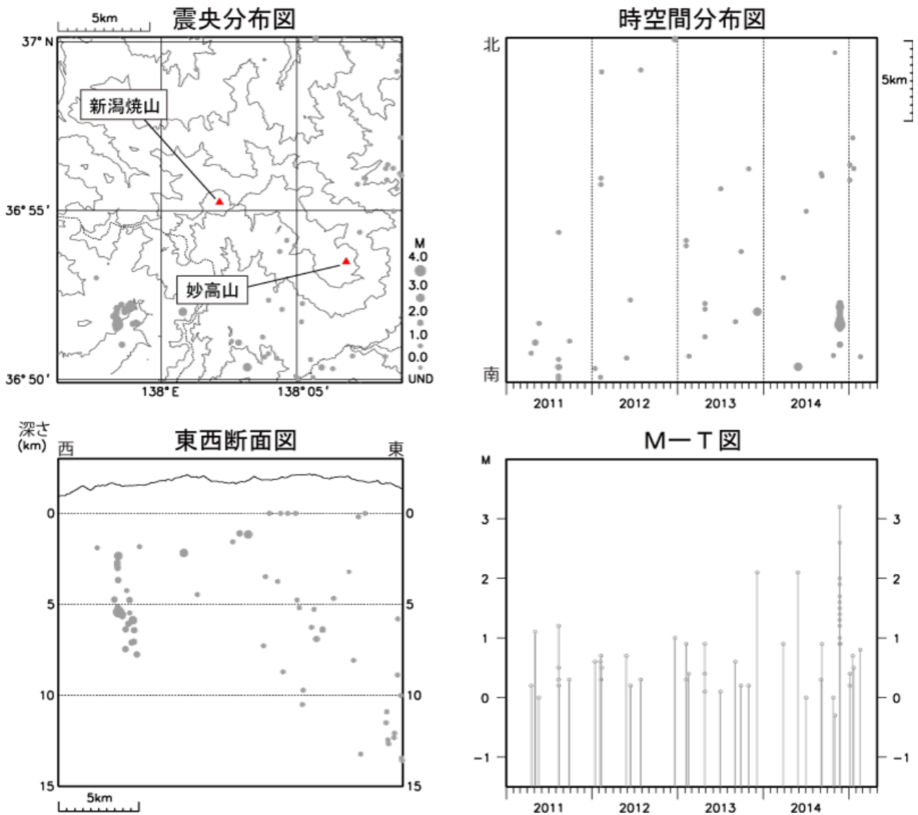
図 4 新潟焼山 広域地震観測網による山体・周辺の地震活動（2011 年 1 月 1 日～2015 年 4 月 30 日）
