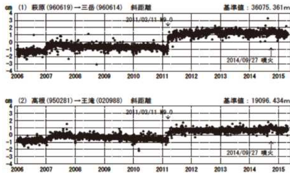
図6 御嶽山 国土地理院によるGNSS基線変化グラフ 4)
