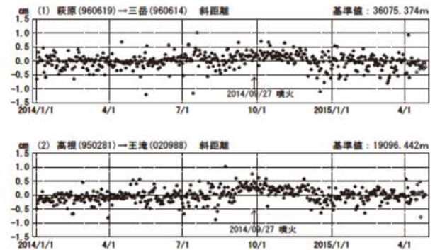
図6 御嶽山 国土地理院によるGNSS基線変化グラフ 4)
