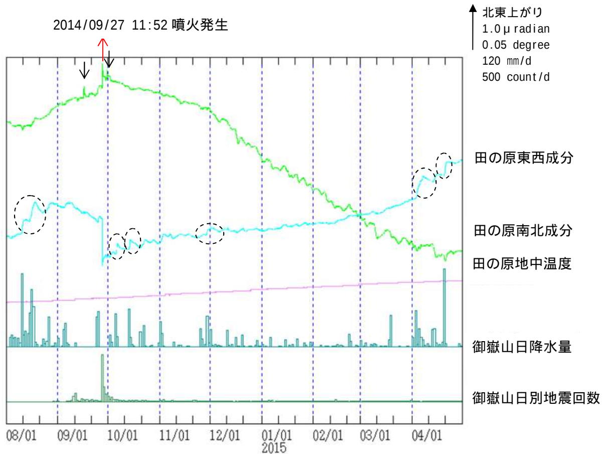
図5 御嶽山 田の原観測点（剣ヶ峰山頂の南東約3 km）の傾斜変動 （2014年8月1日～2015年4月30日）
