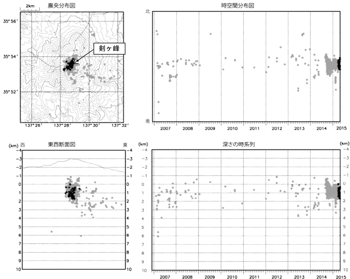
図 2 御嶽山 震源分布図（2006 年 12 月 1 日～2015 年 4 月 30 日）
