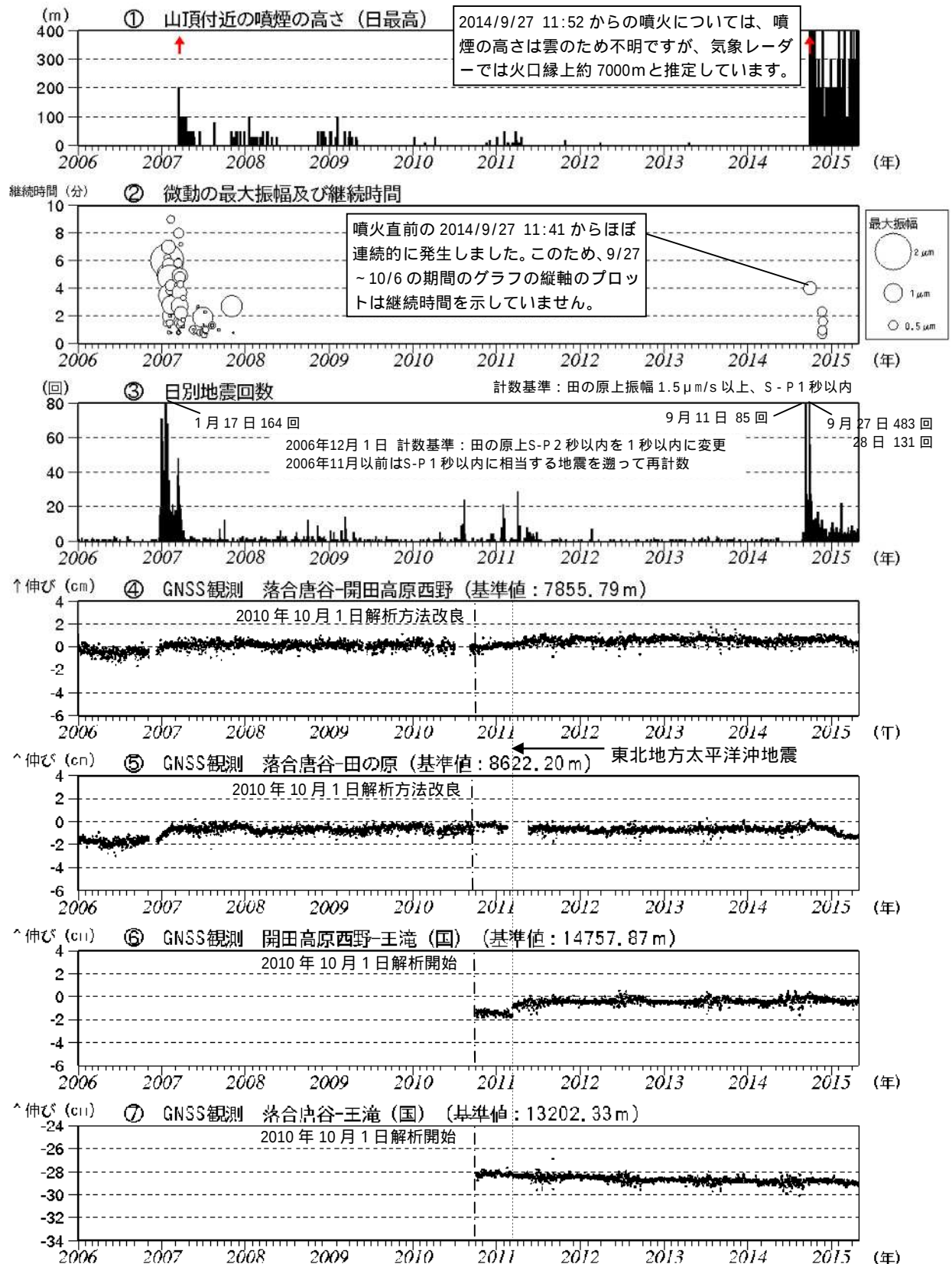
図4 御嶽山 長期間の火山活動経過図（2006年1月1日～2015年4月30日）
