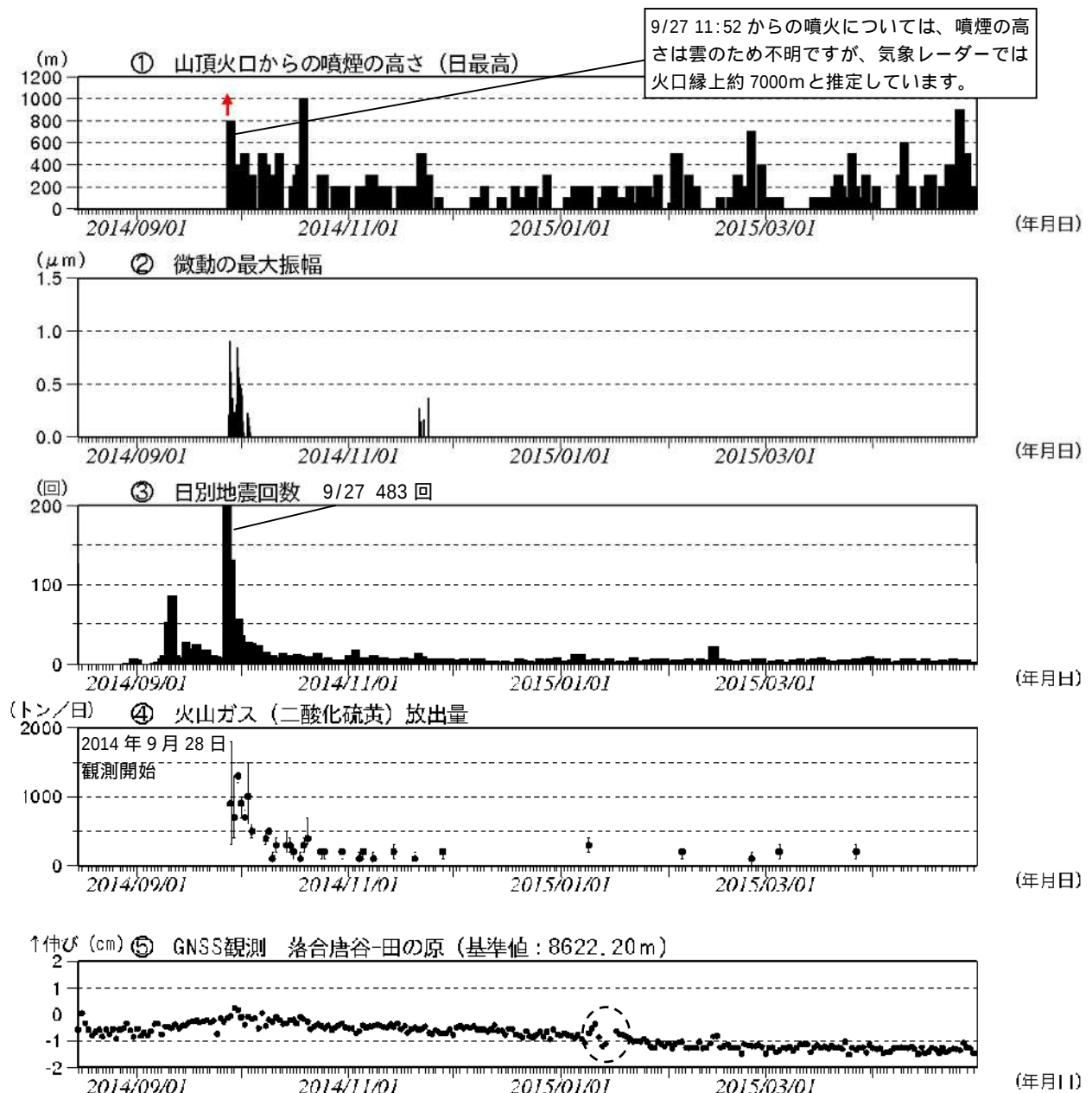
図 3 御嶽山 最近の火山活動経過図（2014 年 8 月 15 日～2015 年 4 月 30 日）
