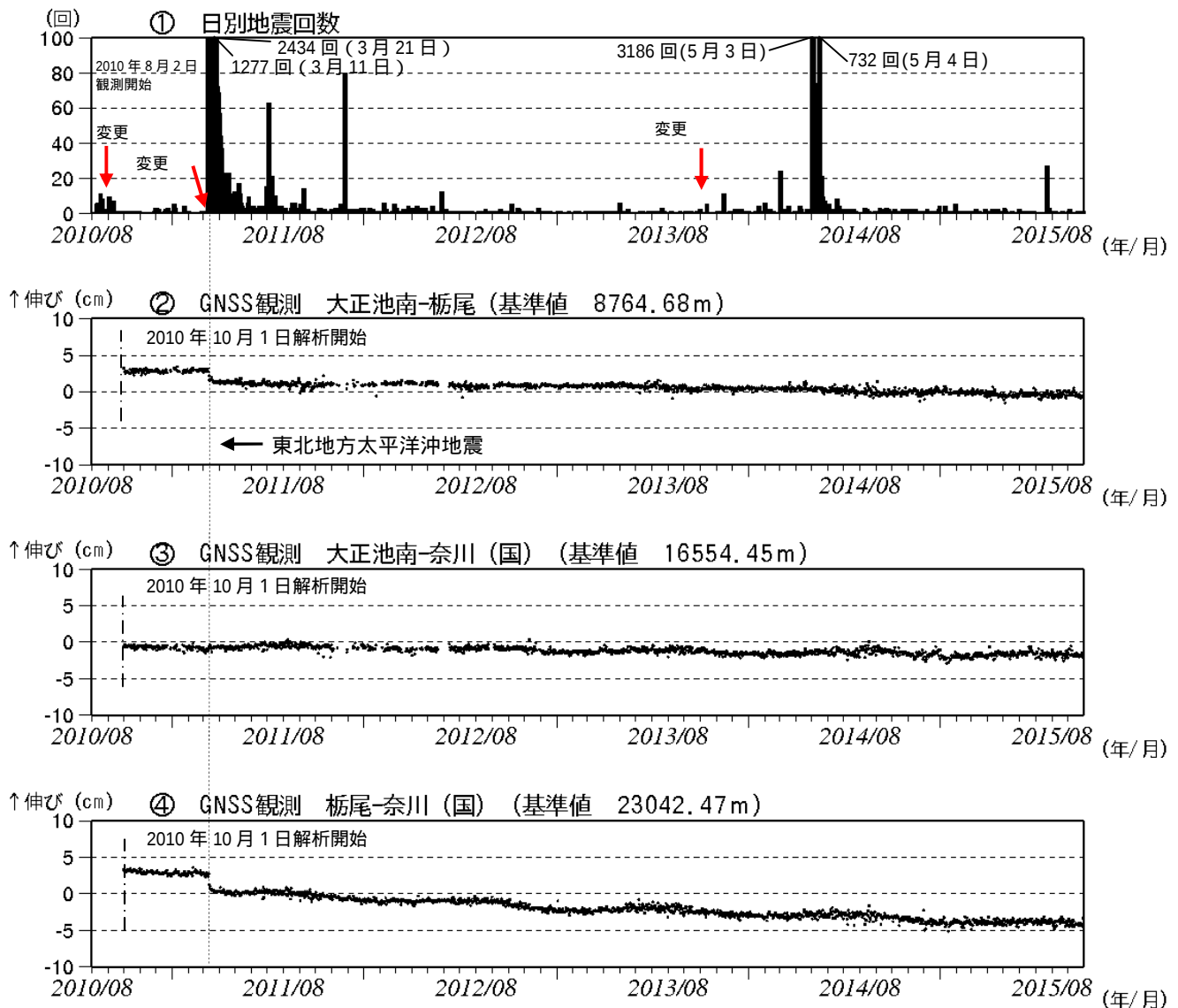
図 2 焼岳 火山活動経過図（2010年 8 月 2 日～2015年 9 月30日）
