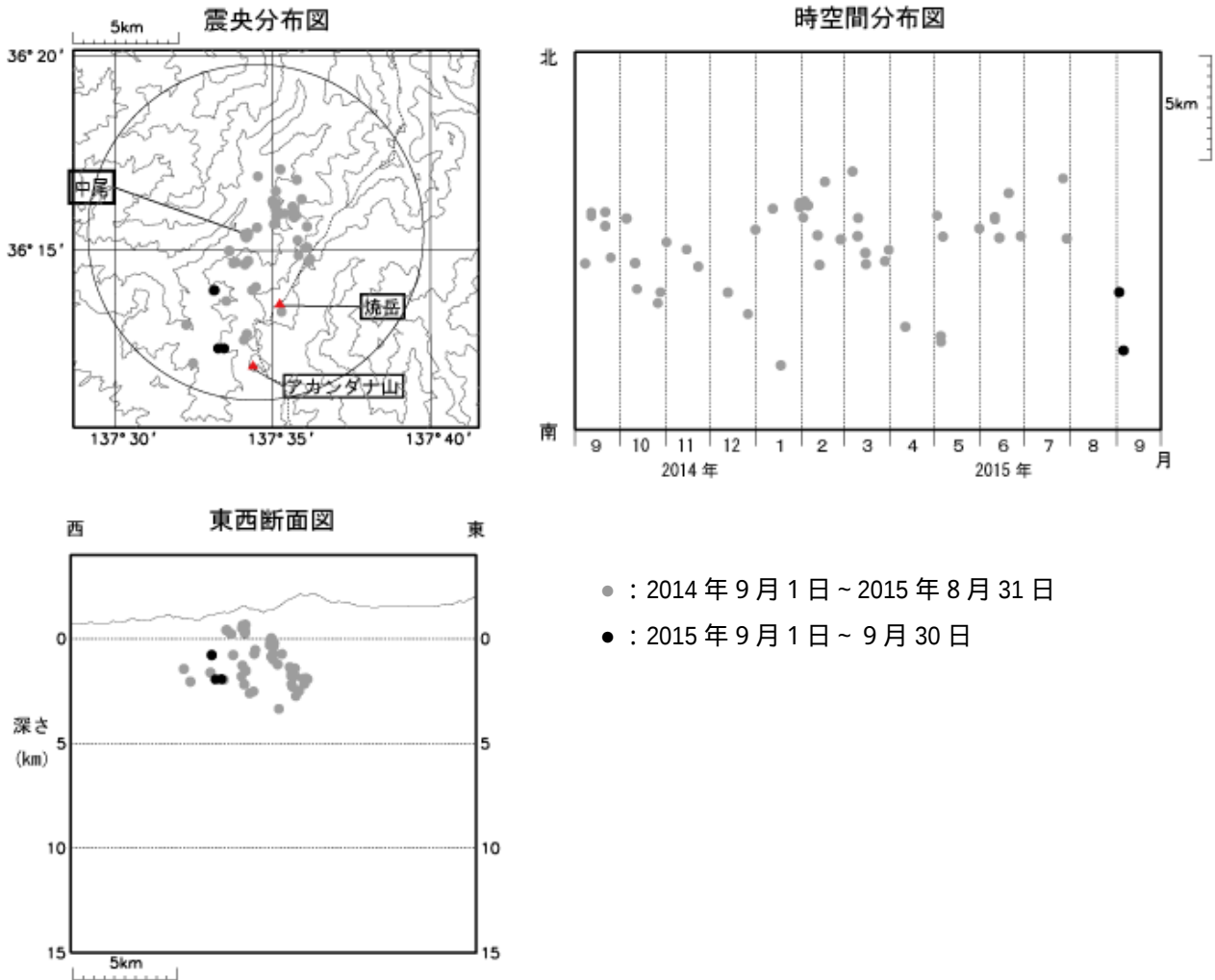
図 3 焼岳 震源分布図（2014 年 9 月 1 日～2015 年 9 月 30 日）
