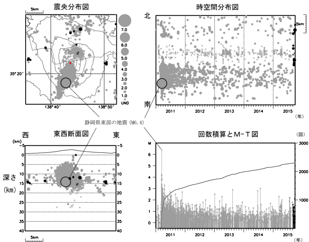
図 3 富士山 広域地震観測網による山体・周辺の地震活動 (2011 年 1 月 1 日 ~ 2015 年 9 月 30 日)
