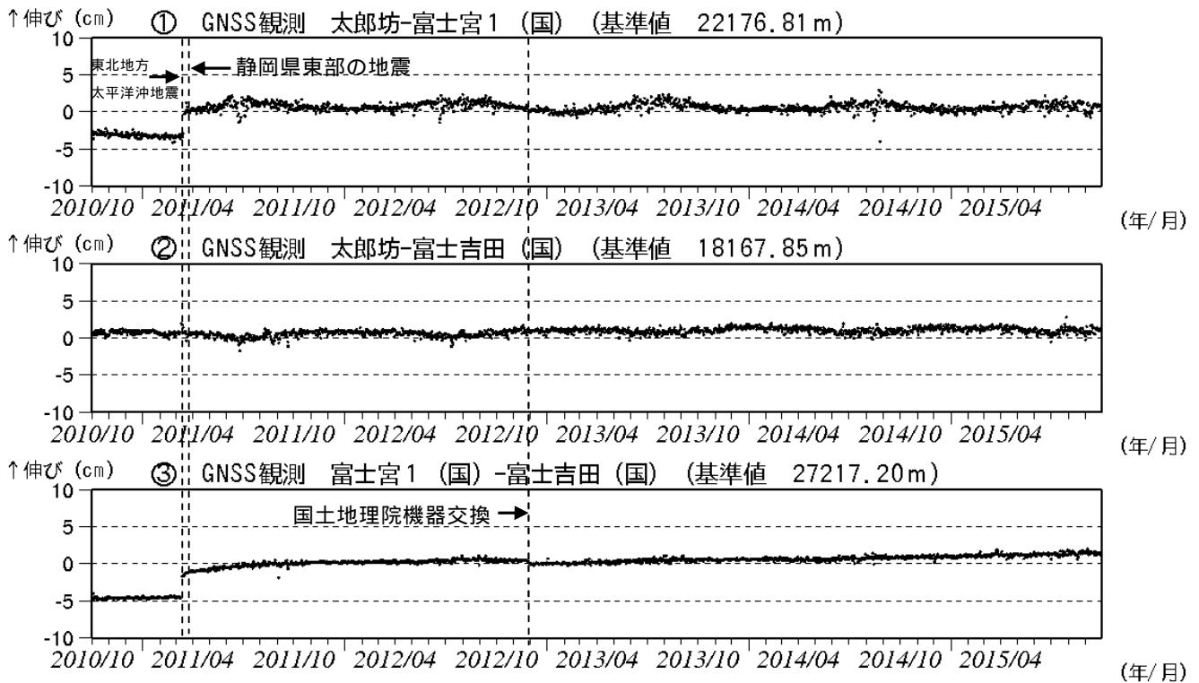
図4 富士山 GNSS 連続観測による基線長変化 (2010 年 10 月 1 日～2015 年 9 月 30 日) (国): 国土地理院
