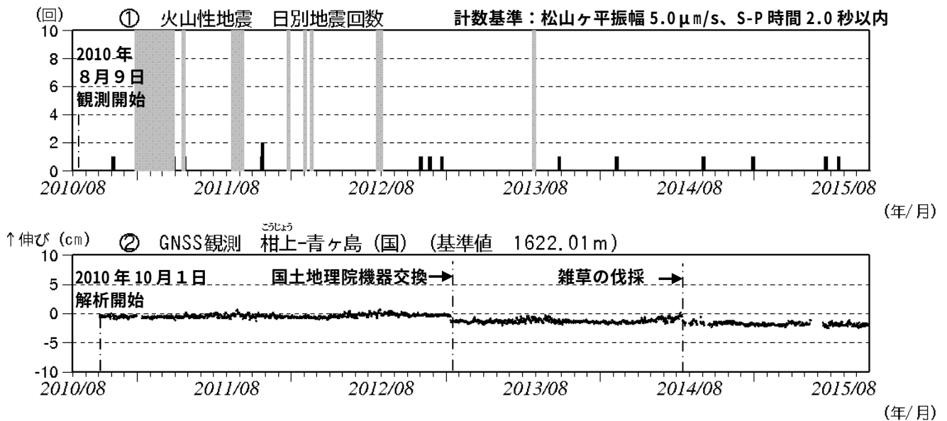
図2 青ヶ島 火山活動経過図 (2010年8月9日～2015年9月30日)
