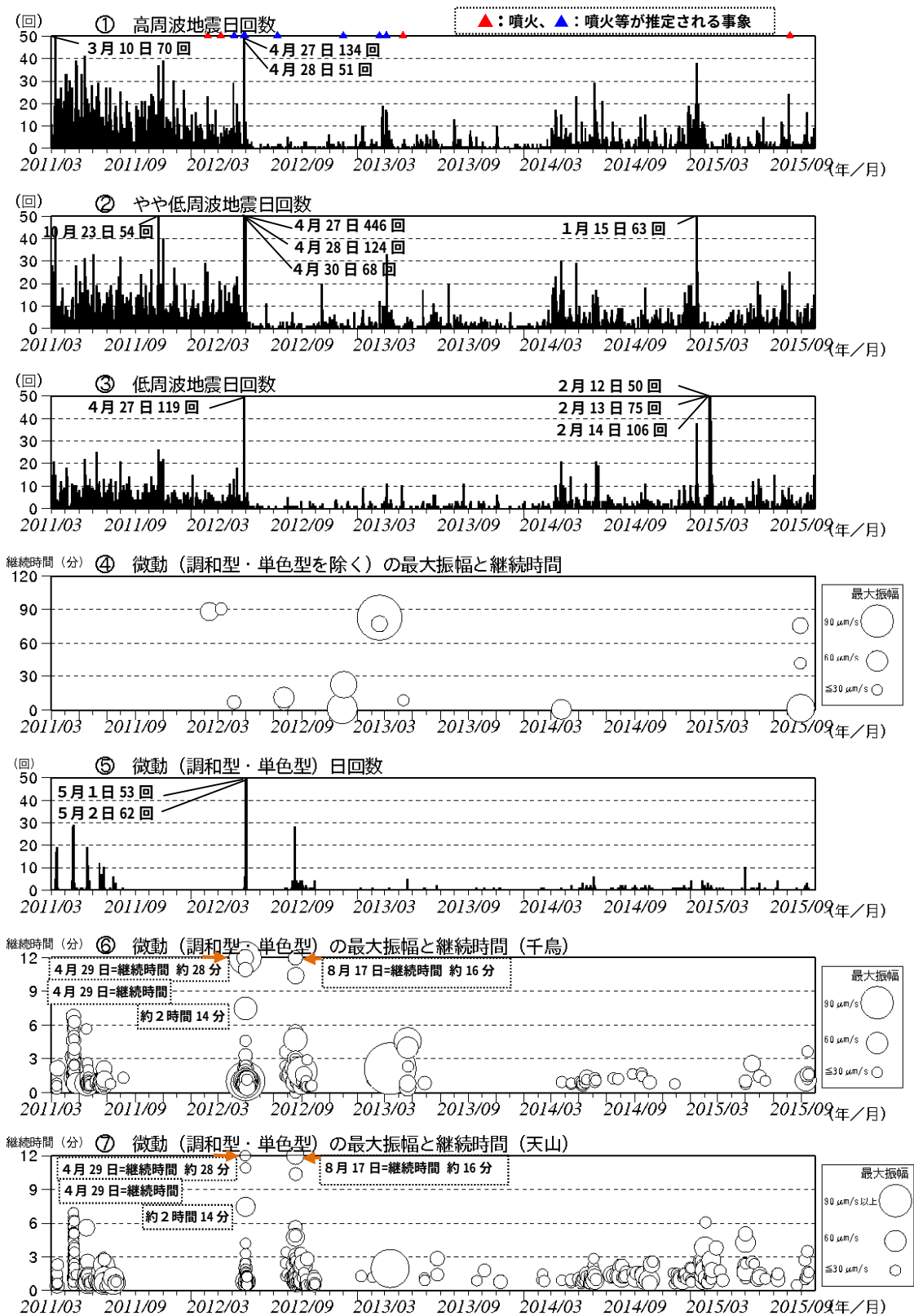
図5 硫黄島 火山活動経過図（2011年3月8日～2015年9月30日）
