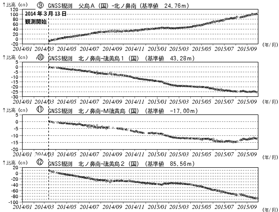
図7 硫黄島 GNSS 1) 観測結果(2014年1月～2015年9月) (国):国土地理院
