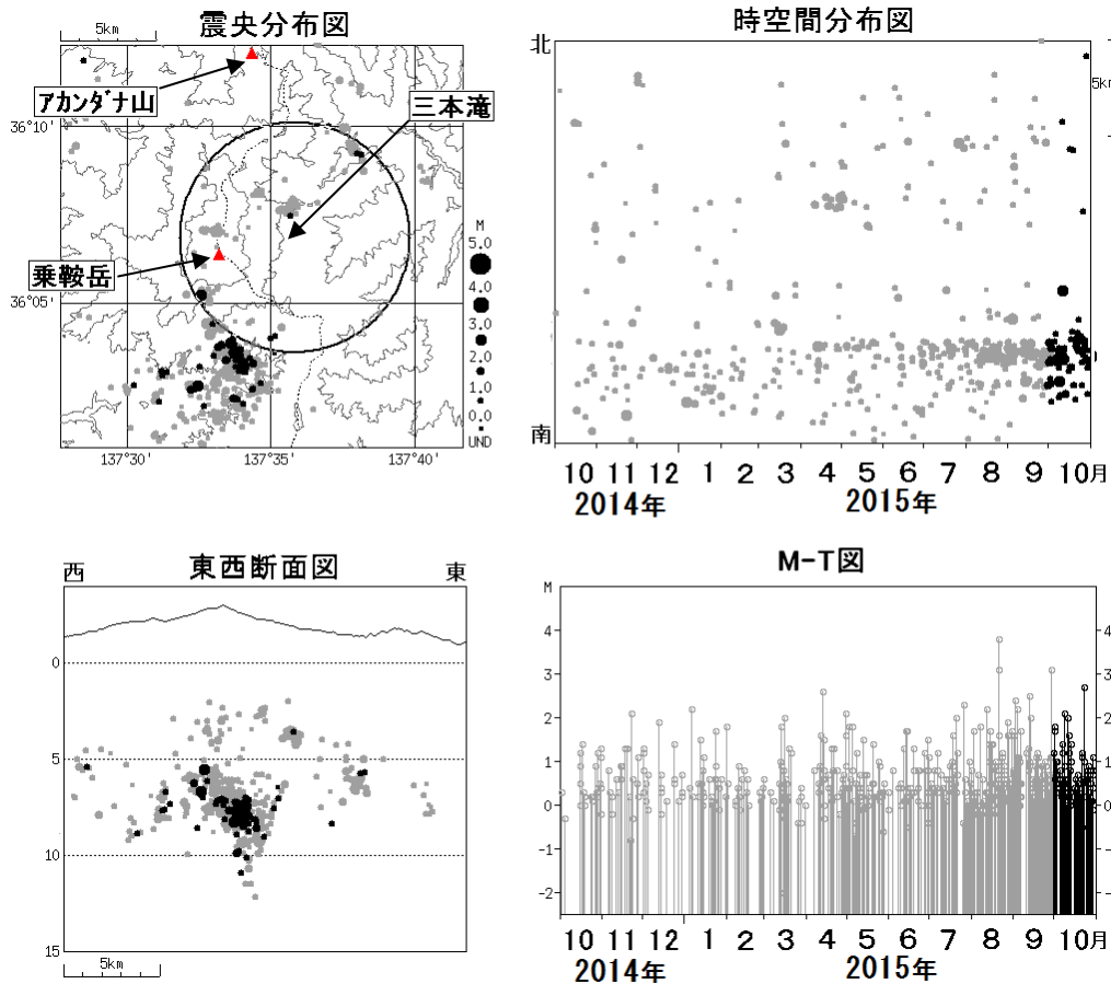
図 3 乗鞍岳 広域地震観測網による山体・周辺の地震活動(2014 年 10 月 1 日～2015 年 10 月 31 日)
