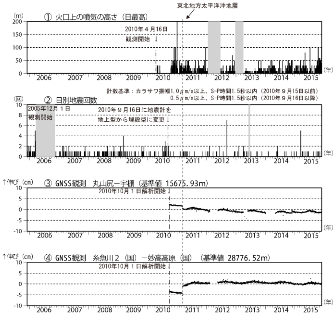
図3 新潟焼山 火山活動経過図（2005年12月1日～2015年11月30日）
