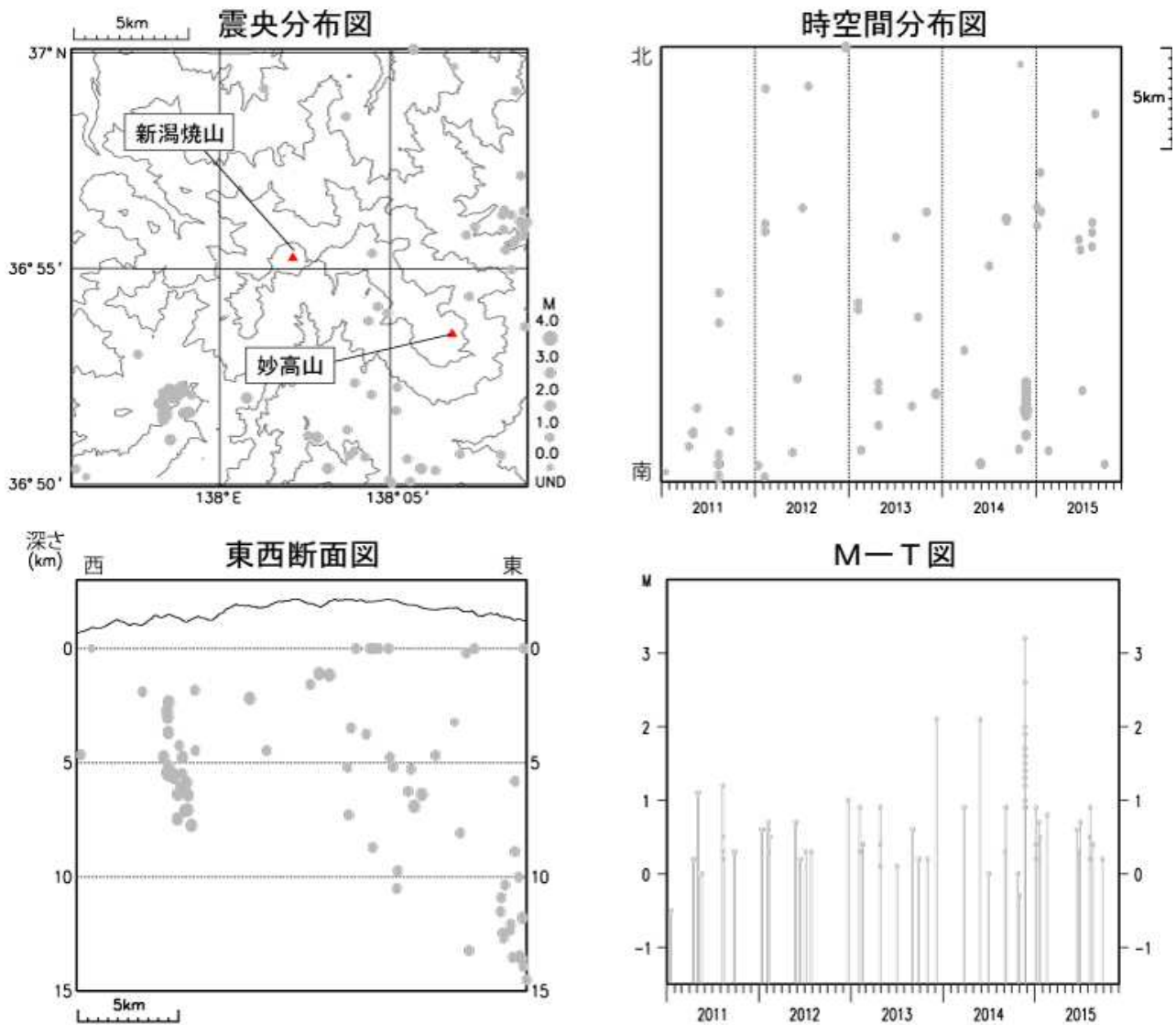
図4 新潟焼山 広域地震観測網による山体・周辺の地震活動（2011年1月1日～2015年11月30日）
