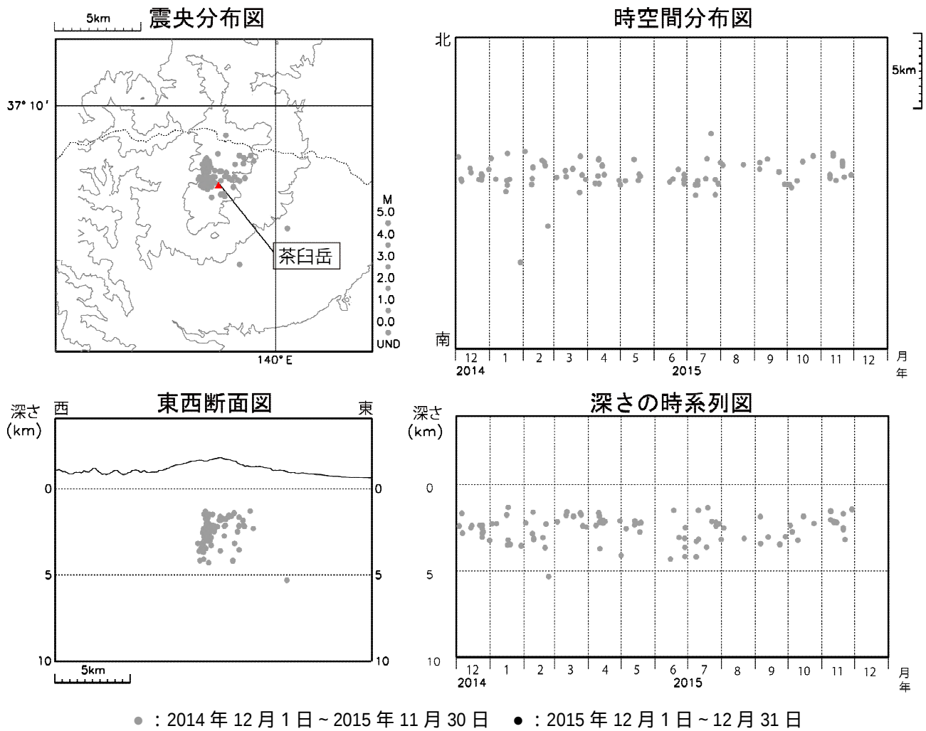
図3 那須岳 震源分布図（2014年12月1日～2015年12月31日） 今期間に震源が求まった地震はありませんでした。
