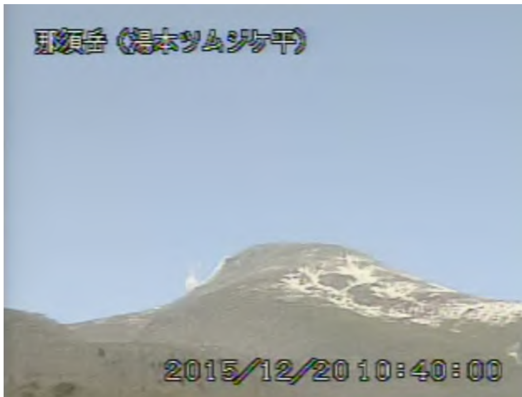
図 1 那須岳 茶臼岳の状況（12 月 20 日、那須湯本ツムジケ平遠望カメラによる）
