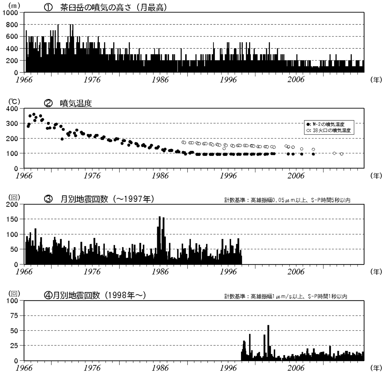
図2 那須岳 火山活動経過図（1966年1月～2015年12月）
