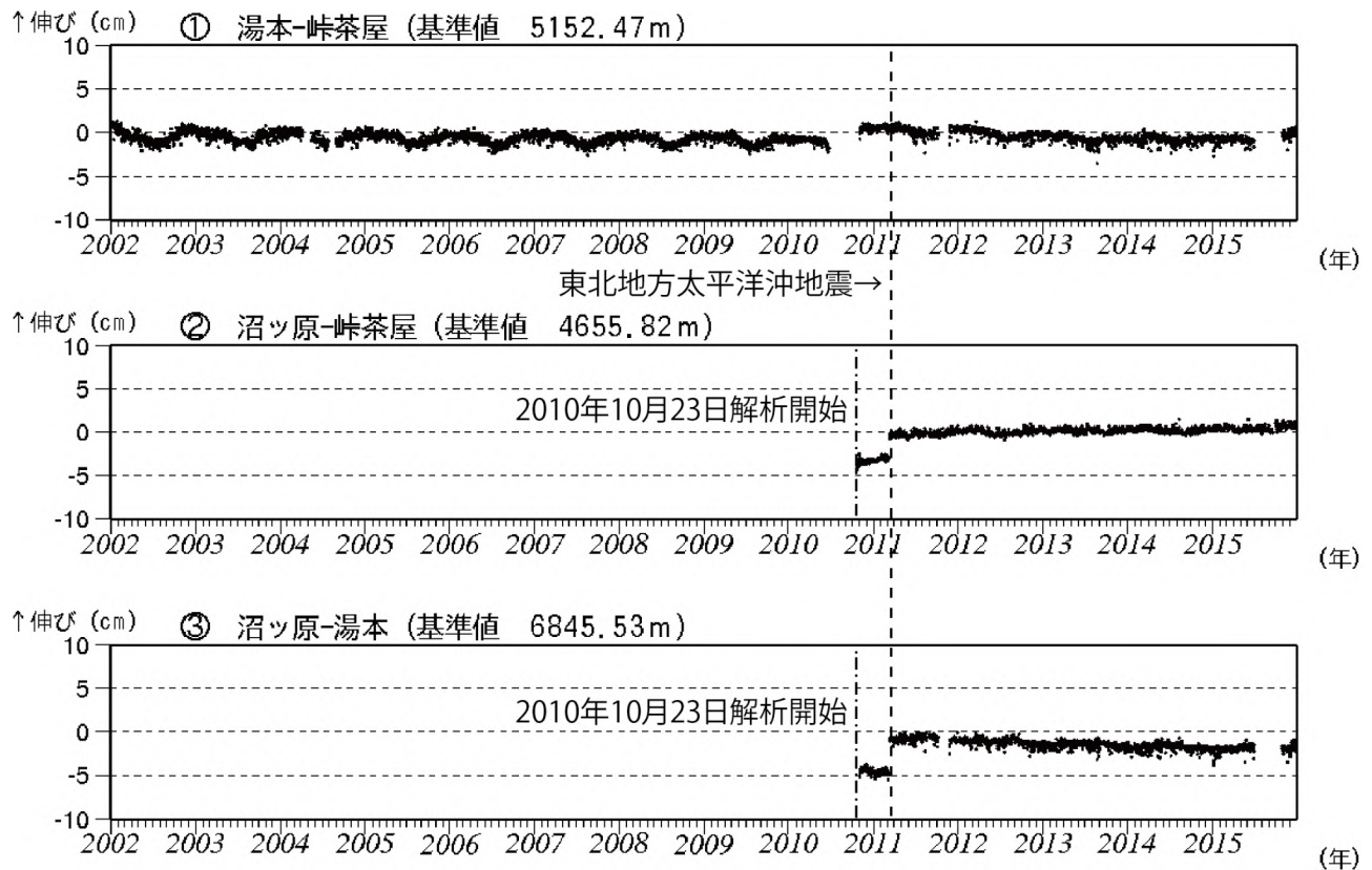
図4 那須岳 GNSS 連続観測による基線長変化（2002 年 1 月 1 日～2015 年 12 月 31 日） 2010 年 10 月以降のデータについては、電離層の影響を補正する等、解析方法を改良しています。 基線長変化にみられる冬季の伸びと夏季の縮みの傾向は季節変動による変化です。 2011 年 3 月 11 日に発生した東北地方太平洋沖地震の影響により、ステップ状の変化がみられます。 ～ は図 5 の GNSS 基線 ～ に対応しています。グラフの空白部分は欠測を示します。
