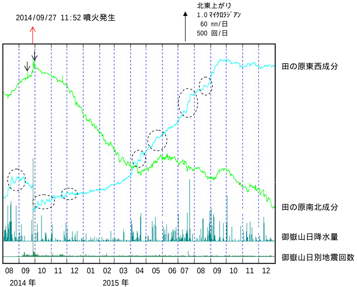
図5 御嶽山 田の原観測点（剣ヶ峰山頂の南東約 3 km）の傾斜変動 （2014 年 8 月 1 日～2015 年 12 月 31 日）
