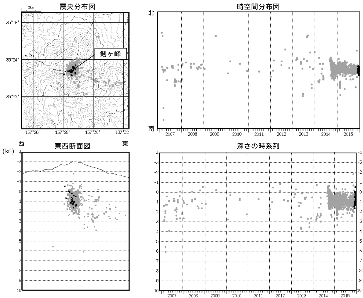
図 2 御嶽山 震源分布図（2006 年 12 月 1 日～2015 年 12 月 31 日）
