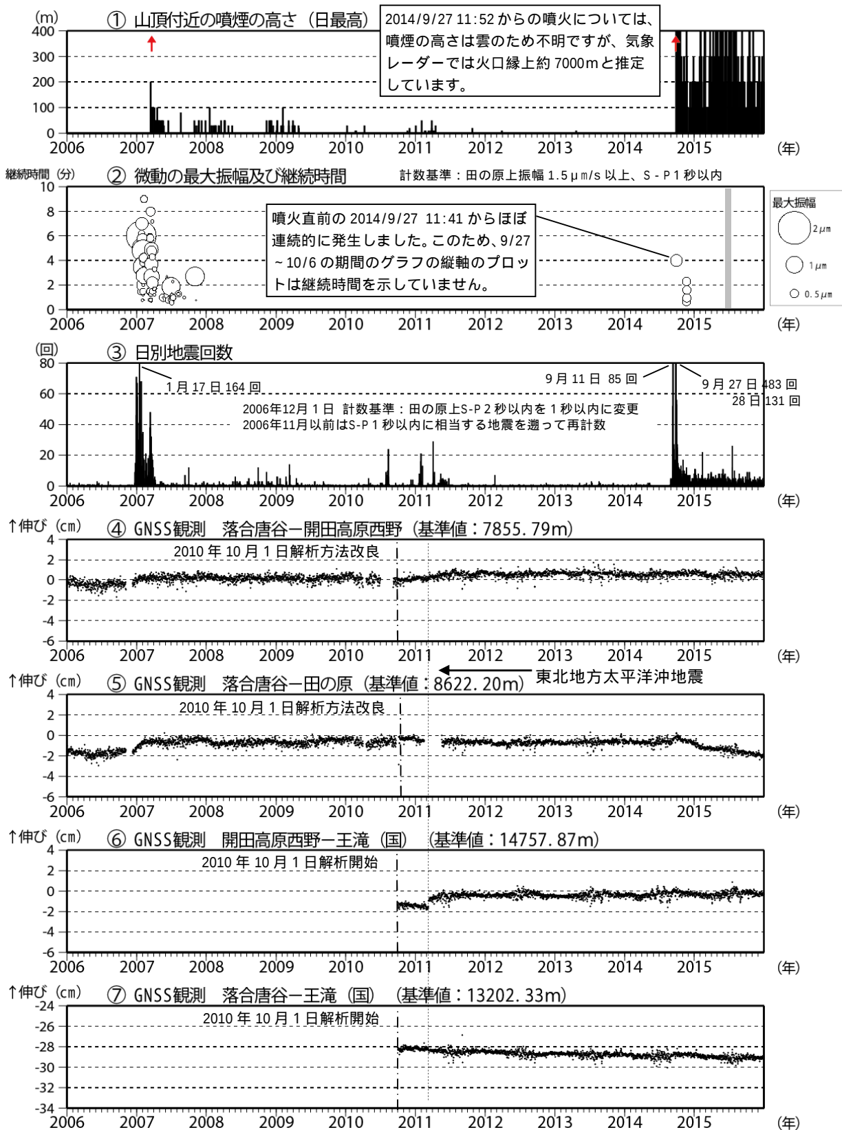
図4 御嶽山 長期間の火山活動経過図（2006年1月1日～2015年12月31日）
