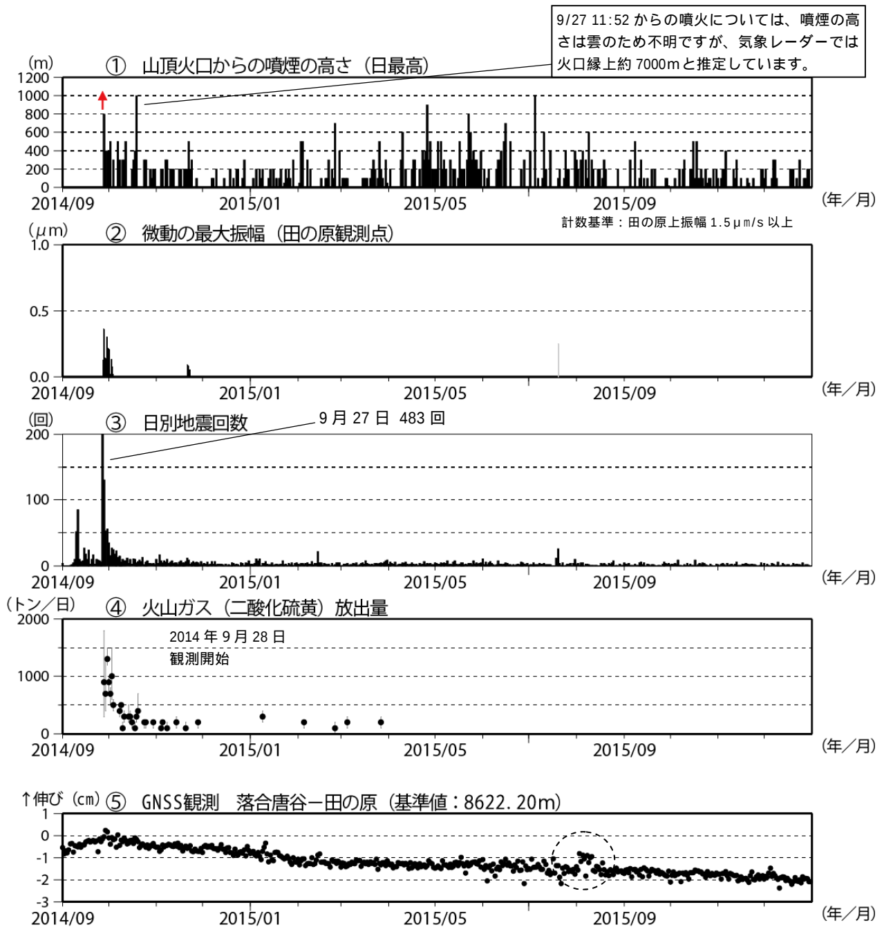
図 3 御嶽山 最近の火山活動経過図（2014 年 9 月 1 日～2015 年 12 月 31 日）
