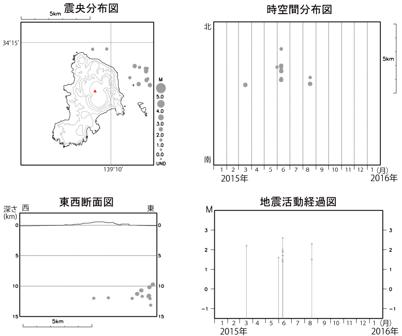
図4 神津島 広域地震観測網による山体・周辺の地震活動（2015 年 1 月 1 日～2016 年 1 月 31 日）
