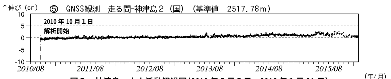
図 3 神津島 火山活動経過図(2010 年 8 月 2 日～2016 年 1 月 31 日)
