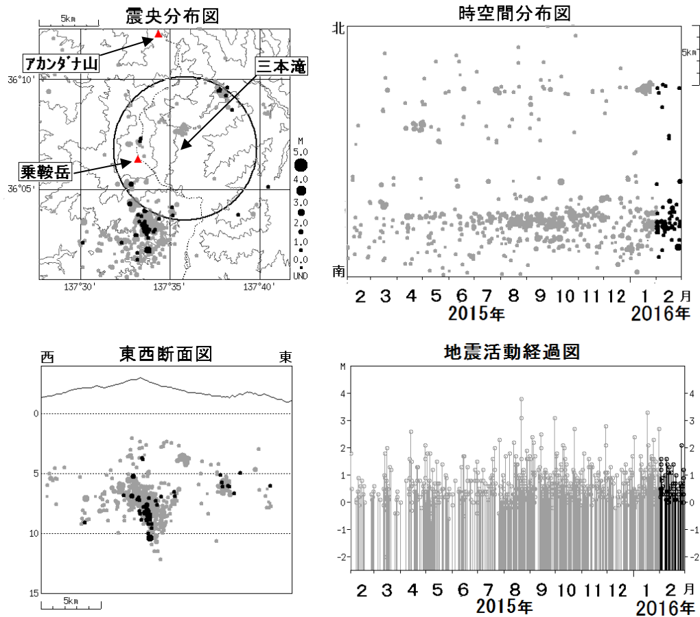
図3 乗鞍岳 広域地震観測網による山体・周辺の地震活動(2015年2月1日～2016年2月29日)
