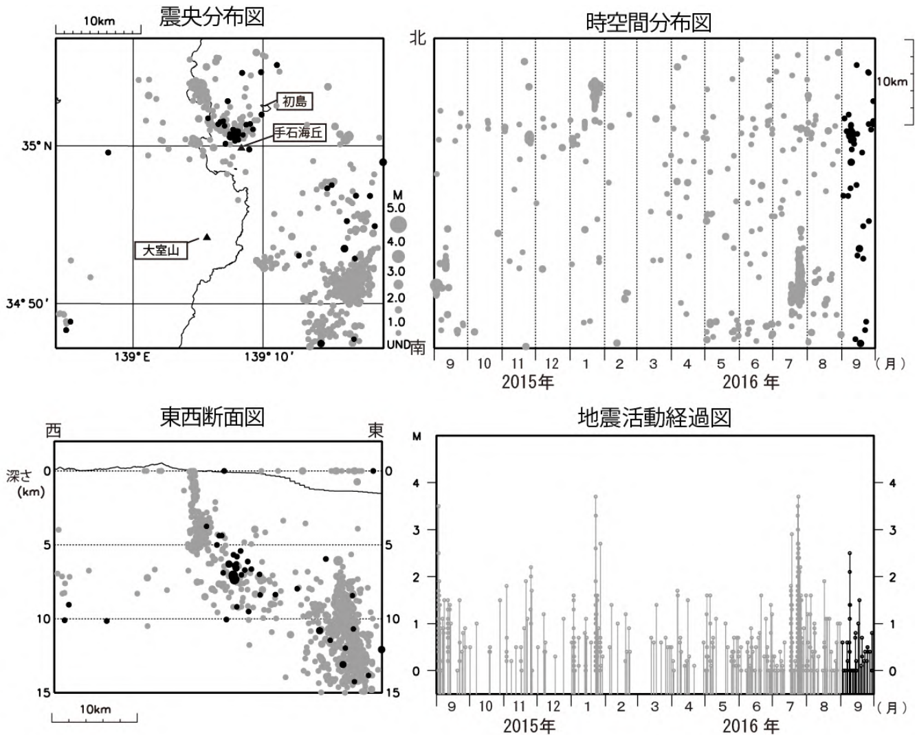
図2 伊豆東部火山群 広域地震観測網による震源分布図（2015年9月1日～2016年9月30日）
