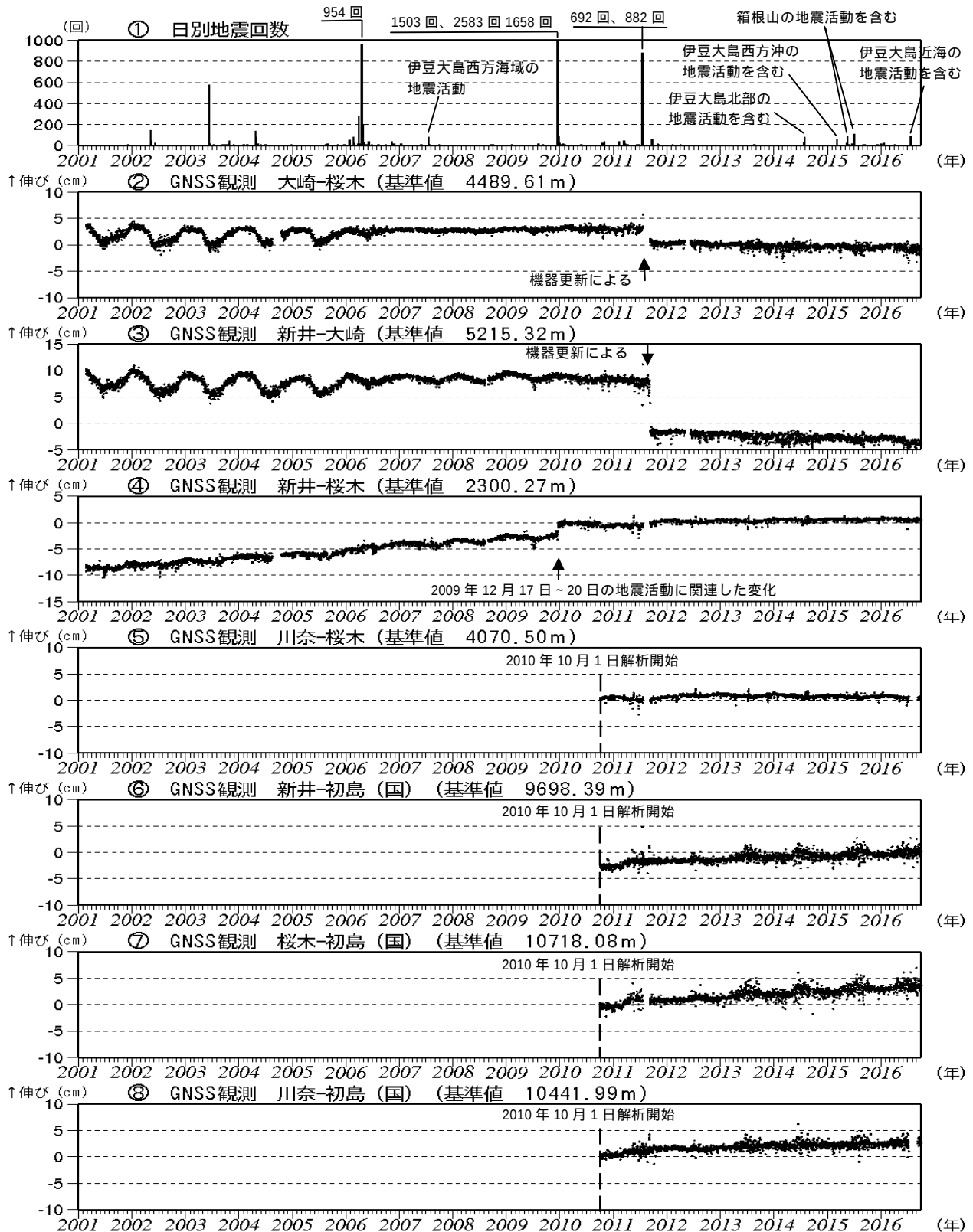
図3 伊豆東部火山群 火山活動経過図(2001年1月1日~2016年9月30日)
