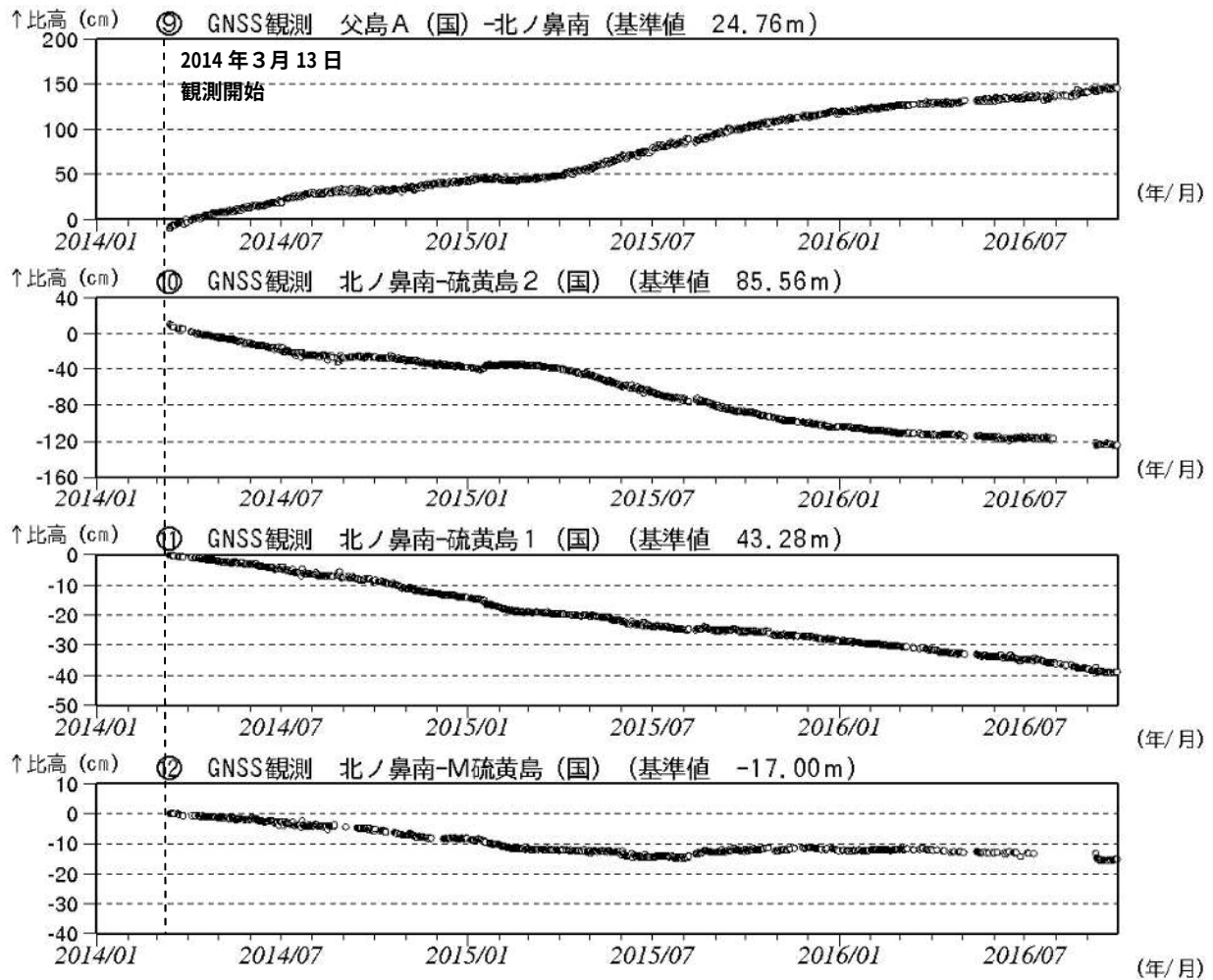
図7 硫黄島 GNSS 観測結果（2014年3月13日～2016年9月30日）（国）：国土地理院
