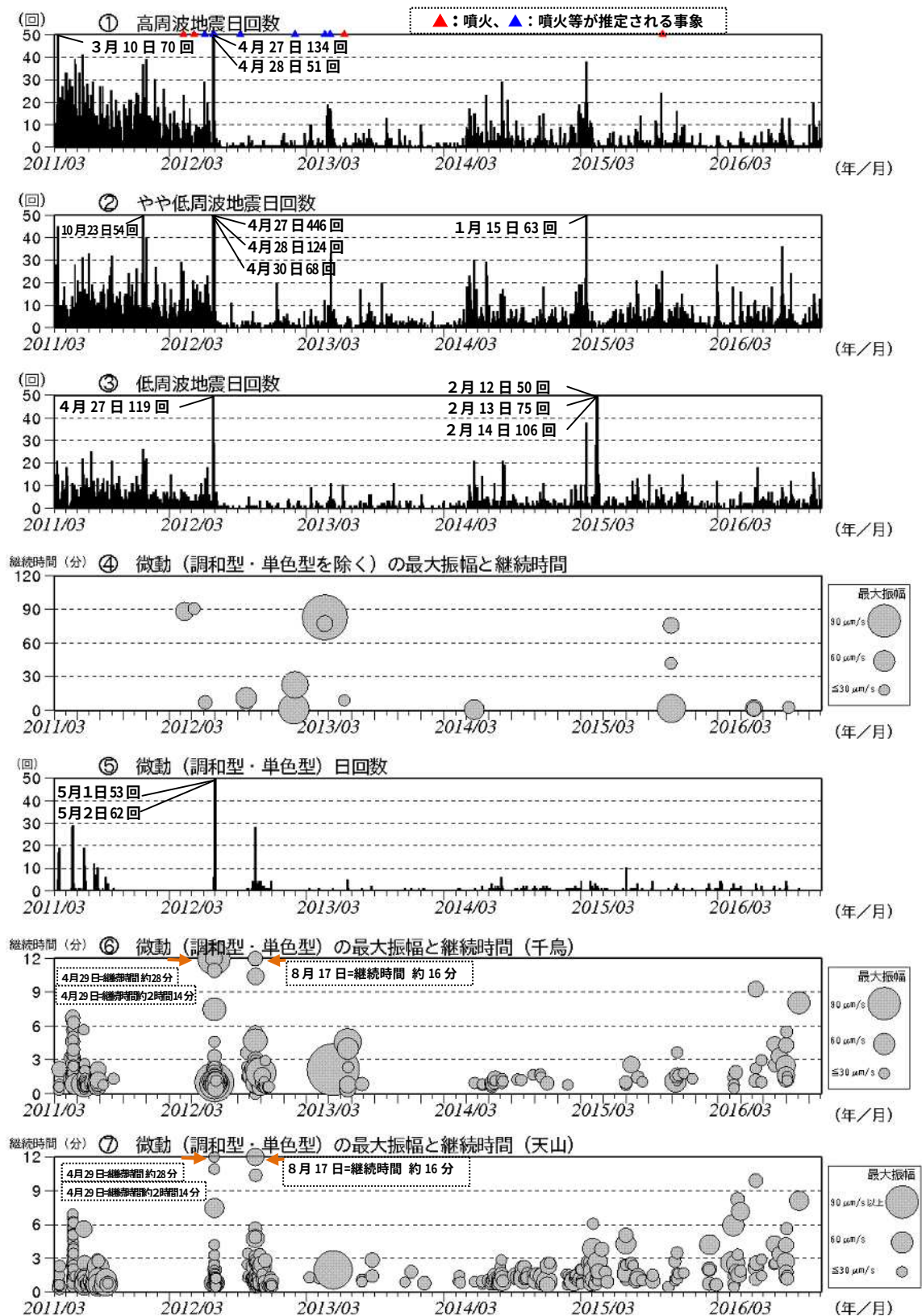
図5 硫黄島 火山活動経過図（2011年3月8日～2016年9月30日）
