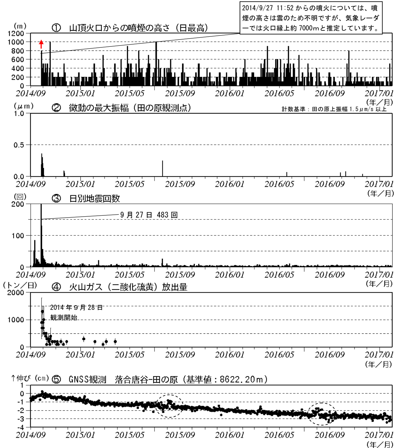
図 3 御嶽山 最近の火山活動経過図（2014 年 9 月 1 日～2017 年 1 月 31 日）
