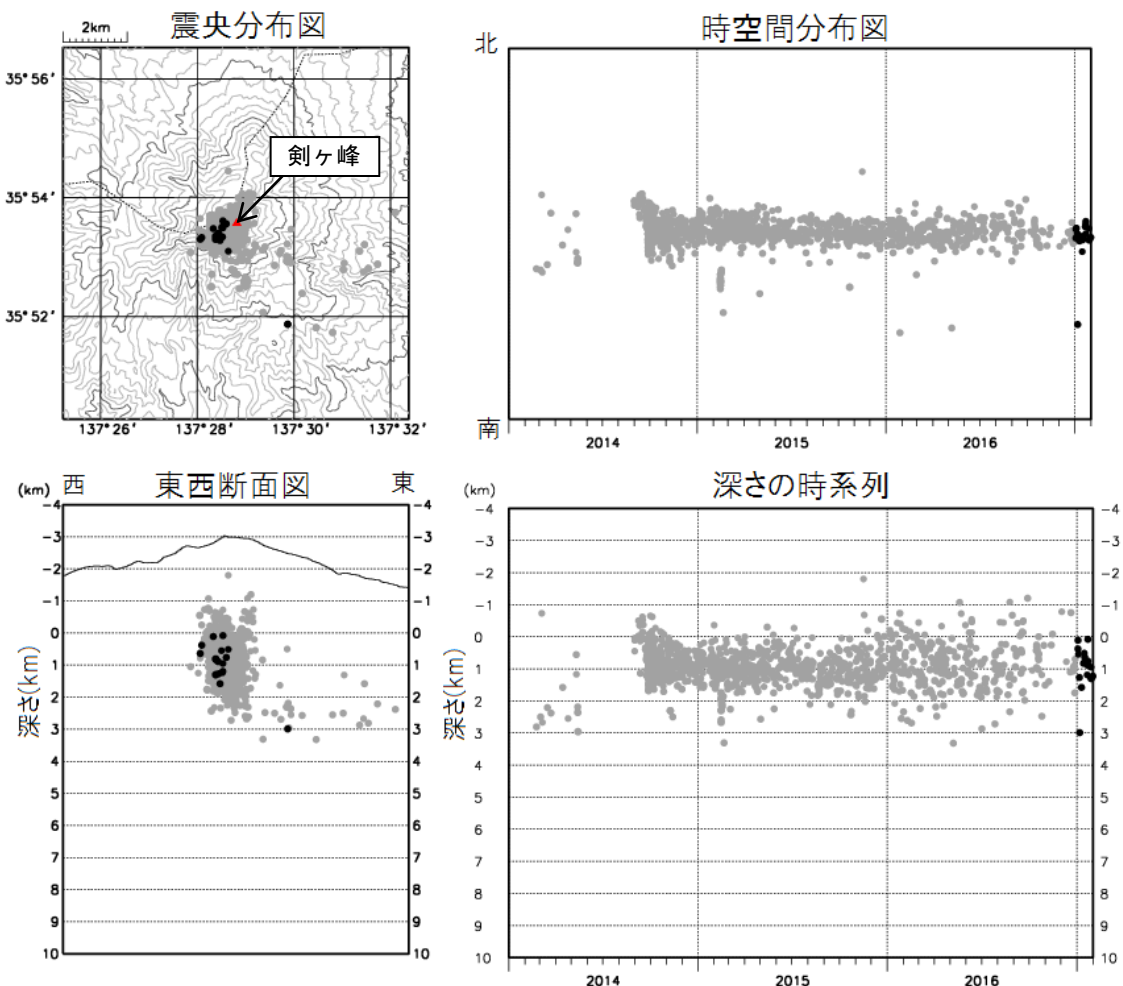
図 2 御嶽山 震源分布図（2014 年 1 月 1 日～2017 年 1 月 31 日）
