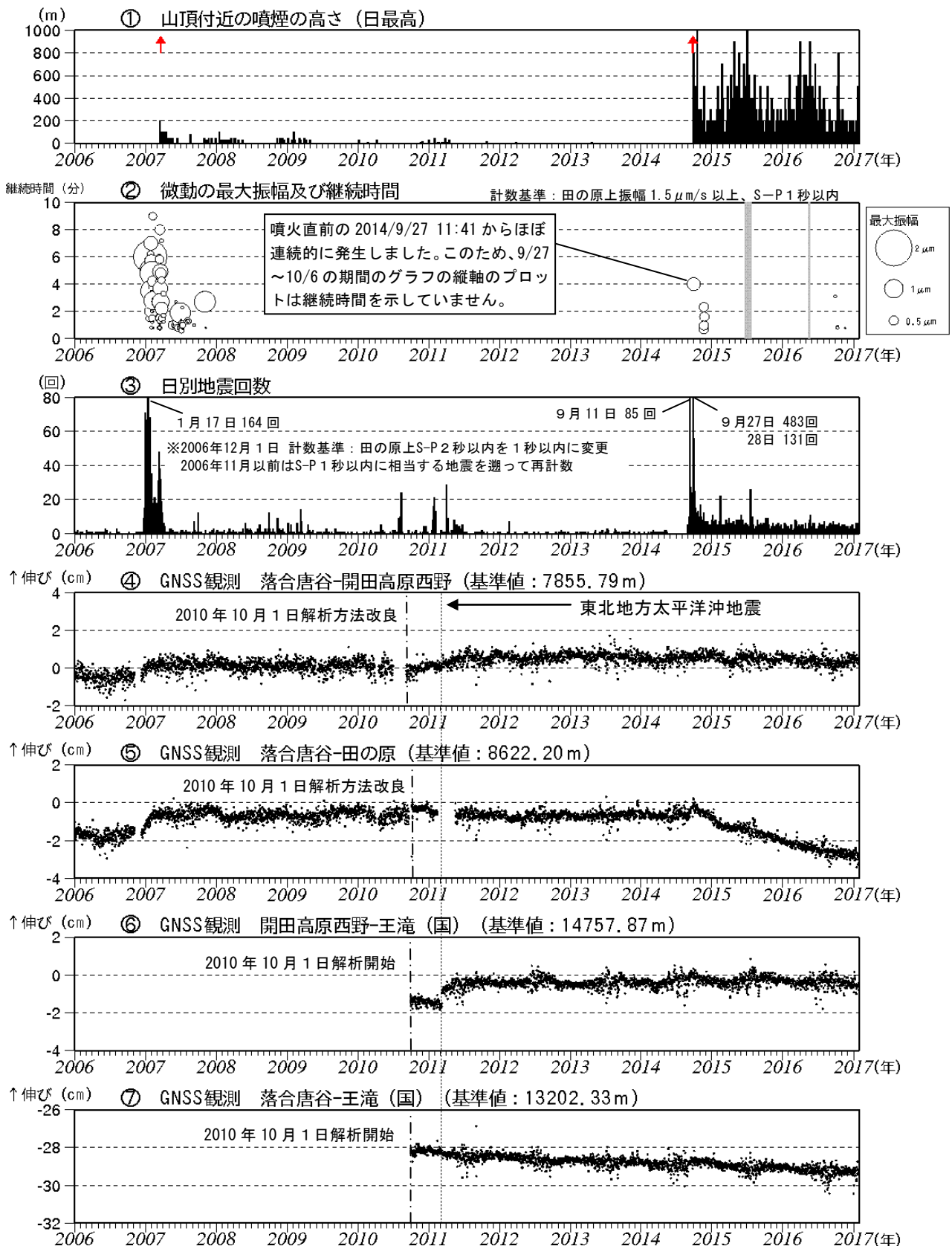
図4 御嶽山 長期間の火山活動経過図（2006 年 1 月 1 日～2017 年 1 月 31 日）
