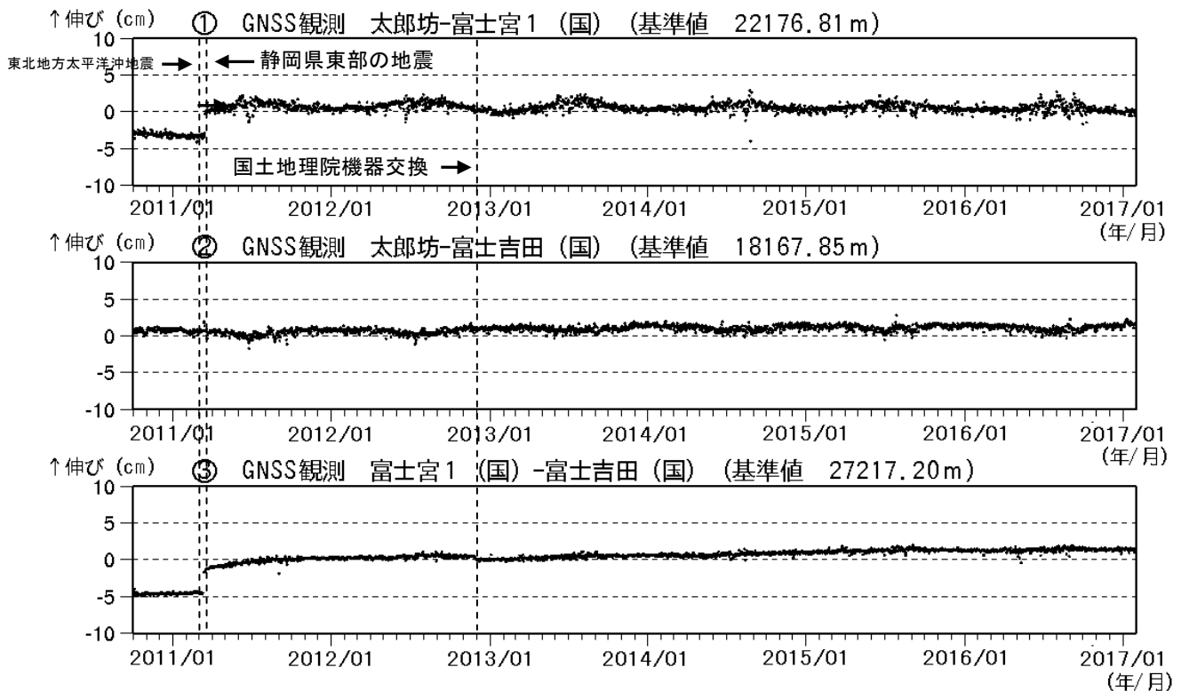
図4 富士山 GNSS 連続観測による基線長変化 (2010 年 10 月 1 日～2017 年 1 月 31 日) (国)：国土地理院
