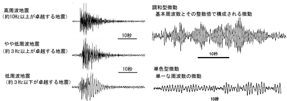
図3 硫黄島で見られる主な火山性地震、微動（調和型、単色型）の特徴と波形例
