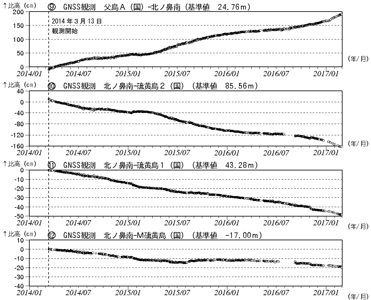
図6 硫黄島 GNSS 観測結果（2014年3月13日～2017年2月28日）（国）：国土地理院
