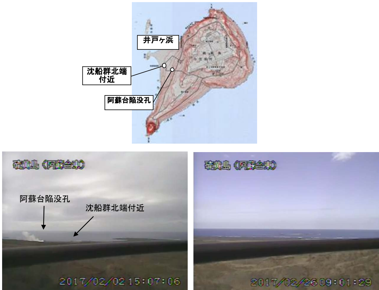
図2 硫黄島 海岸付近の噴気の状態、阿蘇台東監視カメラによる 上図：遠望観測対象地点 ※地形図は日本活火山総覧（第4版）から引用 左下図：阿蘇台陥没孔の噴気の状態（2月2日撮影） 右下図：井戸ヶ浜の状況（2月26日撮影）
