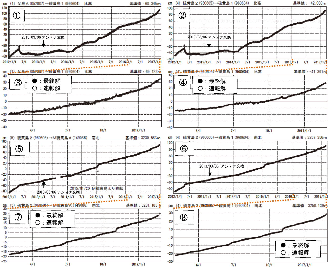
図 5 硫黄島 国土地理院による地殻変動観測結果 2)
