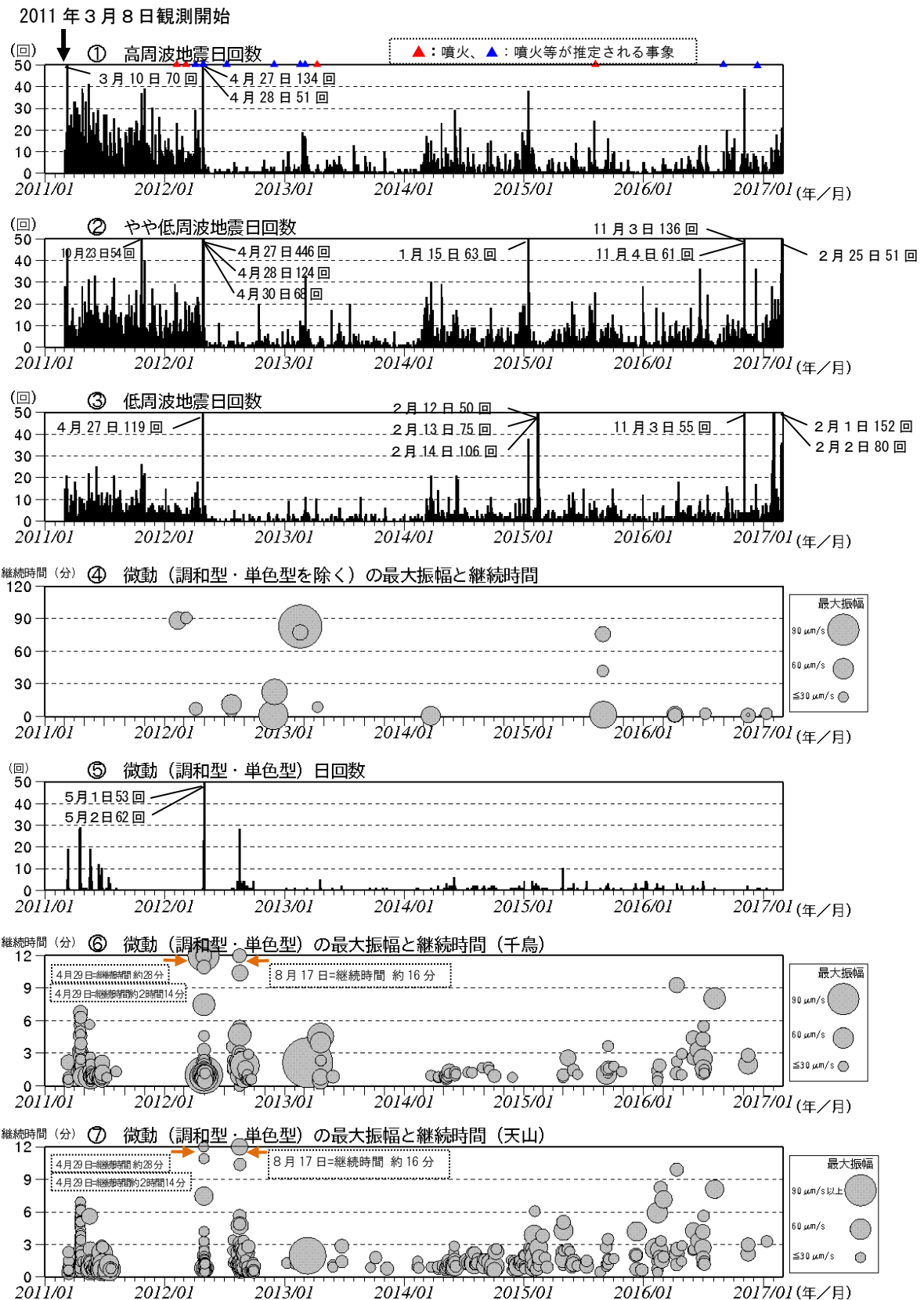
図4 硫黄島 火山活動経過図（2011 年 3 月 1 日～2017 年 2 月 28 日）
