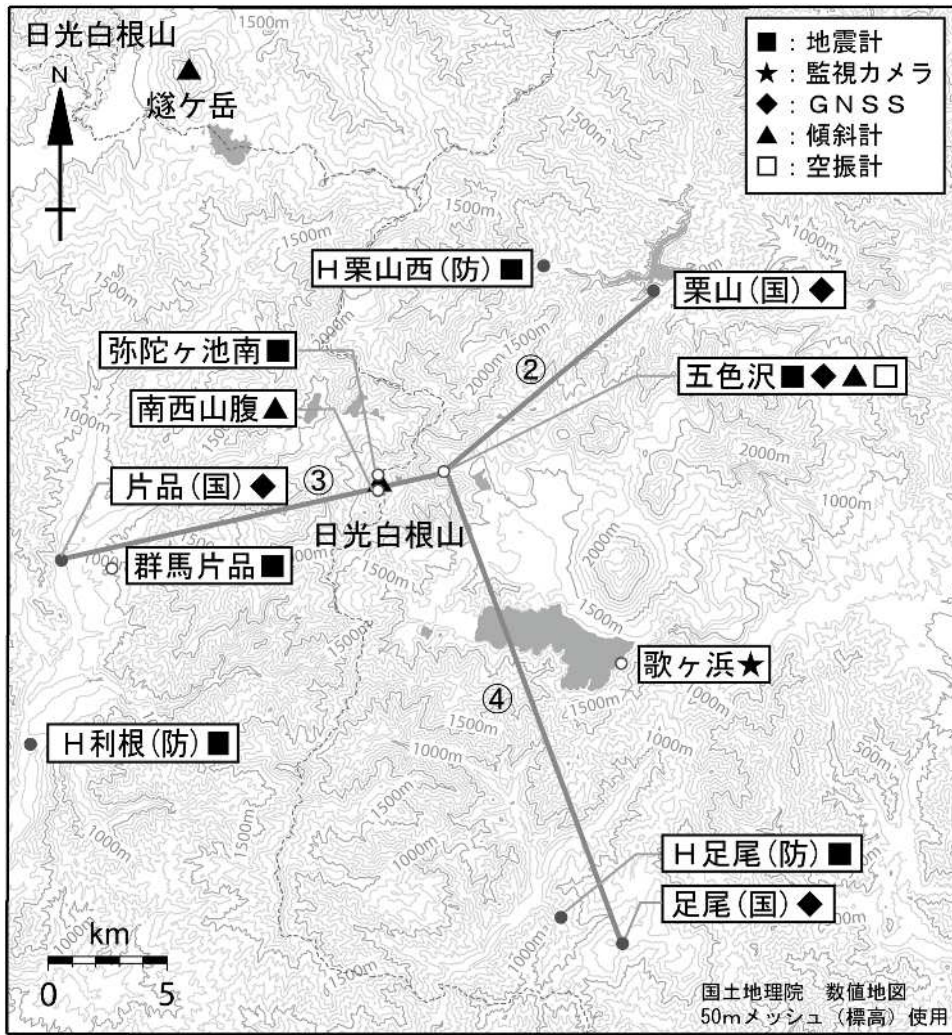
図 5 日光白根山 観測点配置
