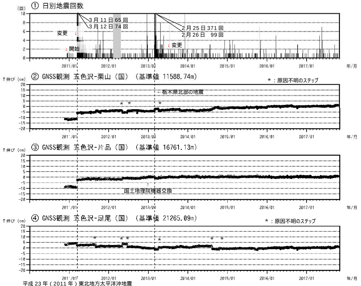
図 3 日光白根山 火山活動経過図（2010 年 11 月 20 日～2017 年 10 月 31 日）
