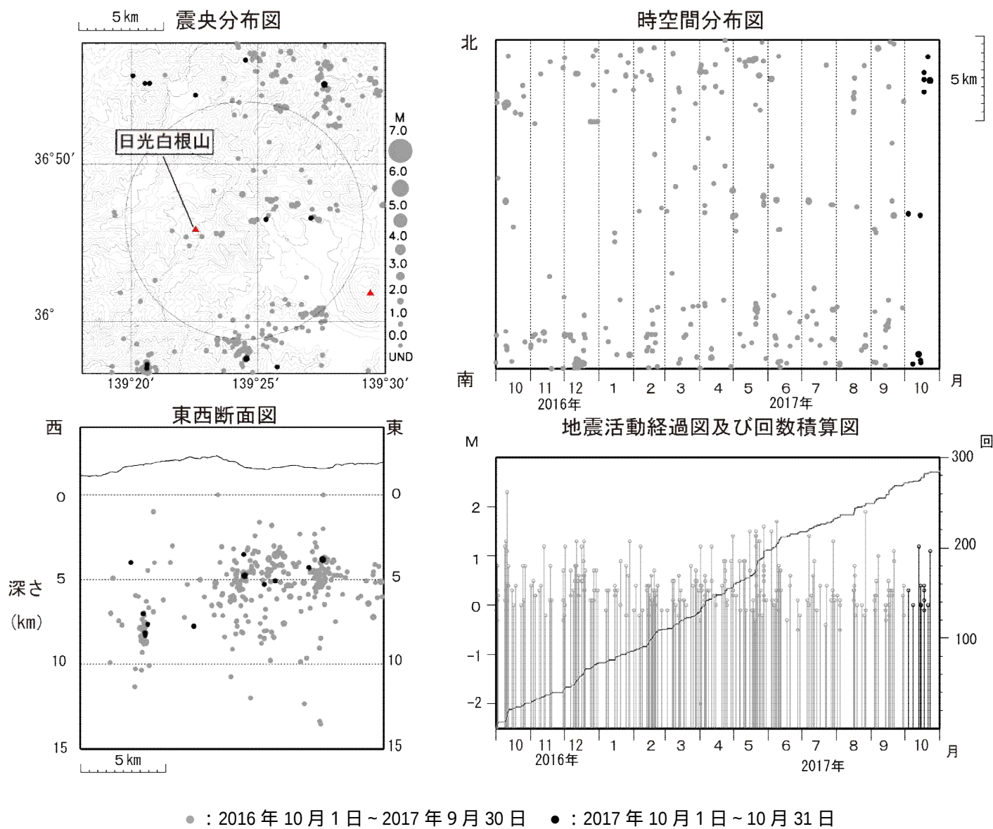
図 4 日光白根山 広域地震観測網による山体・周辺の地震活動(2016 年 10 月 1 日 ~ 2017 年 10 月 31 日) 震央分布図中の円は図 2 - の計数対象地震（五色沢で S - P 時間 1 秒以内）のおよその範囲を示しています。 震源の深さは全て海面以下として震源決定しています。 図中の震源要素は一部暫定値が含まれており、後日変更することがあります。
