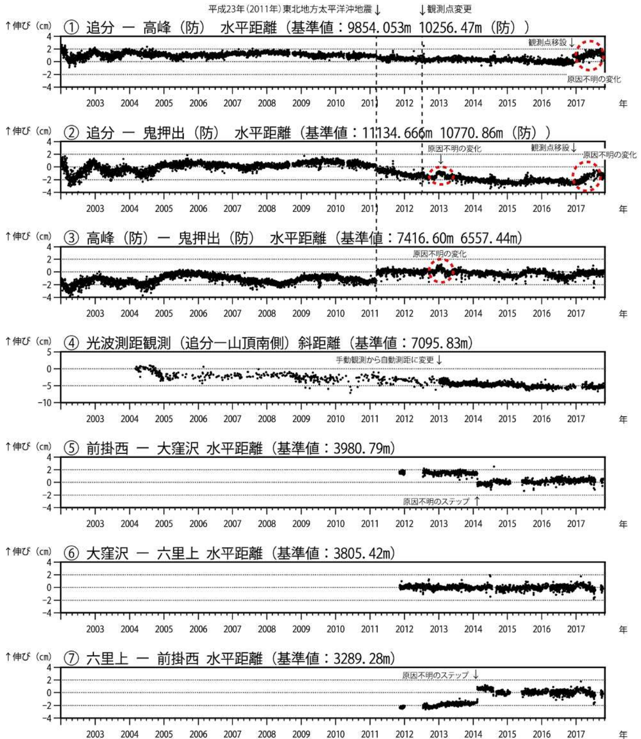
図6 浅間山 GNSS 連続観測及び光波測距観測の結果(2002 年 1 月 1 日 ~ 2017 年 10 月 31 日)
