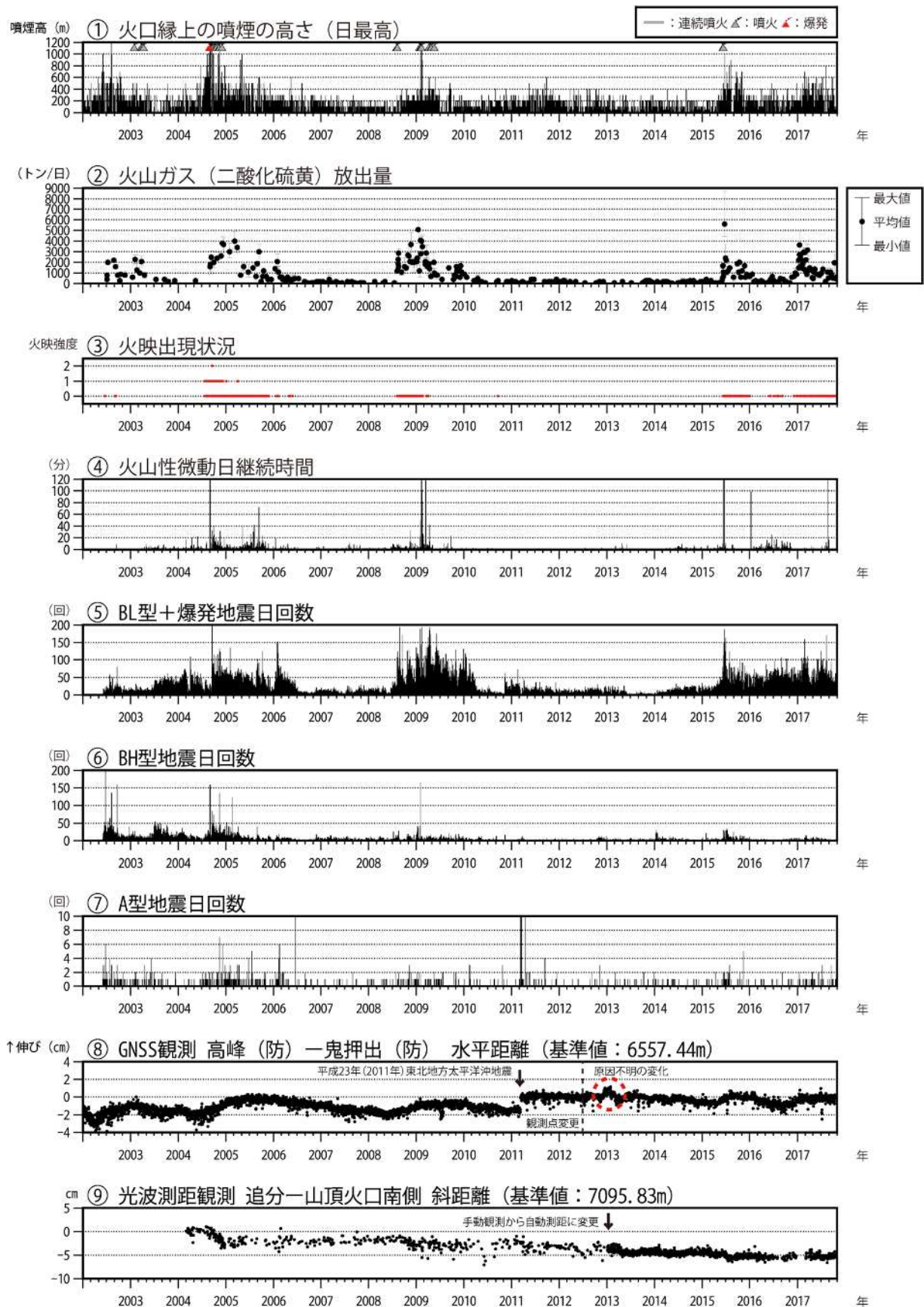
図 3 浅間山 火山活動経過図 (2002 年 1 月 1 日 ~ 2017 年 10 月 31 日)
