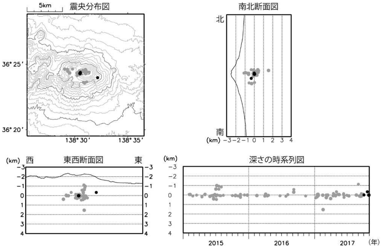
図 5 浅間山 震源分布図（2015 年 1 月 1 日～2017 年 10 月 31 日）
