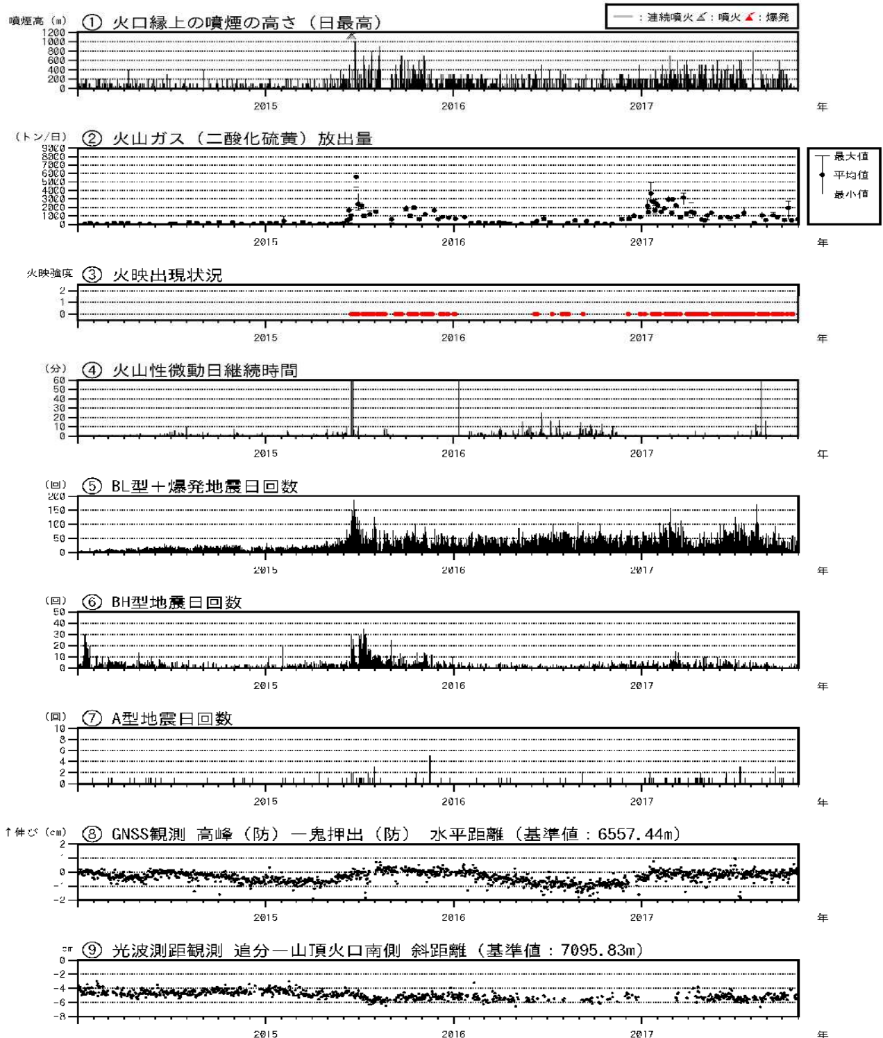
図4 浅間山 最近の火山活動経過図（2014年1月1日～2017年10月31日）
