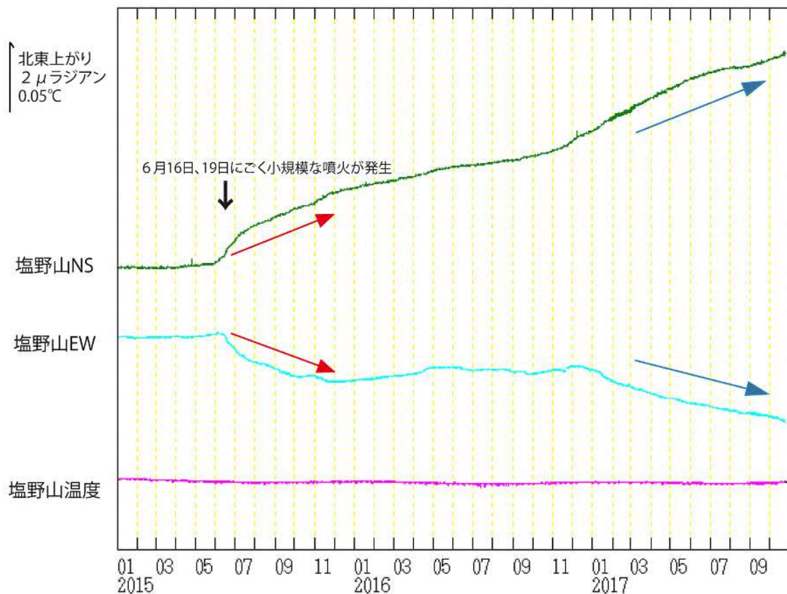
図8 浅間山 塩野山観測点における傾斜データ（2015年1月1日～2017年10月31日）
