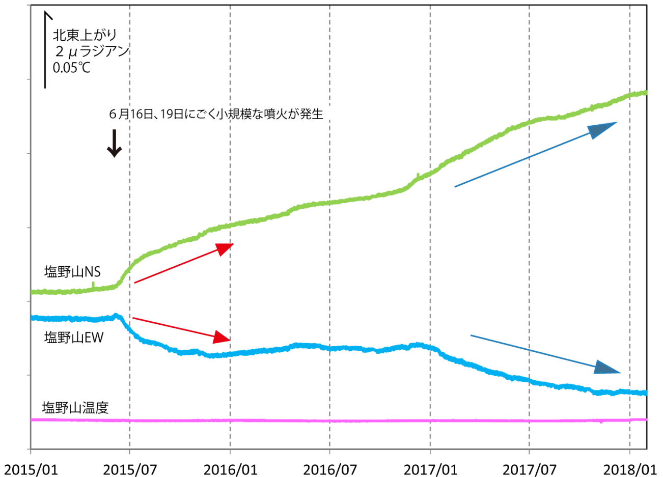
図8 浅間山 塩野山観測点における傾斜データ（2015年1月1日～2018年1月31日）
