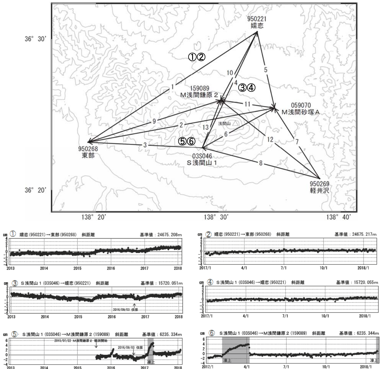
図9 浅間山 国土地理院による地殻変動観測結果 5)
