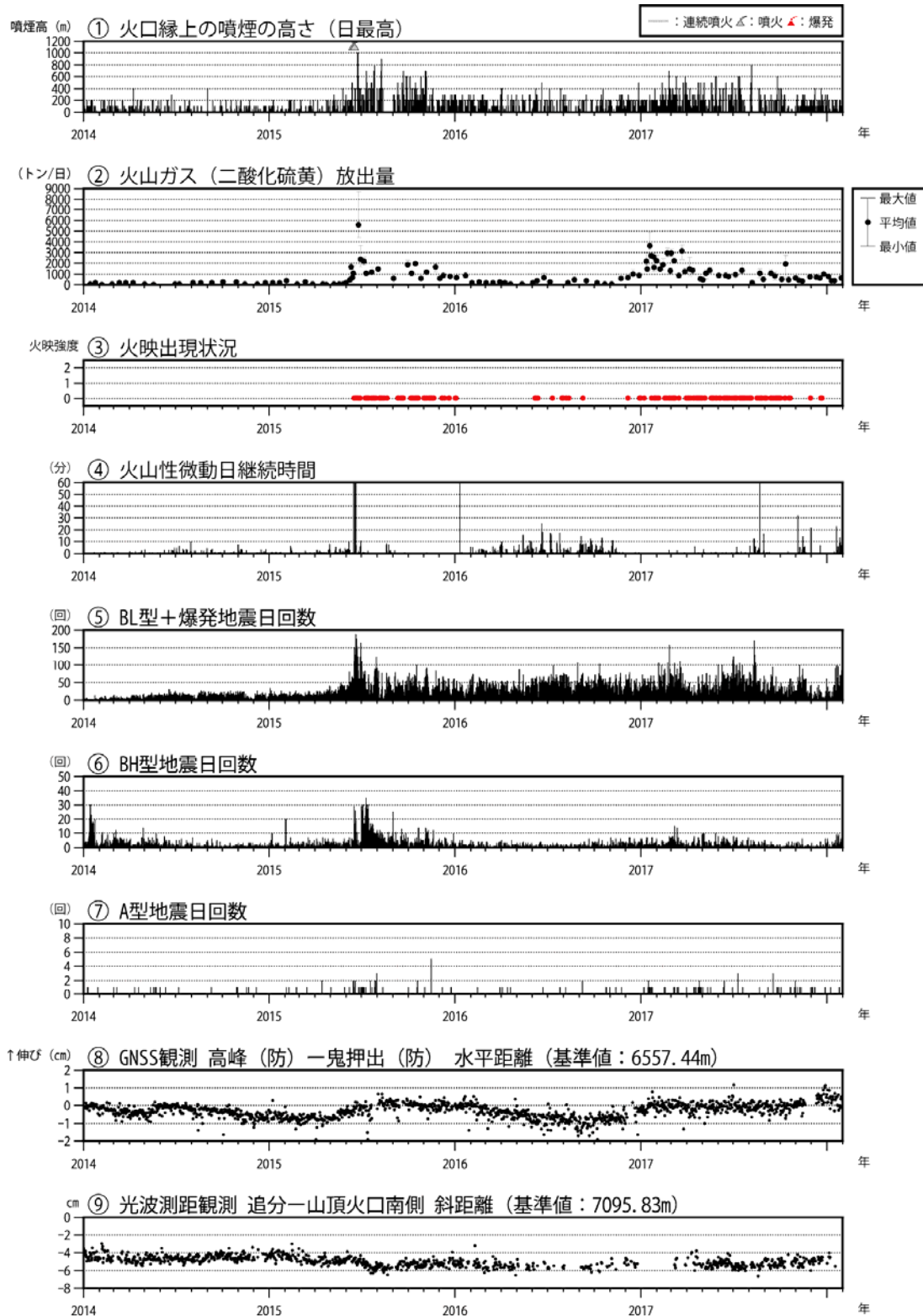
図 4 浅間山 最近の火山活動経過図（2014 年 1 月 1 日～2018 年 1 月 31 日）
