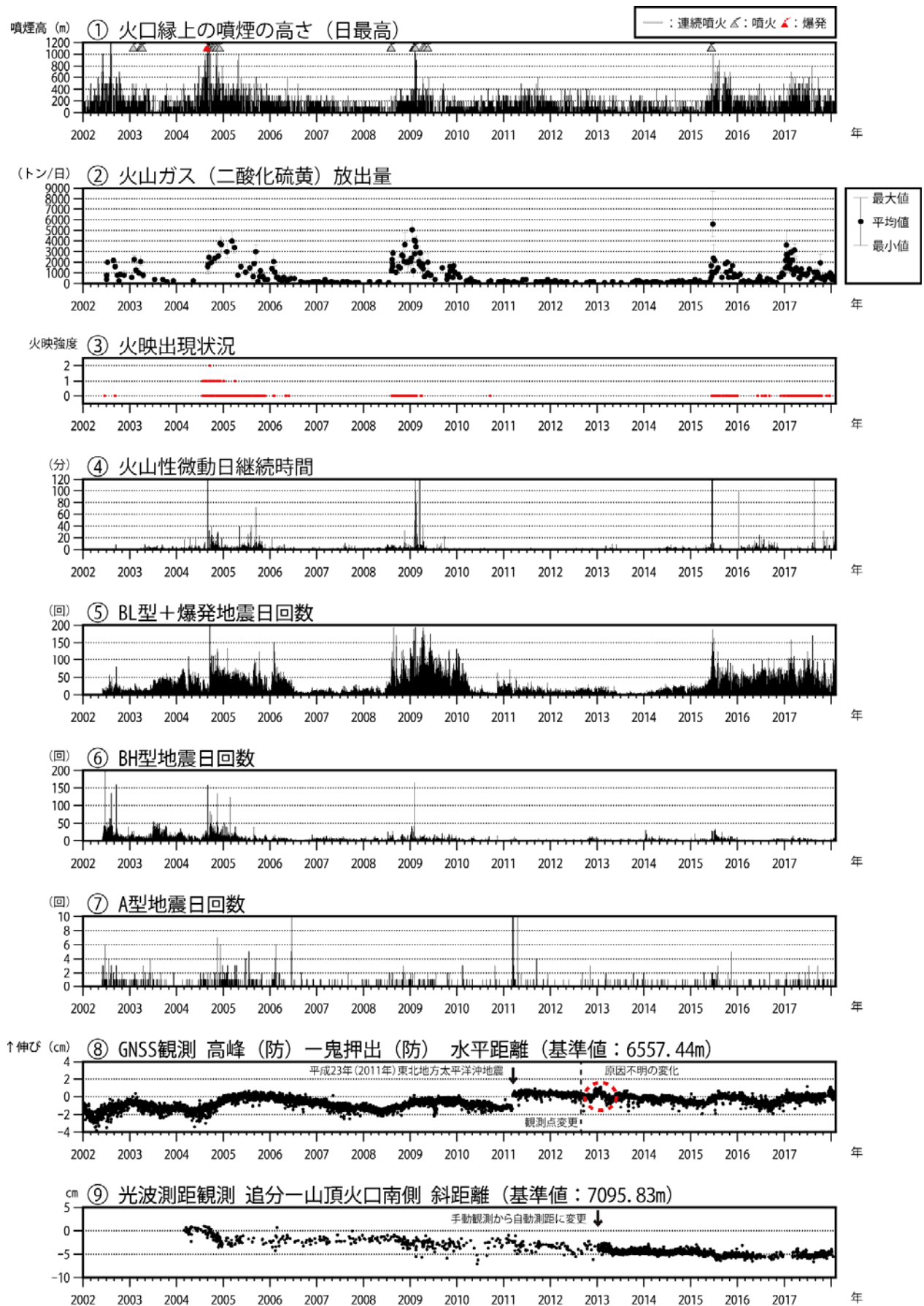
図3 浅間山 火山活動経過図（2002年1月1日～2018年1月31日）
