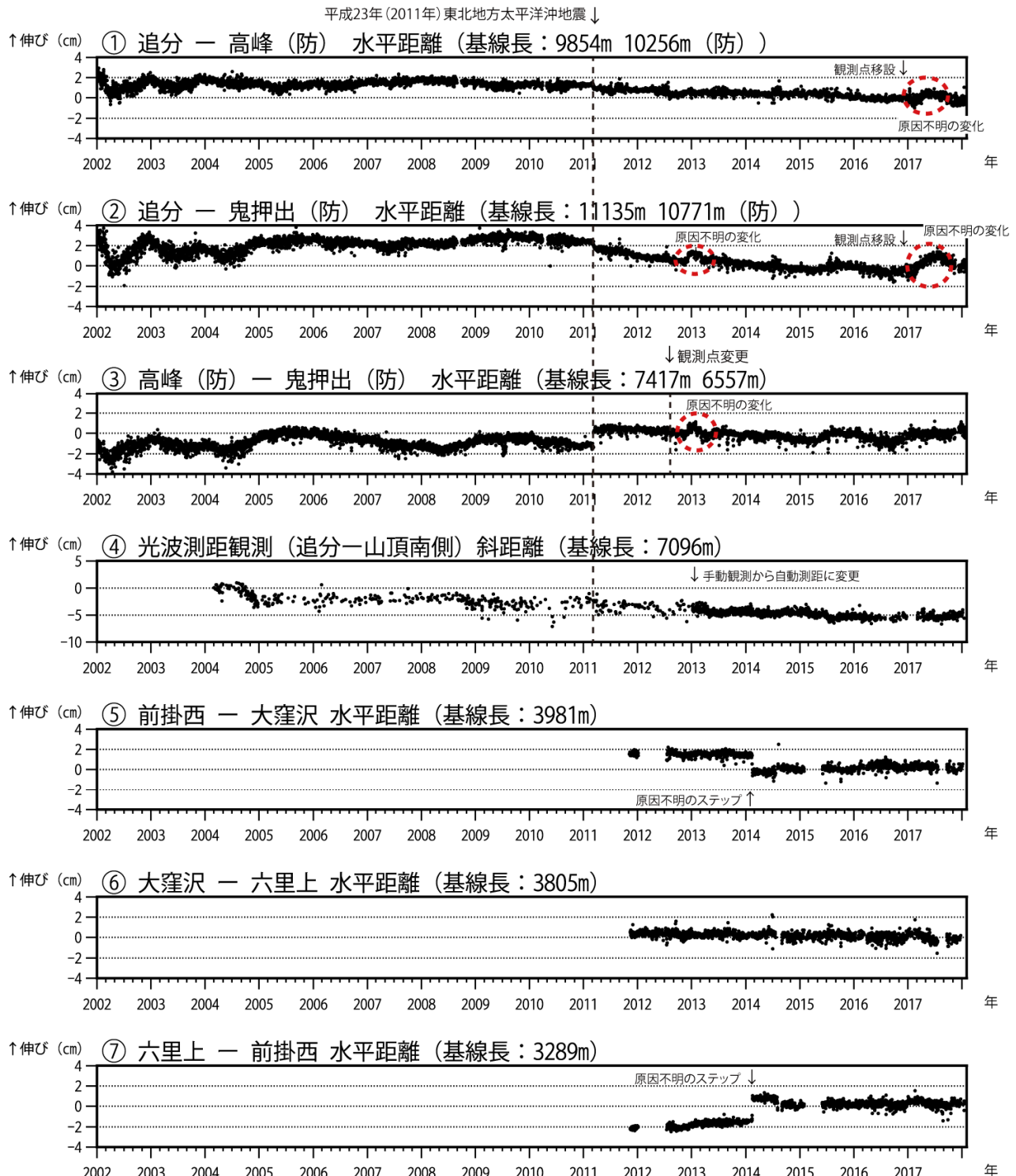
図 6 浅間山 GNSS 連続観測及び光波測距観測の結果 (2002 年 1 月 1 日～2018 年 1 月 31 日)
