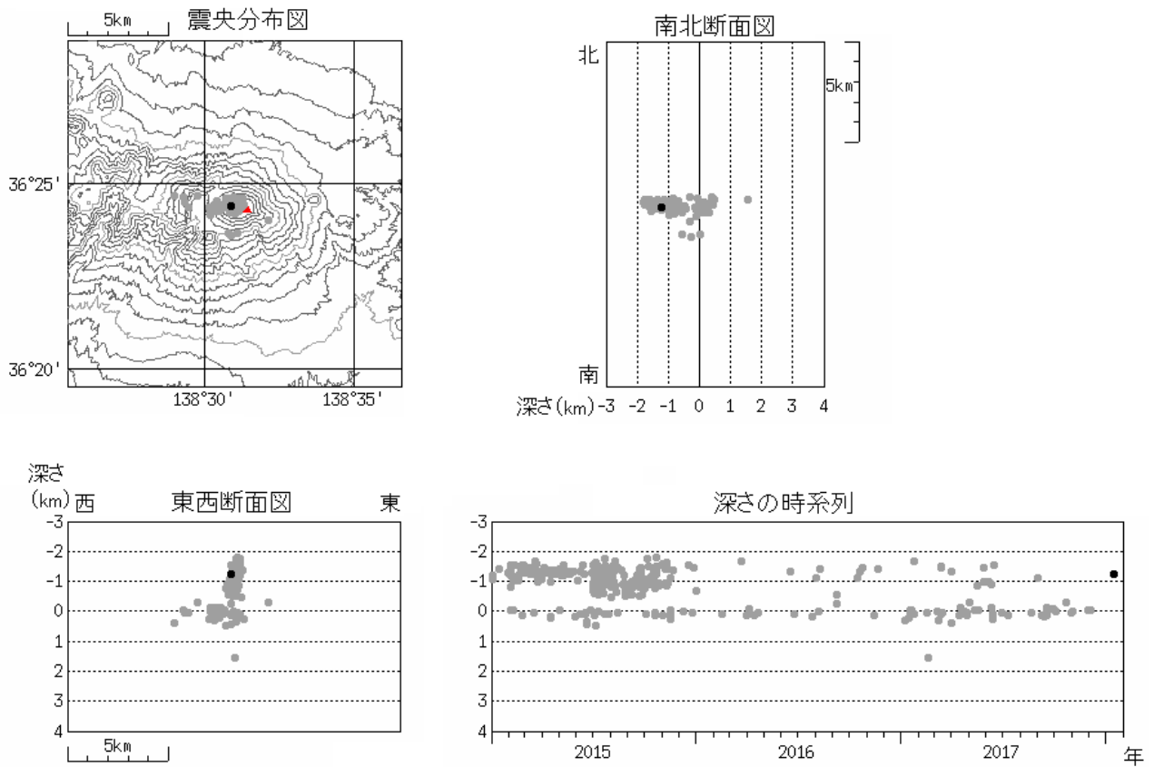
図5 浅間山 震源分布図（2015 年 1 月 1 日～2018 年 1 月 31 日）
