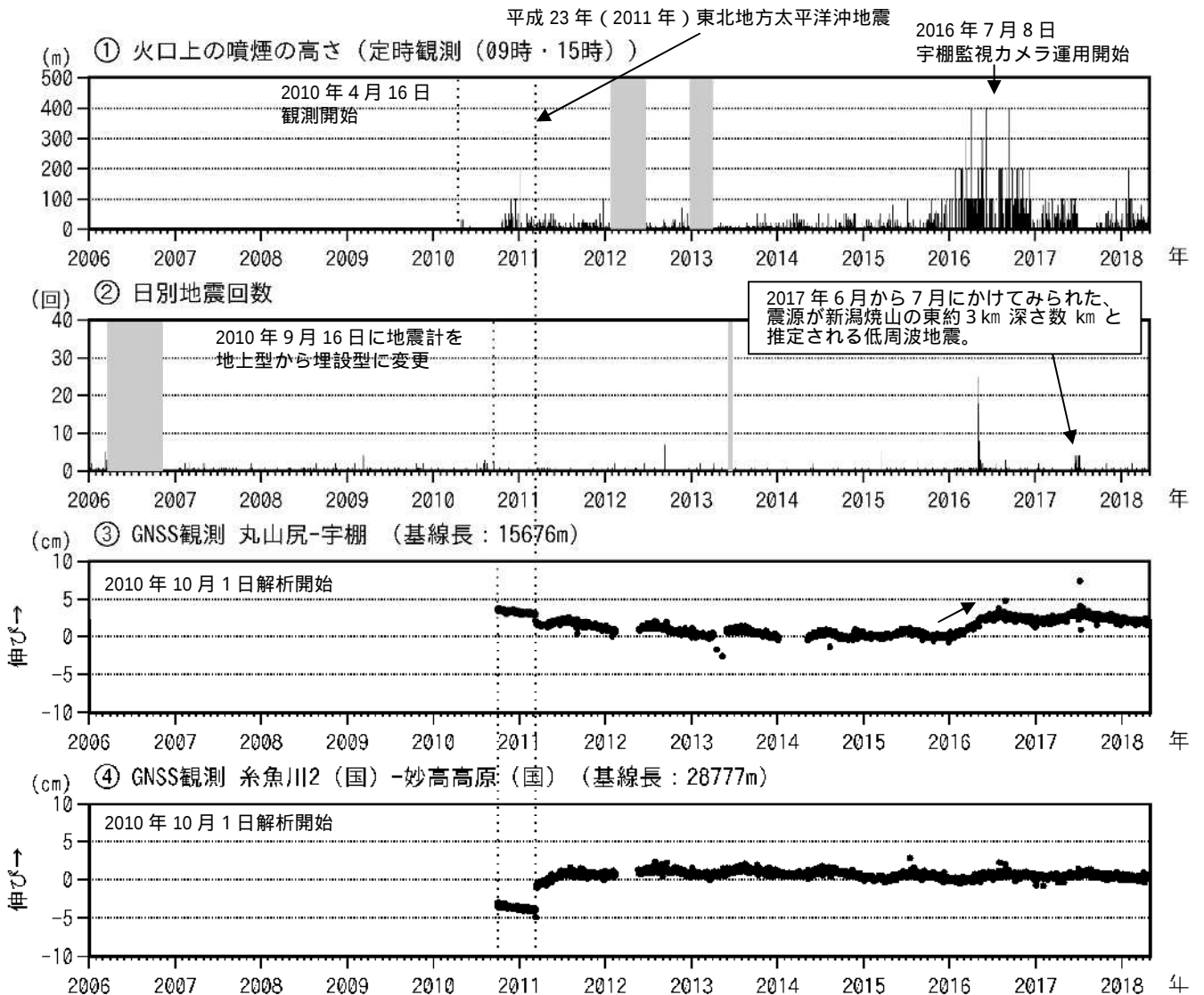
図 3 新潟焼山 火山活動経過図（2006 年 1 月 1 日～2018 年 4 月 30 日）
