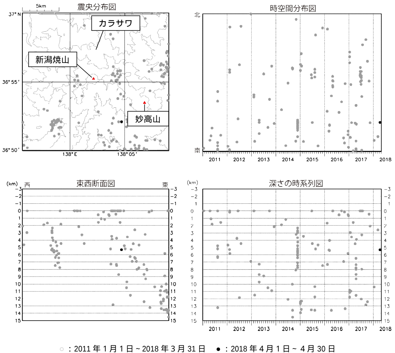
図 8 新潟焼山 広域地震観測網による山体・周辺の地震活動（2011 年 1 月 1 日～2018 年 4 月 30 日）
