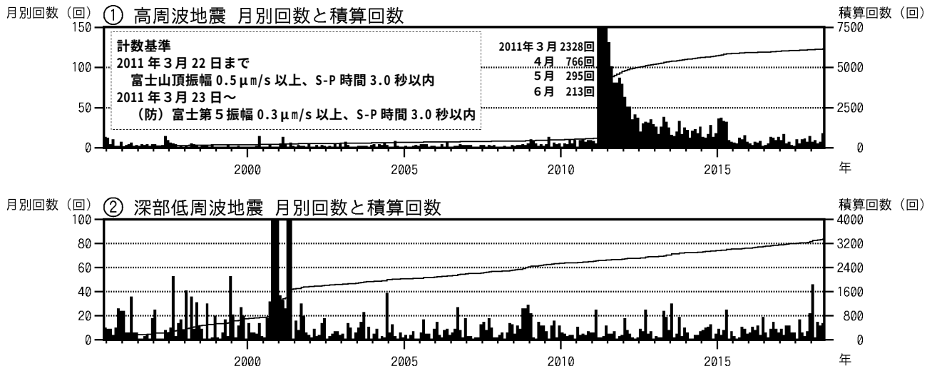
図 2 富士山 月別地震回数 (1995 年 6 月 1 日～2018 年 5 月 31 日)
