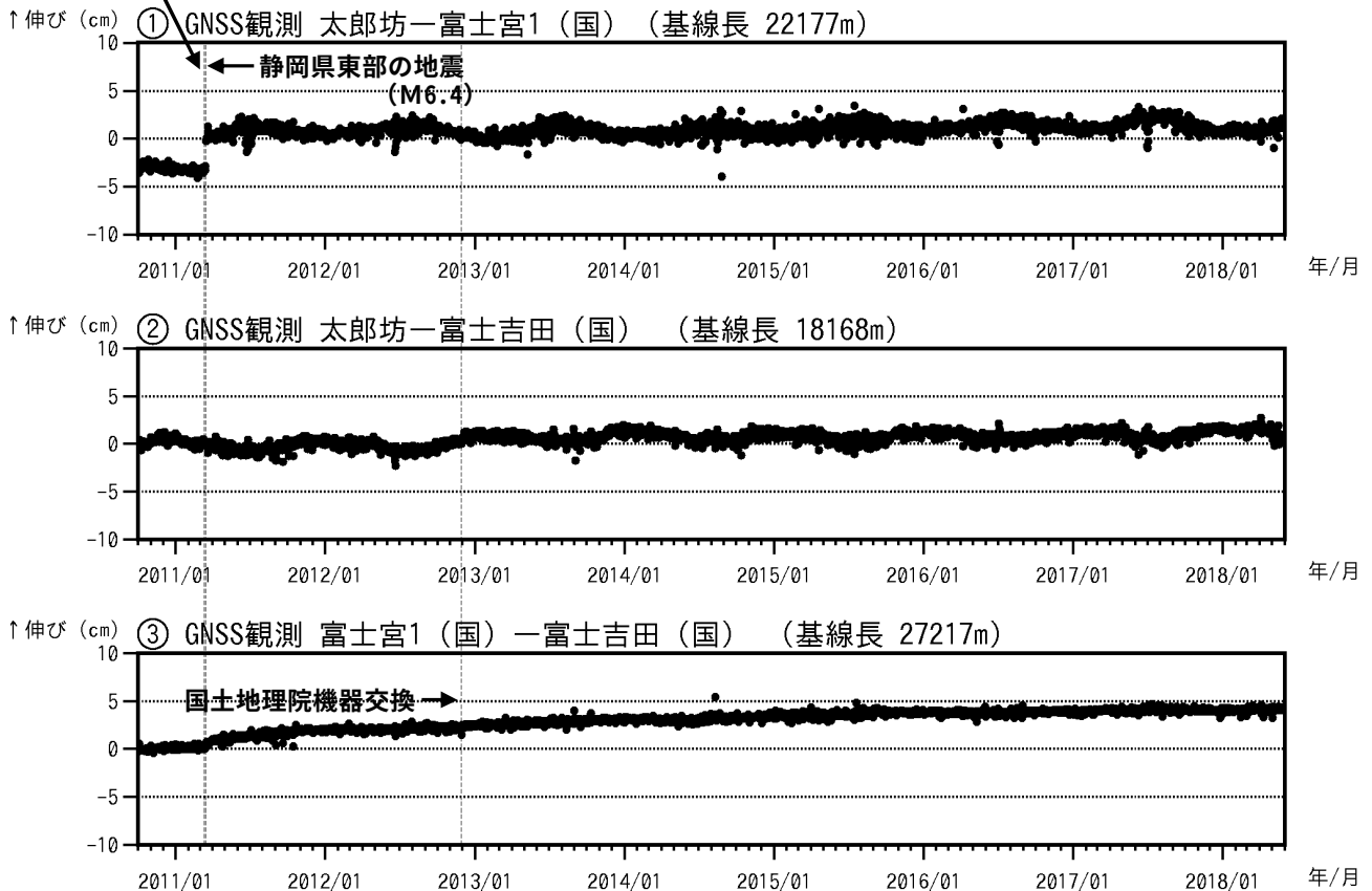
図 4 富士山 GNSS 連続観測による基線長変化 (2010 年 10 月 1 日～2018 年 5 月 31 日)
