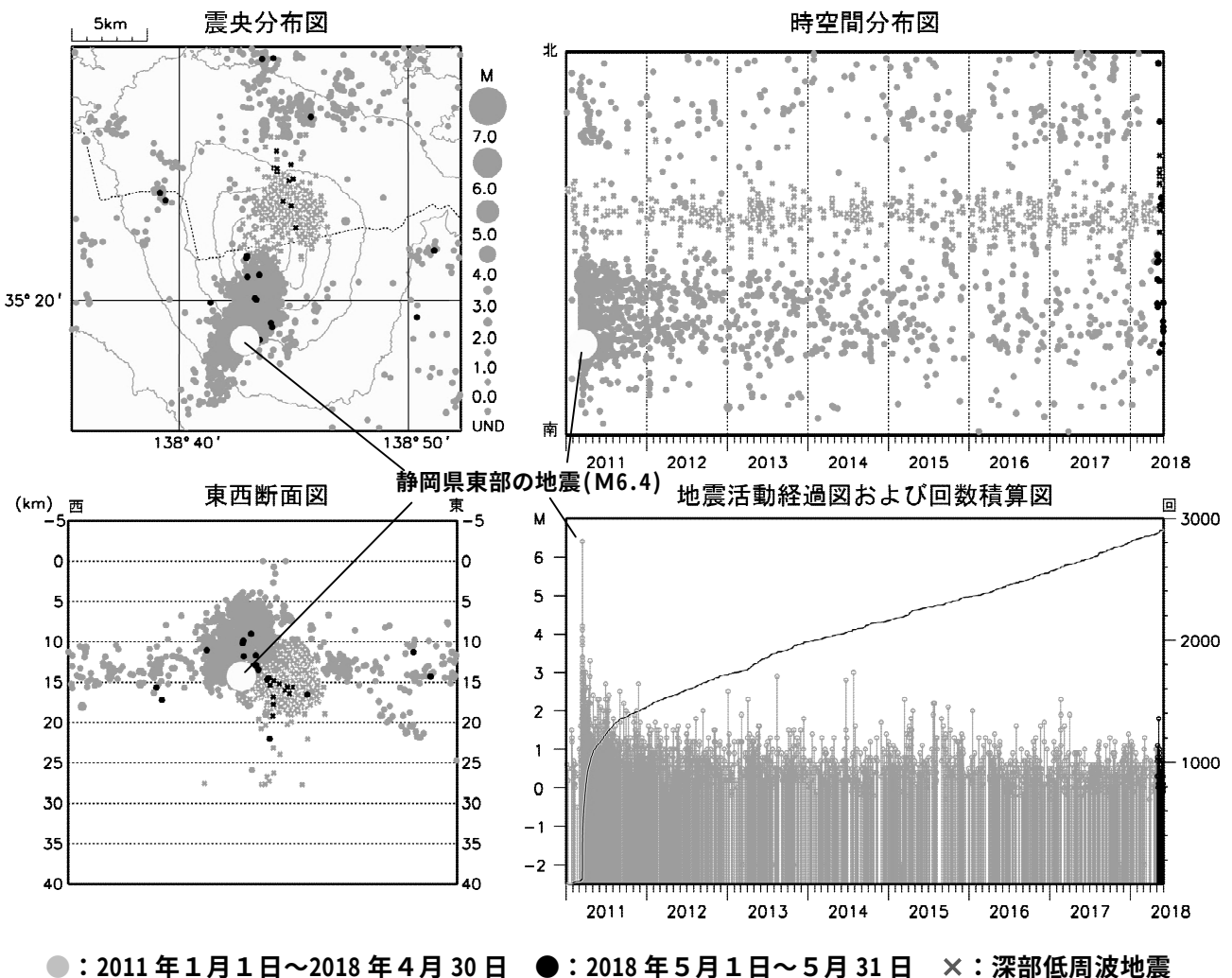
図 3 富士山 広域地震観測網による山体・周辺の地震活動 (2011 年 1 月 1 日～2018 年 5 月 31 日)
