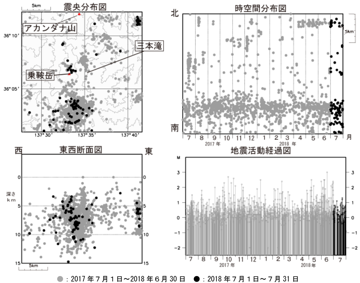
図 3 乗鞍岳 広域地震観測網による山体・周辺の地震活動(2017 年 7 月 1 日～2018 年 7 月 31 日)
