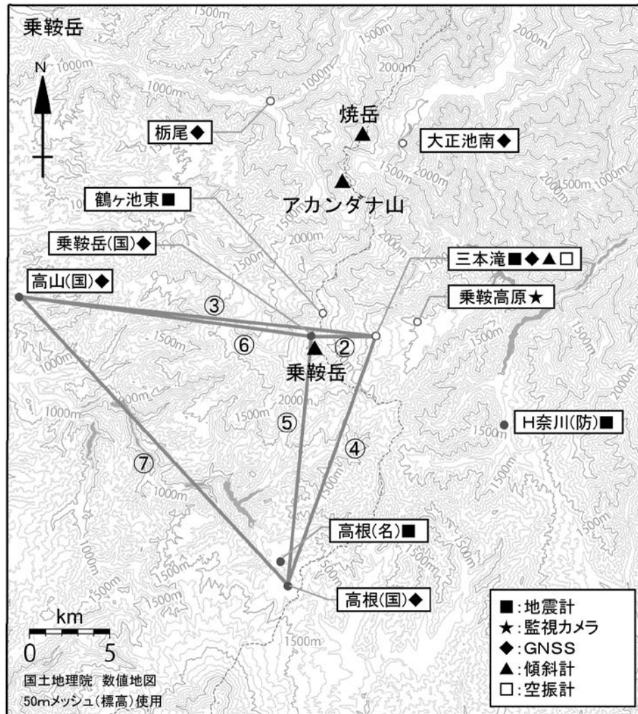
図 4 乗鞍岳 観測点配置図 GNSS 基線②～④は図 2 の②～④に対応しています。
