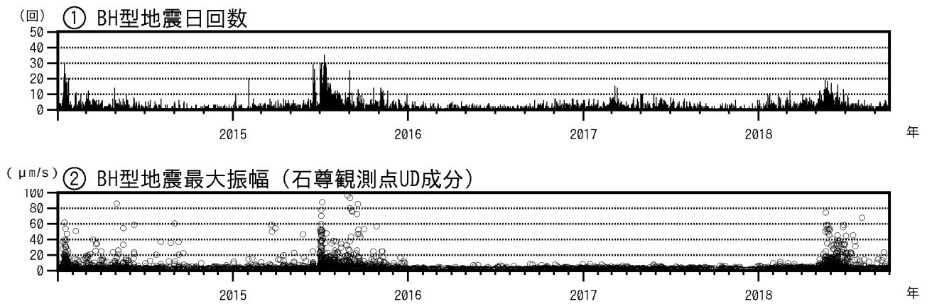
図 5 浅間山 BH 型地震の日別回数とその最大振幅（2014 年 1 月 1 日～2018 年 9 月 30 日）
