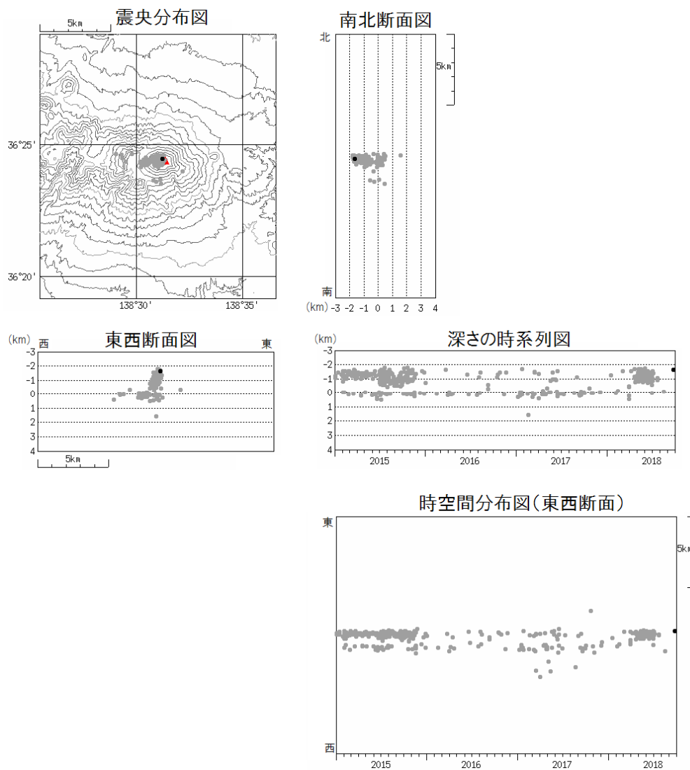
図 6 浅間山 震源分布図（2015 年 1 月 1 日～2018 年 9 月 30 日）
