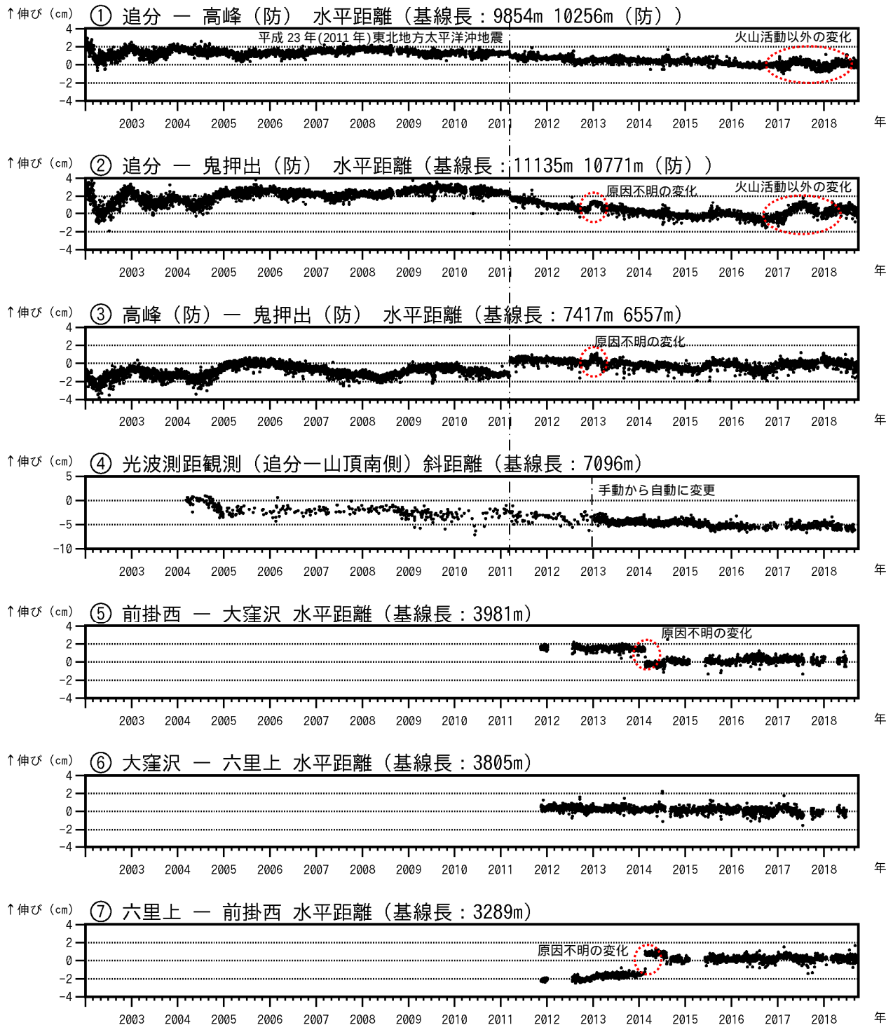
図7 - 1 浅間山 GNSS 連続観測及び光波測距観測の結果(2002年1月1日～2018年9月30日)
