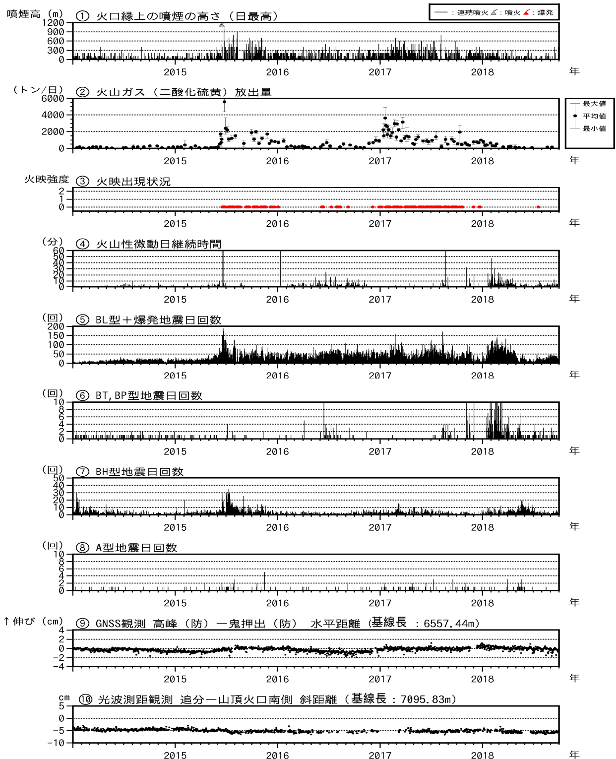
図 4 浅間山 最近の火山活動経過図（2014 年 1 月 1 日～2018 年 9 月 30 日）
