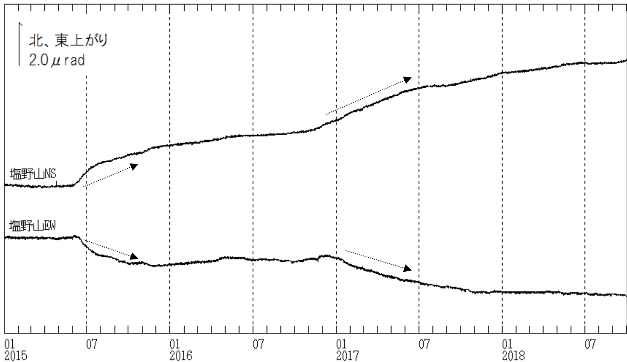
図 9 浅間山 塩野山観測点における傾斜データ（2015 年 1 月 1 日～2018 年 9 月 30 日）
