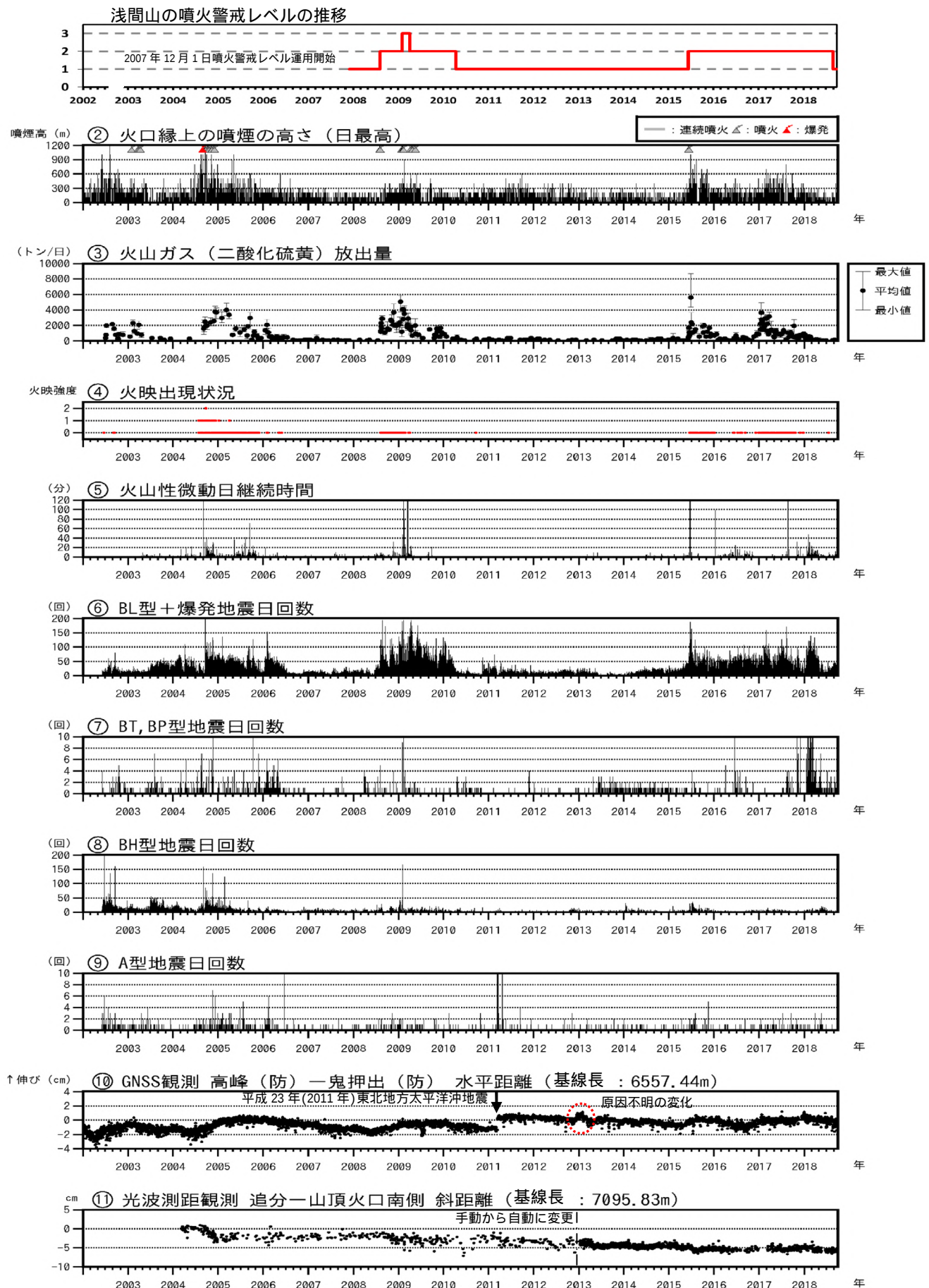
図3 浅間山 火山活動経過図（2002年1月1日～2018年9月30日）
