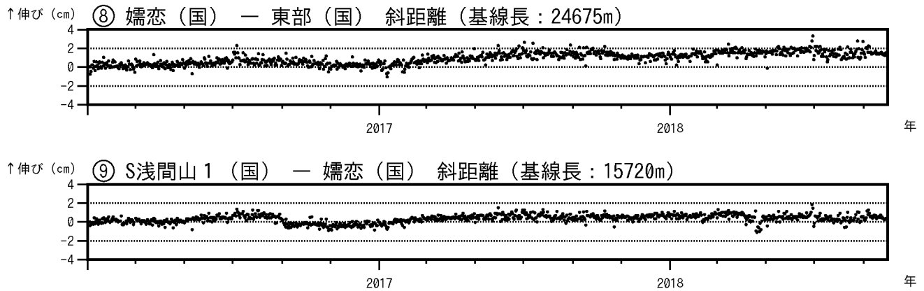
図 7 - 2 浅間山 GNSS 連続観測及び光波測距観測の結果(2016 年 1 月 1 日～2018 年 9 月 30 日) (国): 国土地理院 、 は図 8 の にそれぞれ対応しています。
