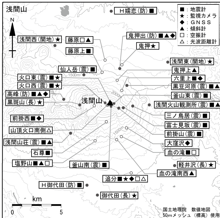
図 2 浅間山 観測点配置図
