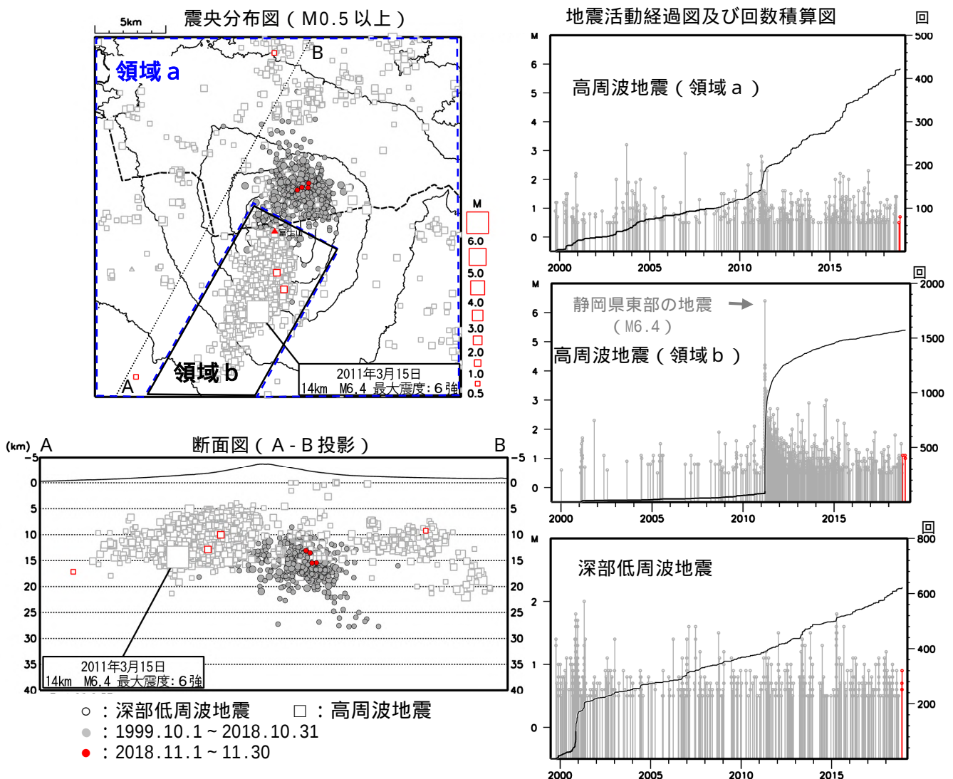
図 3 富士山 広域地震観測網による山体及び周辺の地震活動（1999 年 10 月 1 日～2018 年 11 月 30 日）
