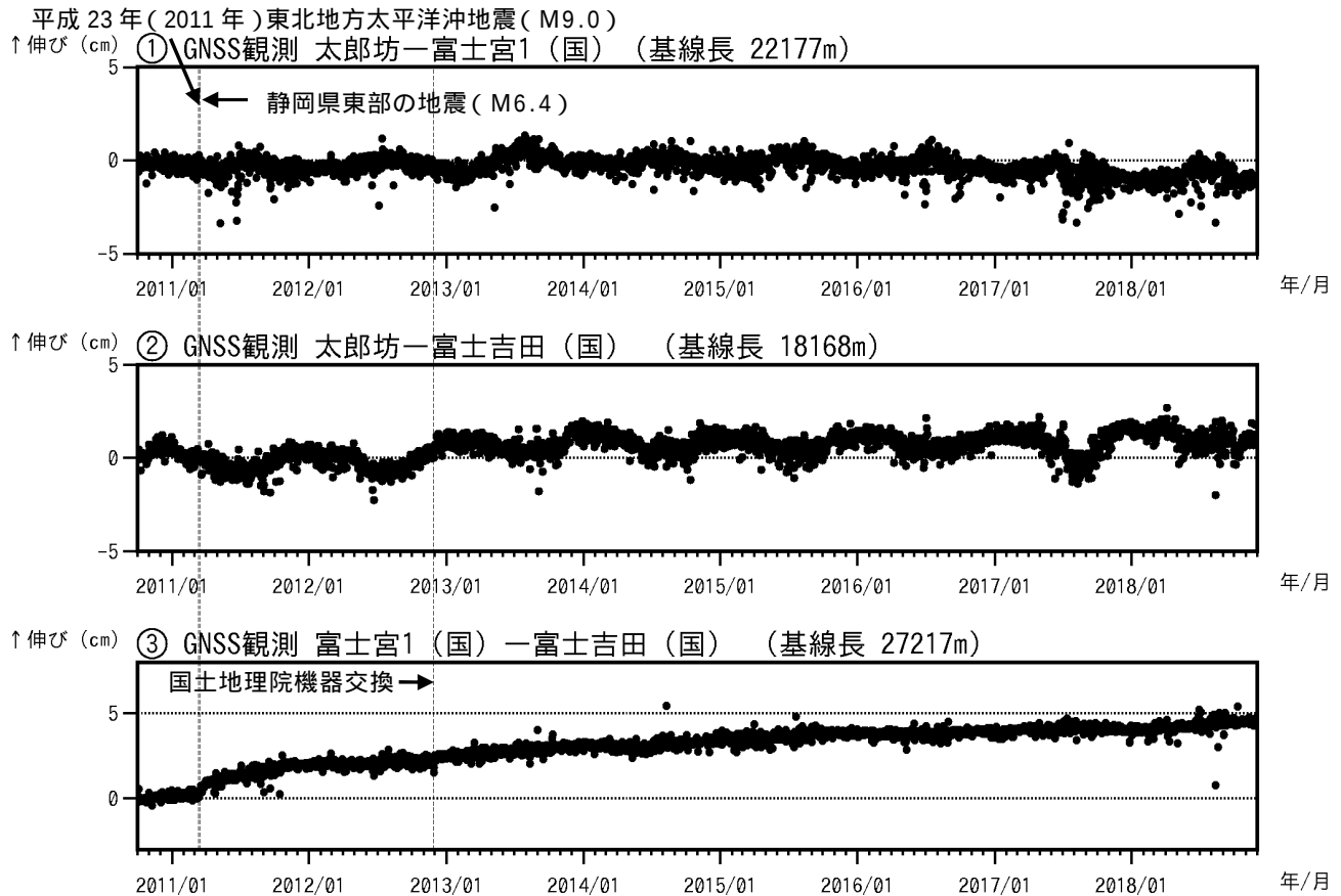
図4 富士山 GNSS連続観測による基線長変化（2010年10月1日～2018年11月30日）
