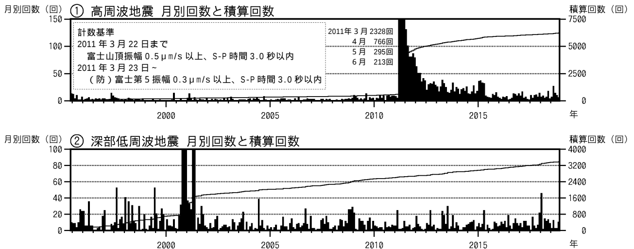
図 2 富士山 月別地震回数（1995 年 6 月 1 日～2018 年 11 月 30 日）
