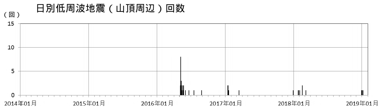
図 6 新潟焼山 日別地震回数（2014 年 1 月 1 日～2019 年 1 月 31 日）
