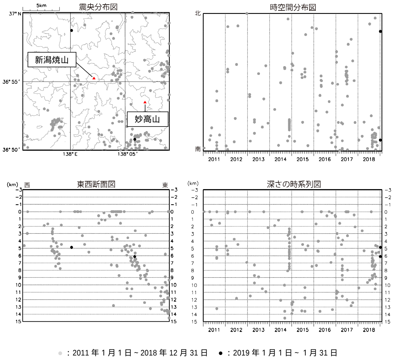
図 8 新潟焼山 広域地震観測網による山体・周辺の地震活動（2011 年 1 月 1 日～2019 年 1 月 31 日）
