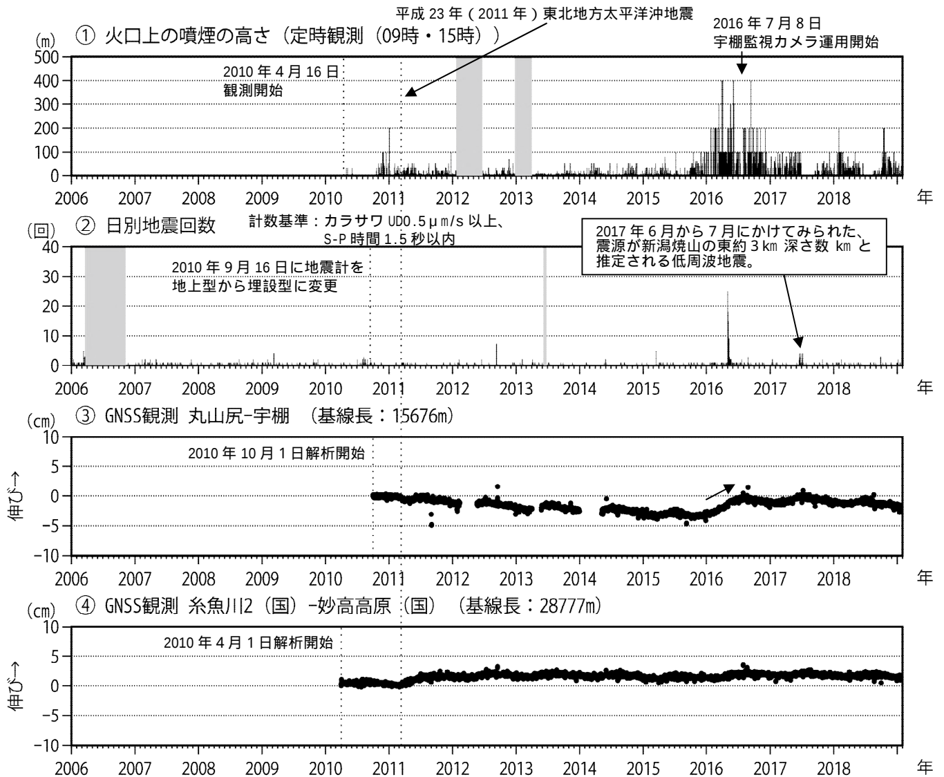
図 3 新潟焼山 火山活動経過図（2006 年 1 月 1 日～2019 年 1 月 31 日）
