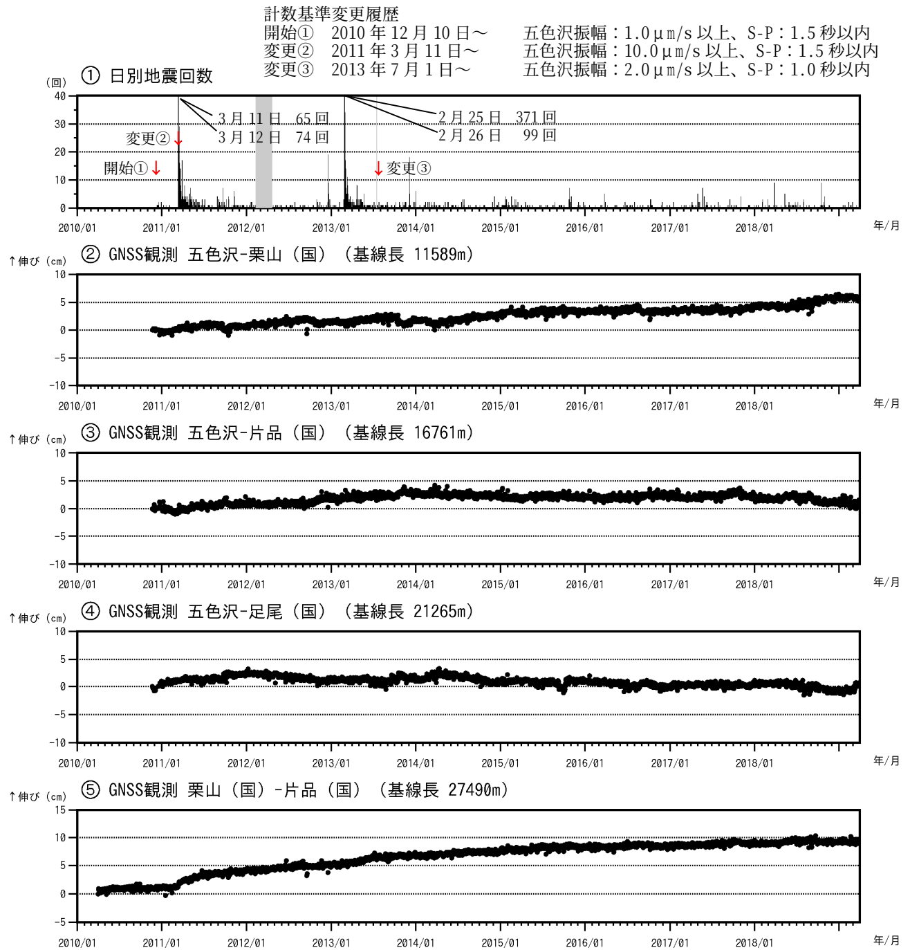
図2 日光白根山 火山活動経過図（2010 年 11 月 20 日～2019 年 3 月 31 日）
