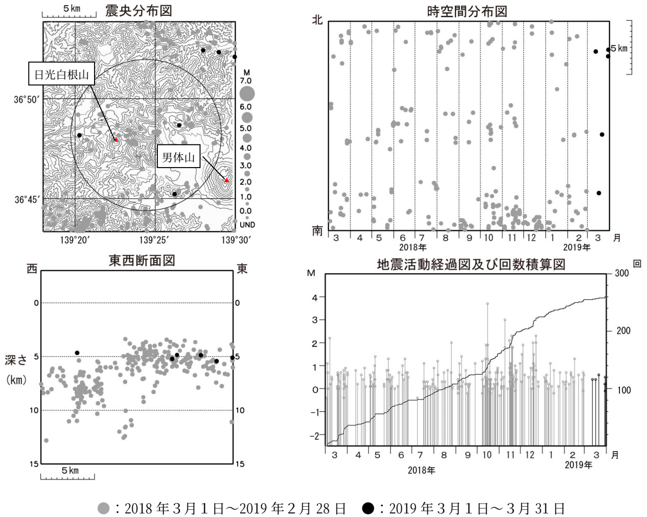
図3 日光白根山 広域地震観測網による山体・周辺の地震活動 (2018 年 3 月 1 日～2019 年 3 月 31 日)
