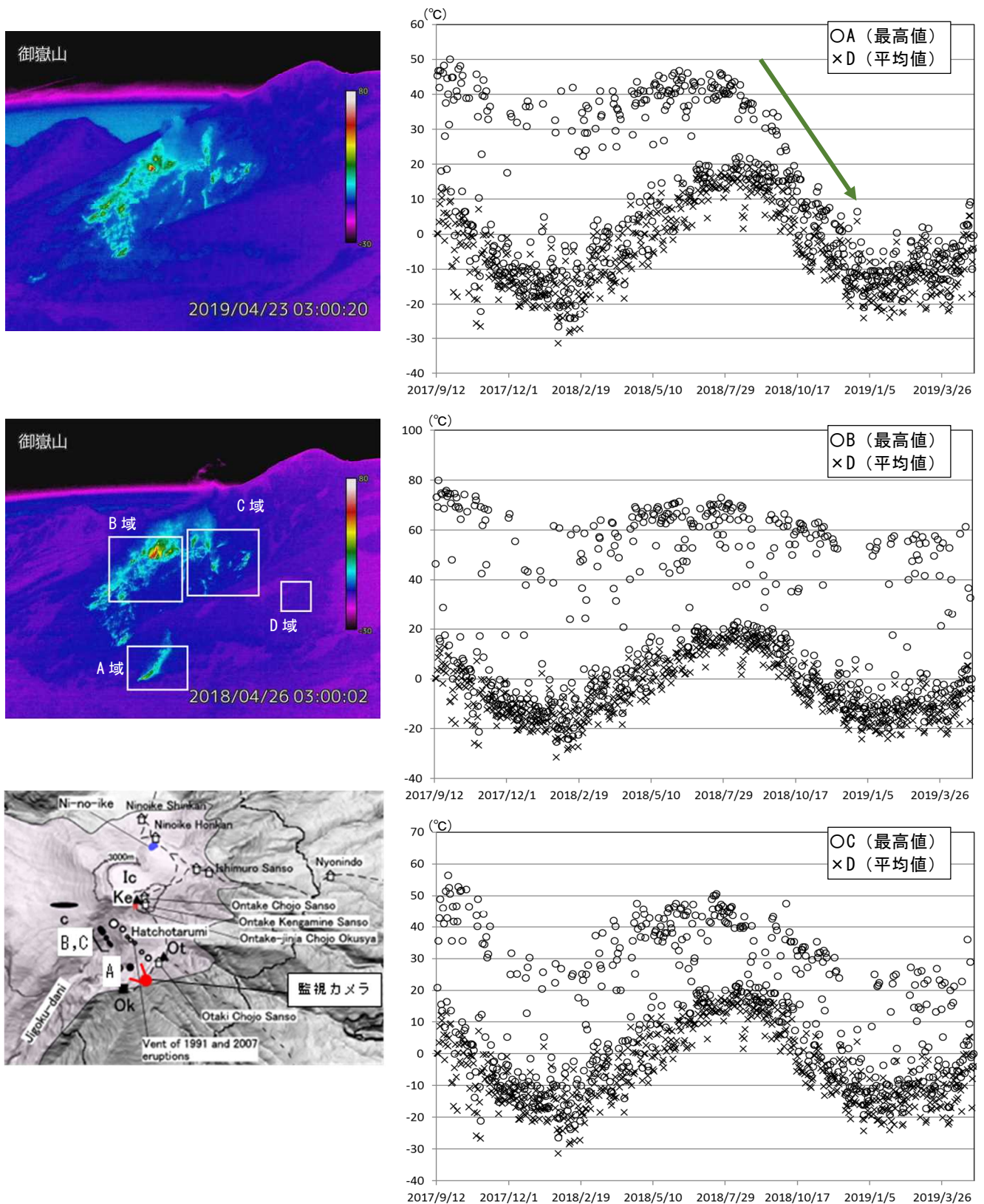
図3 御嶽山 奥の院赤外熱映像カメラによる剣ヶ峰南西側における最高温度の推移 (2017年9月13日～2019年4月30日)と同カメラの位置(Oikawa et al., 2016に加筆)
