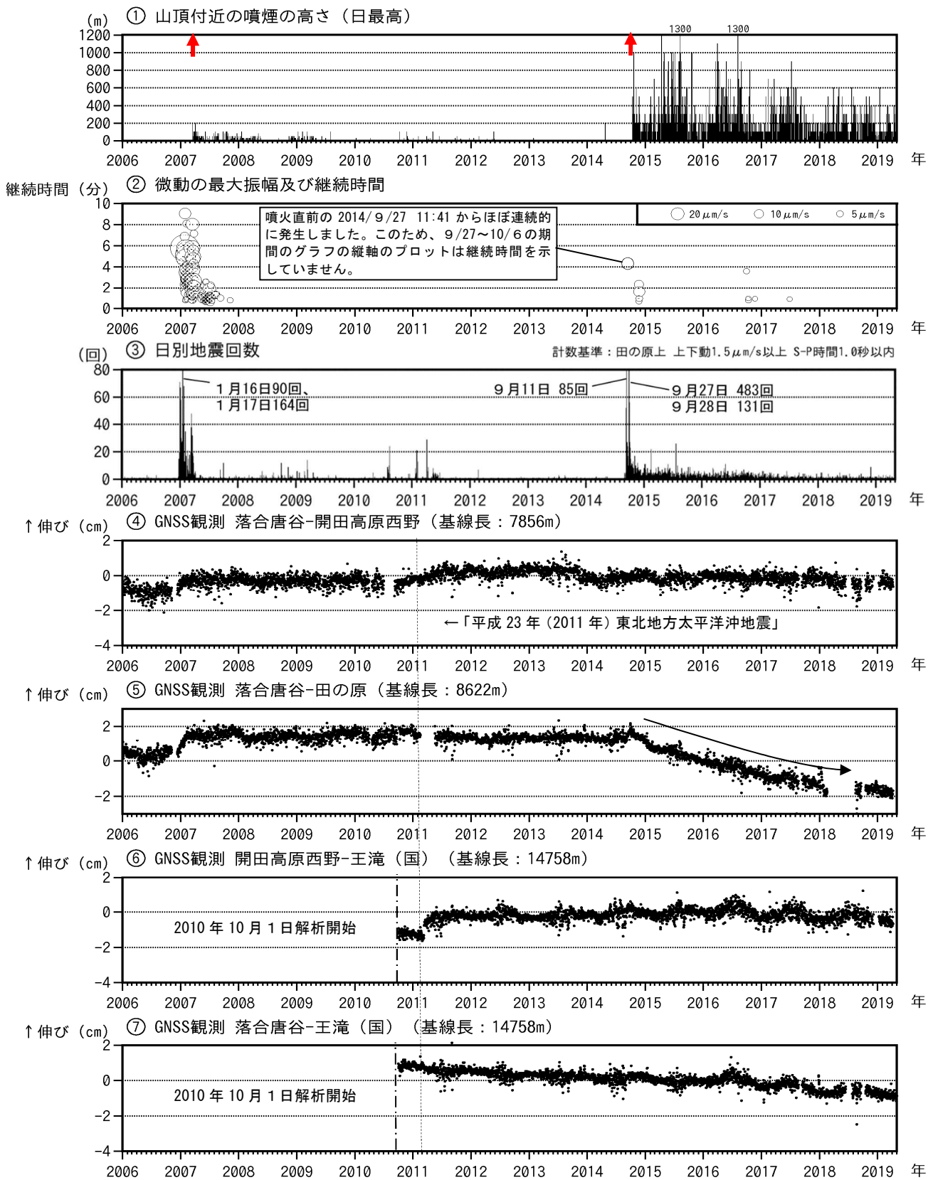
図5 御嶽山 長期間の火山活動経過図（2006年1月1日～2019年4月30日）
