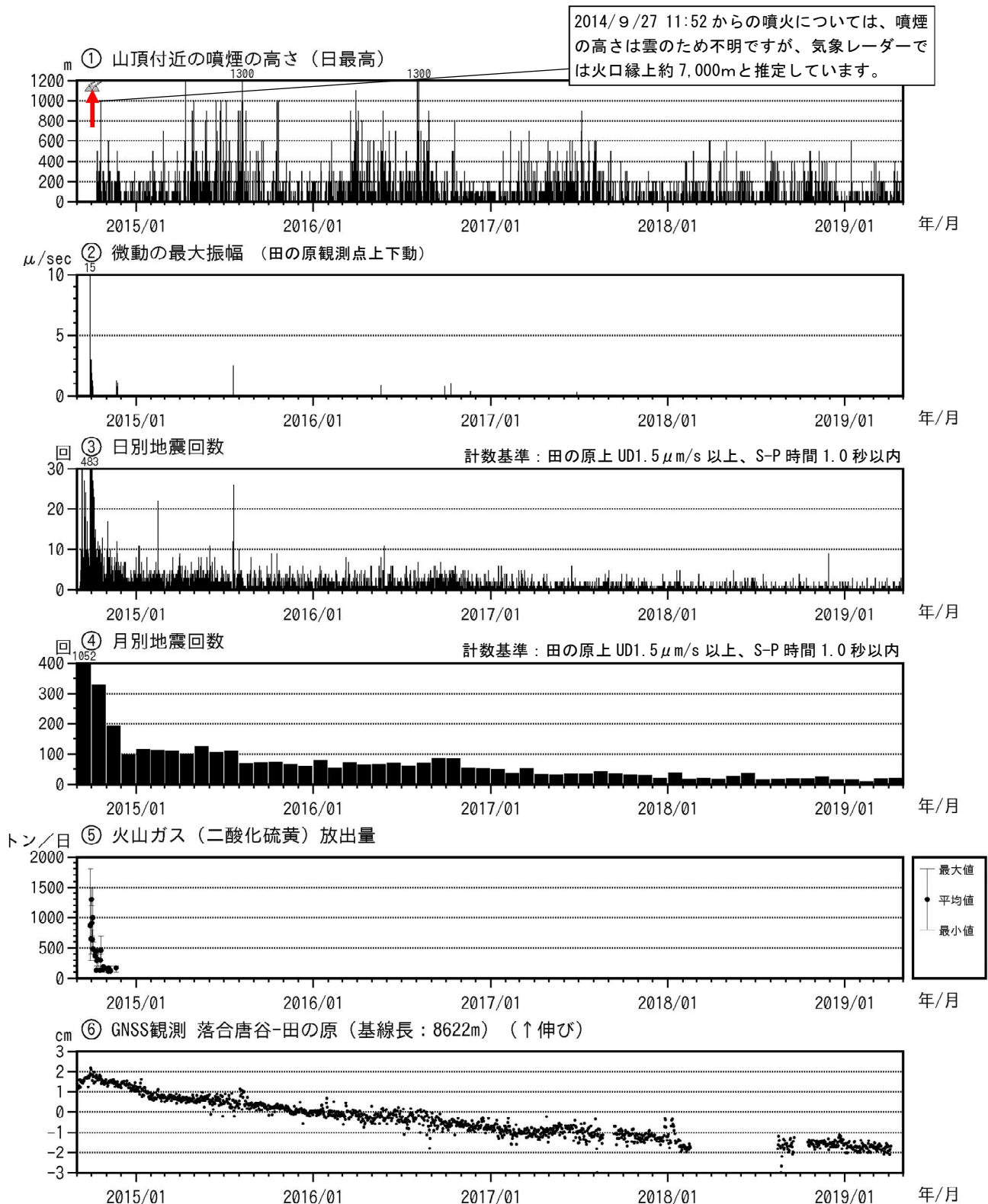
図 4 御嶽山 最近の火山活動経過図（2014 年 9 月 1 日～2019 年 4 月 30 日）
