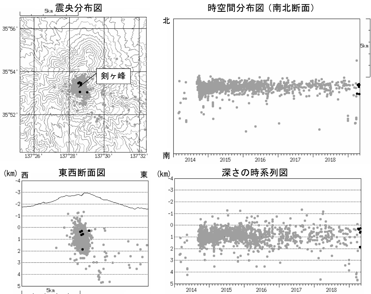
図 2 御嶽山 震源分布図（2014 年 1 月 1 日～2019 年 4 月 30 日）
