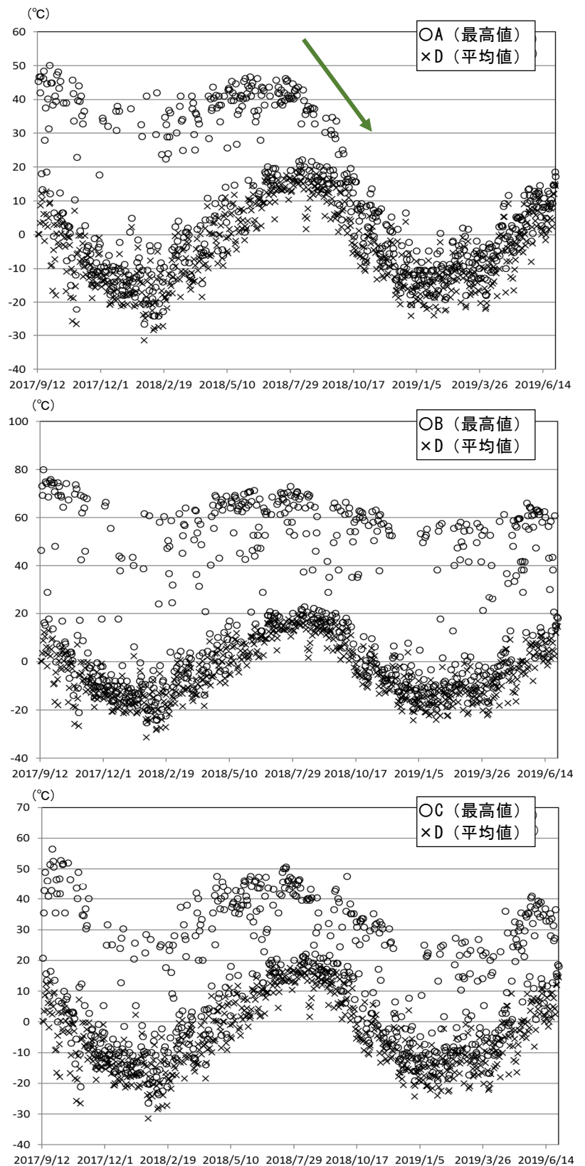
図9 御嶽山 奥の院赤外線熱映像カメラによる剣ヶ峰南西側における最高温度の推移
