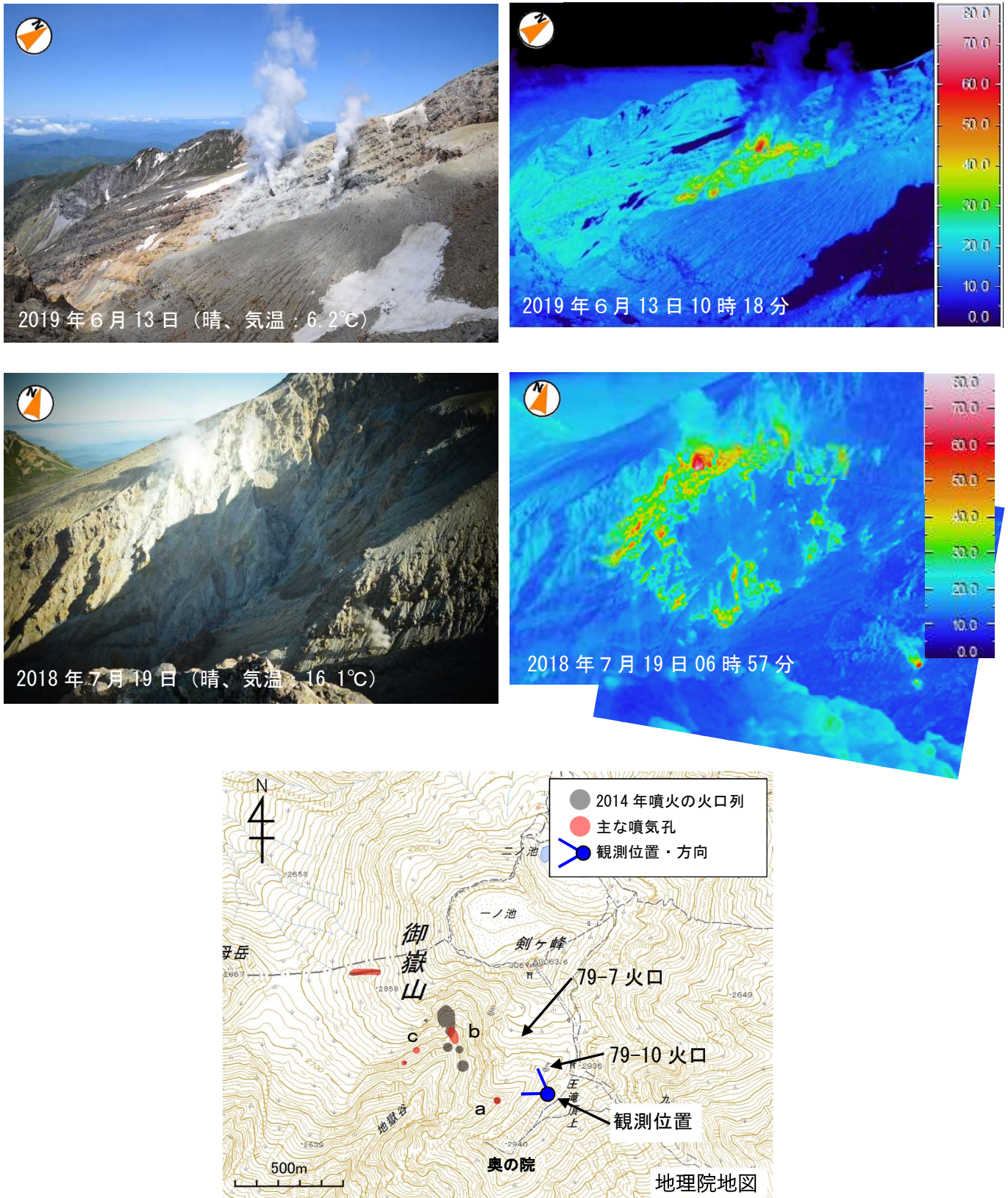
図3 御嶽山 地獄谷（図1-b c方向）の可視画像と赤外熱映像装置による地表面温度分布（奥の院より撮影） ・ 6月13日に実施した機動観測では、2014年に噴火が発生した剣ヶ峰山頂の南西側の火口列の一部の噴気孔で、引き続き活発な噴気活動がみられ、温度の高い部分が認められました。
