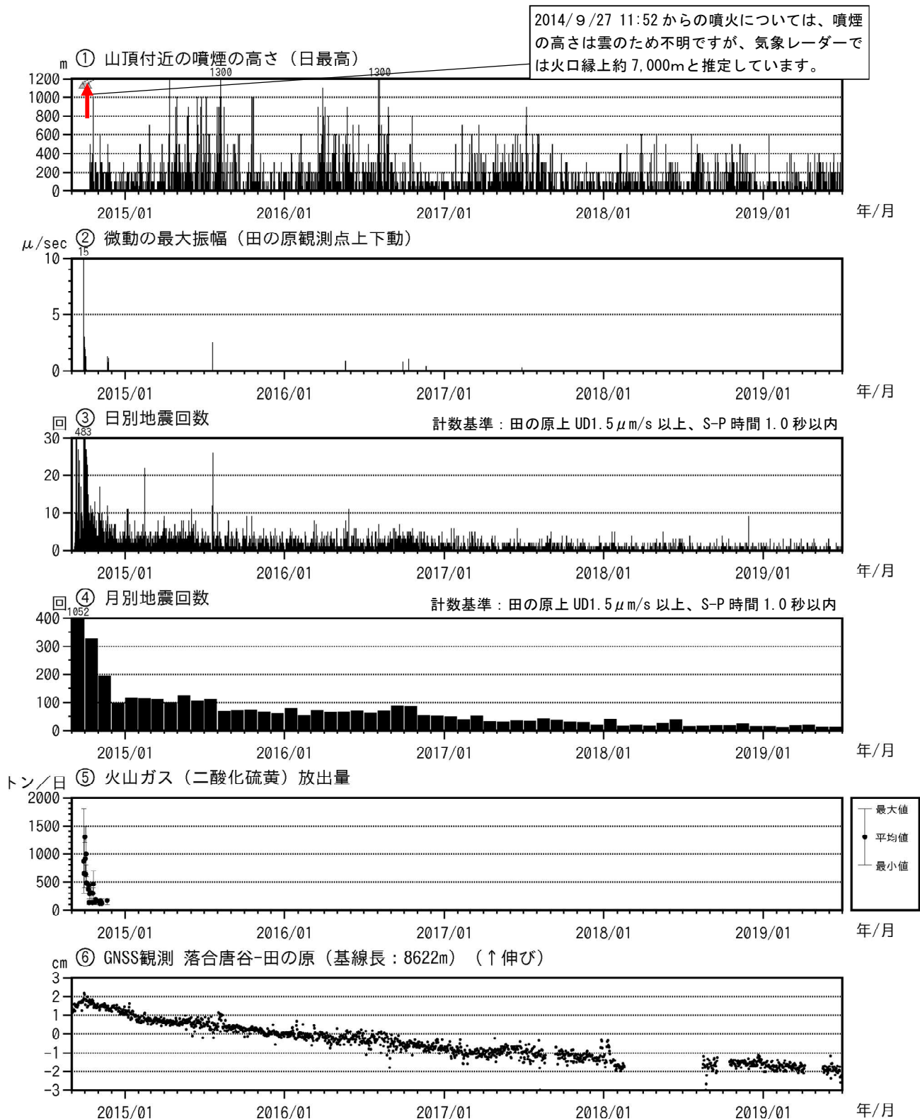
図10 御嶽山 最近の火山活動経過図（2014年9月1日～2019年6月30日）
