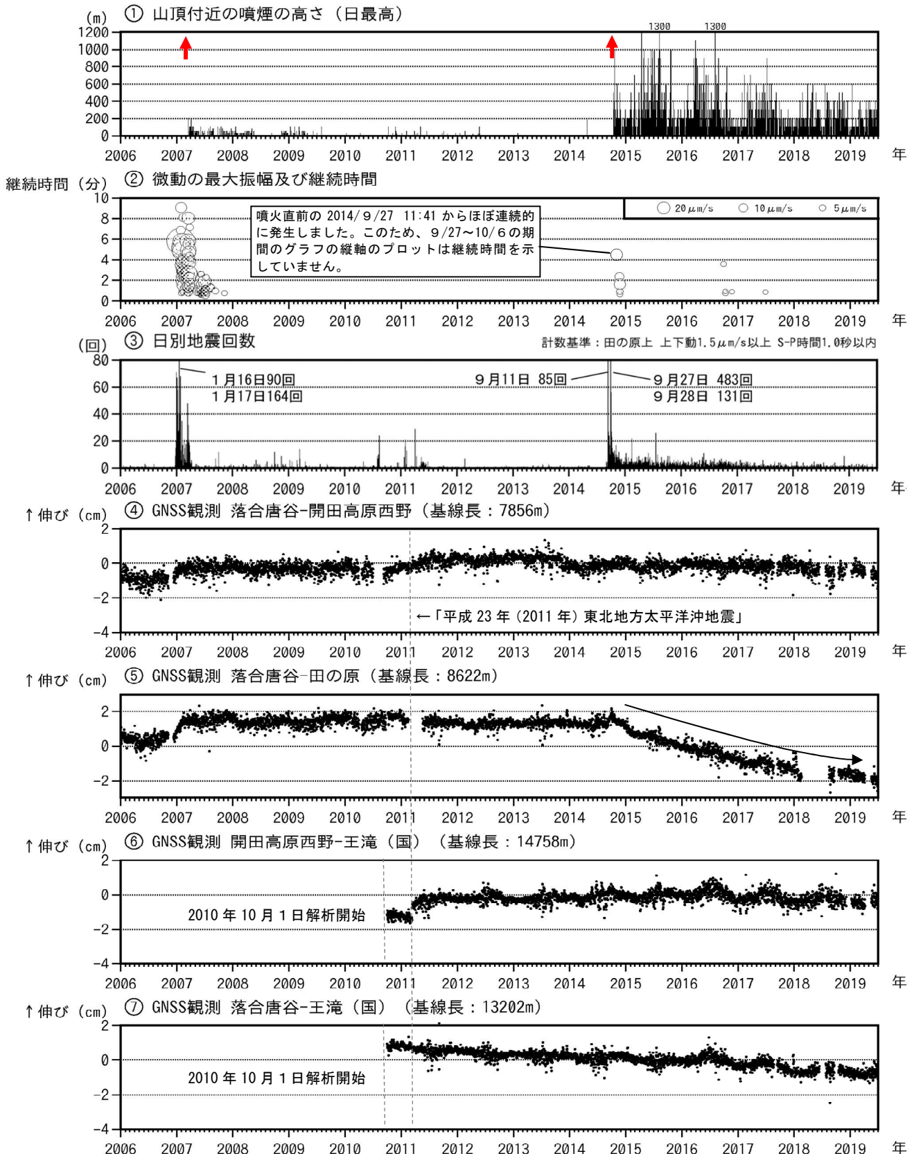
図11 御嶽山 長期間の火山活動経過図（2006年1月1日～2019年6月30日）
