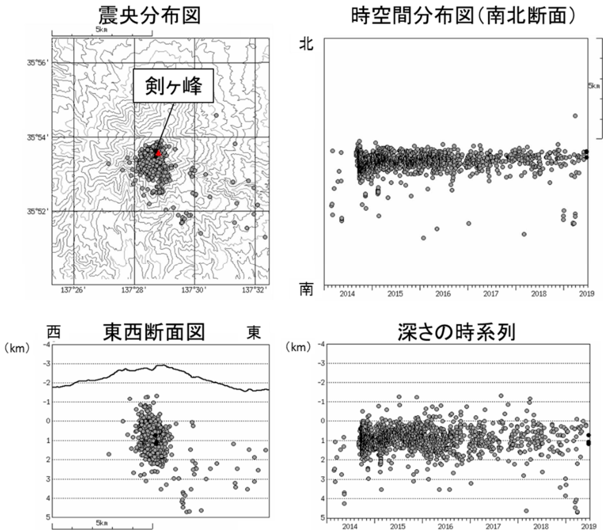
図8 御嶽山 震源分布図（2014年1月1日～2019年6月30日）
