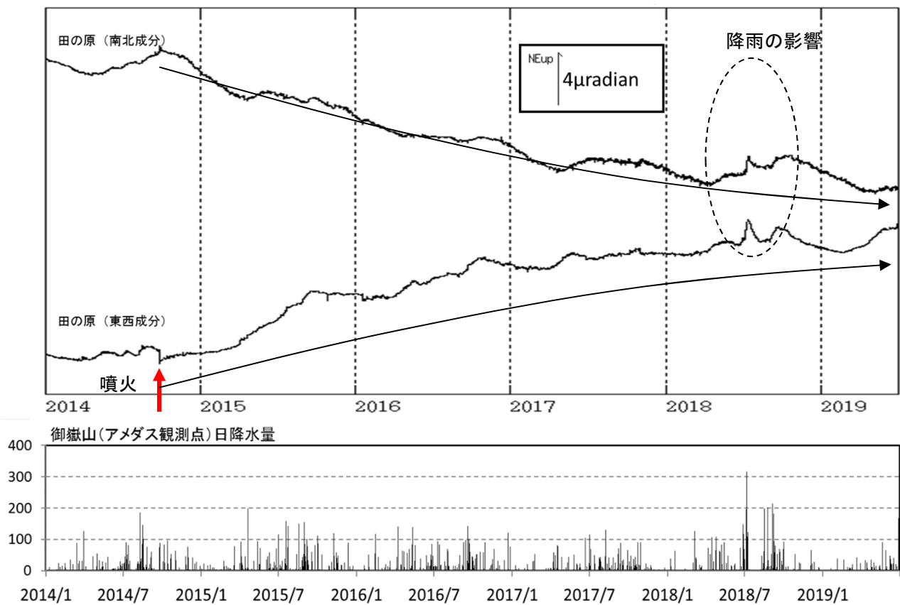
図 13 御嶽山 田の原観測点の傾斜変動（2014 年 1 月 1 日～2019 年 6 月 30 日）
