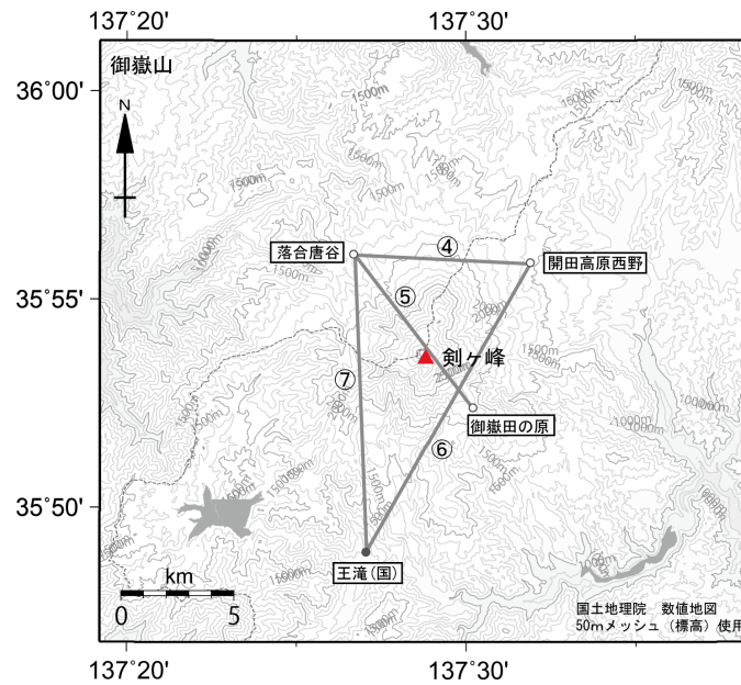
図 12 御嶽山 GNSS 連続観測点と基線番号
