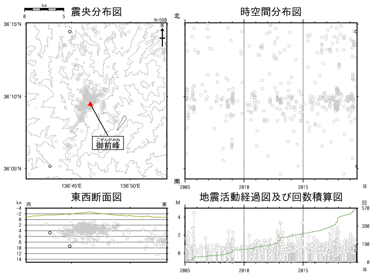
図4 白山 広域地震観測網による山体・周辺の地震活動（2005 年 1 月 1 日～2019 年 7 月 31 日）
