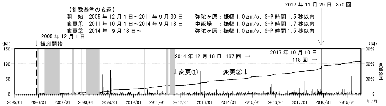
図3 白山 日別地震回数と積算回数（2005 年 12 月 1 日～2019 年 7 月 31 日）
