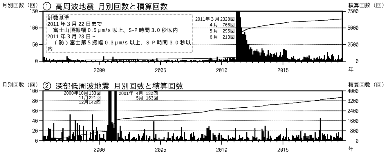
図2 富士山 月別地震回数（1995年6月1日～2019年10月31日）
