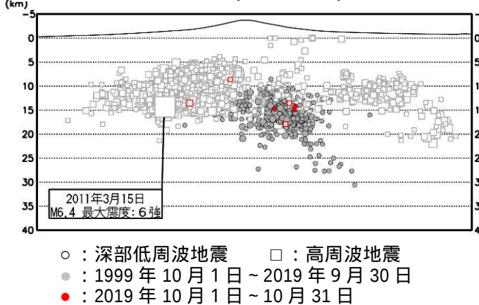
図3 富士山 広域地震観測網による山体及び周辺の地震活動（1999年10月1日～2019年10月31日）
