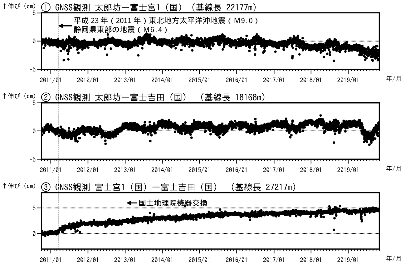
図 4 富士山 GNSS 連続観測による基線長変化 (2010 年 10 月 1 日 ~ 2019 年 10 月 31 日) (国): 国土地理院 「平成 23 年 (2011 年) 東北地方太平洋沖地震」及び 2011 年 3 月 15 日に発生した静岡県東部の地震 (M6.4) によるステップ状の変化を補正しています。 ~ は図 5 の GNSS 基線 ~ に対応しています。
