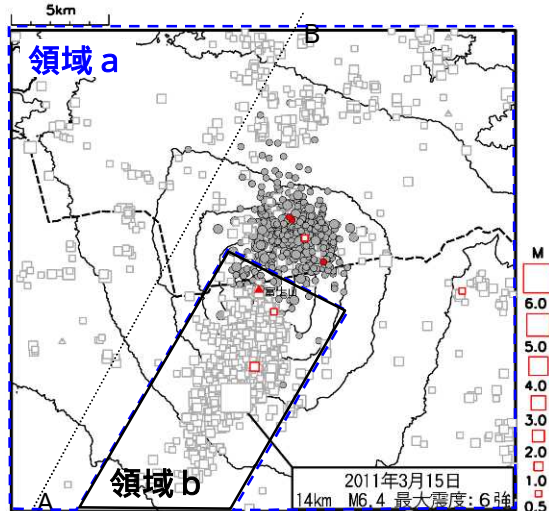
震央分布図（M0.5以上）
