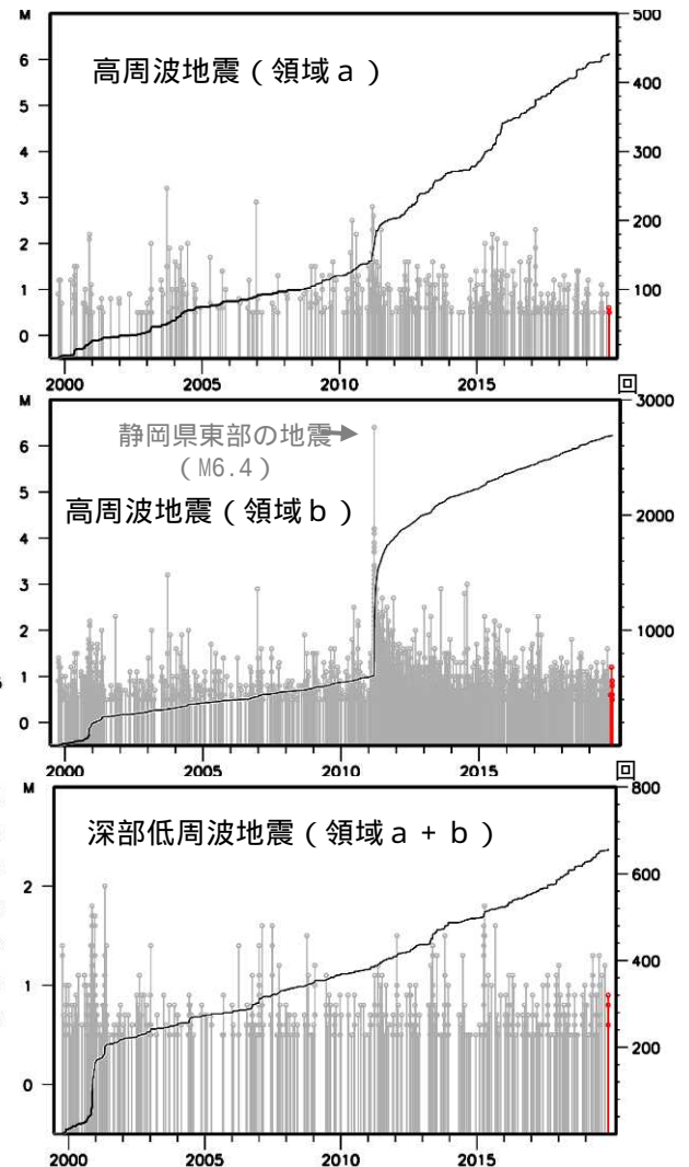
図3 富士山 広域地震観測網による山体及び周辺の地震活動（1999年10月1日～2019年10月31日）
