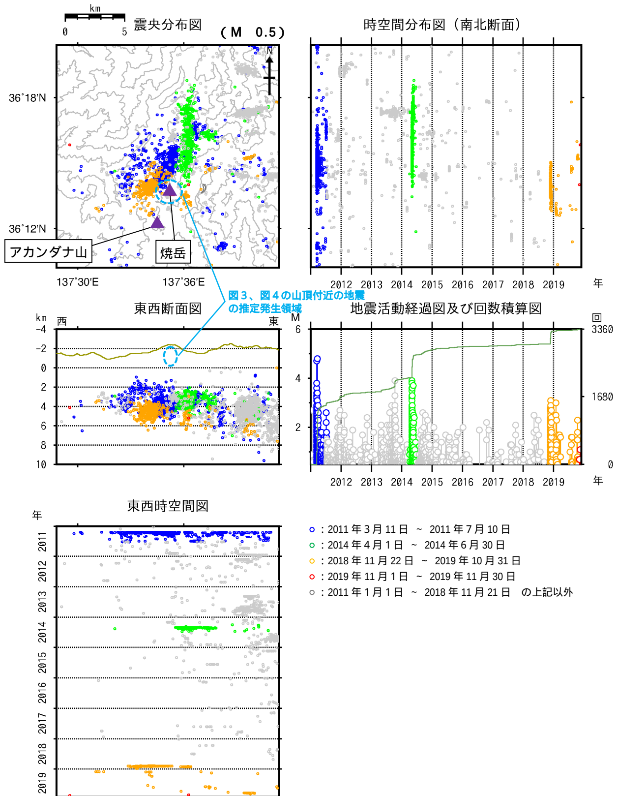
図 5 焼岳 広域地震観測網による山体及び周辺の地震活動(2011年 1 月 1 日 ~ 2019年11月30日)
