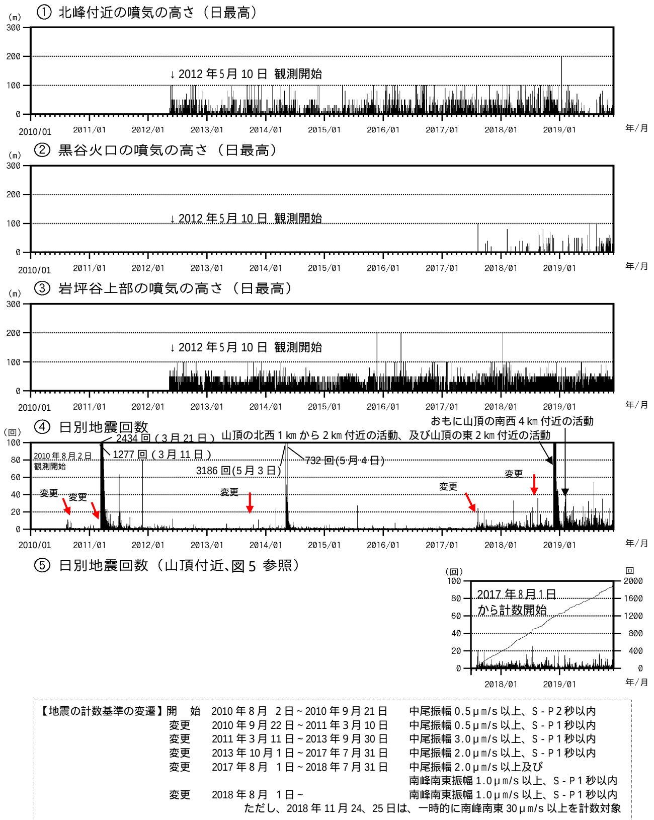
図 3 焼岳 噴気の高さと地震回数の推移(2010 年 8 月 2 日 ~ 2019 年 11 月 30 日)
