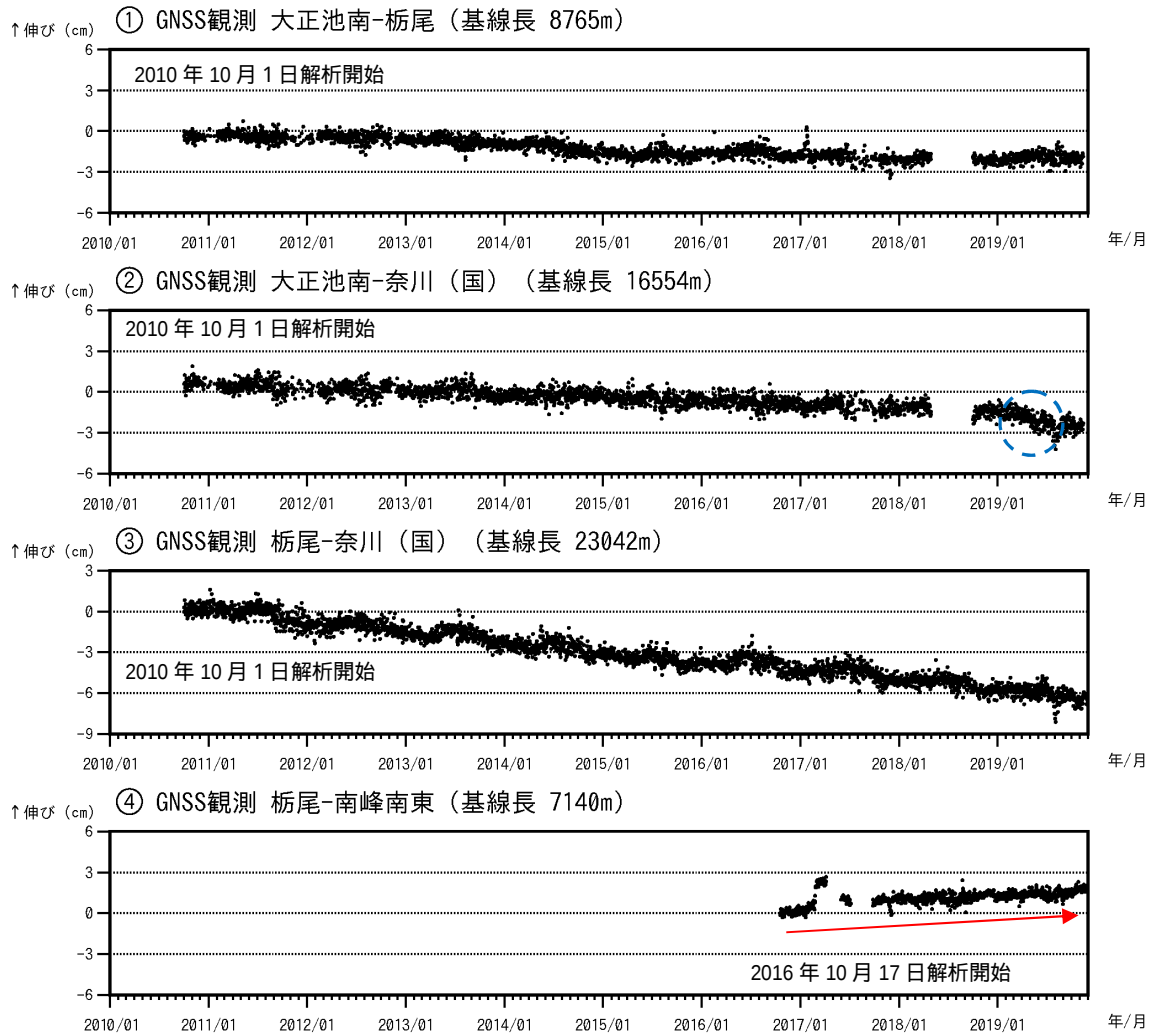
図6 焼岳 GNSS 連続観測による基線長変化（2010年10月1日～2019年11月30日）
