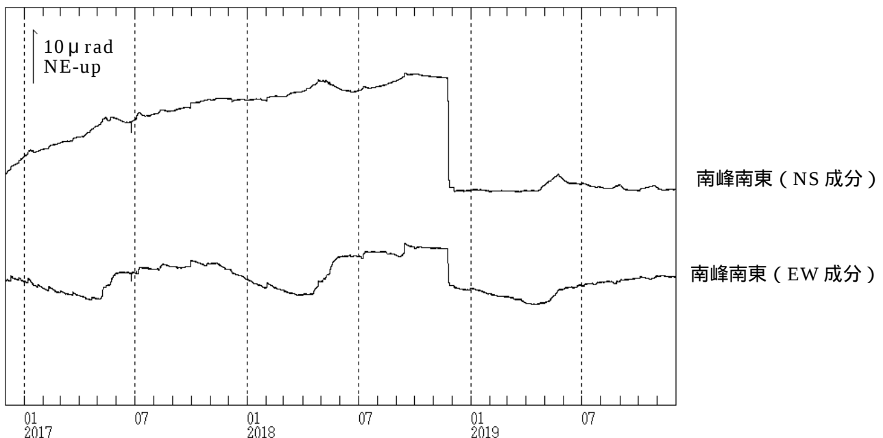
図7 焼岳 南峰南東観測点における傾斜データ（2016年12月1日～2019年11月30日）
