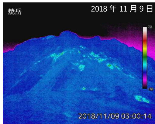
図2 焼岳 中尾峠赤外熱映像カメラによる焼岳の北側斜面の地表面温度分布と可視画像
