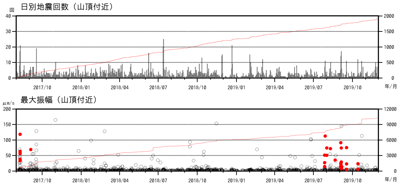
図4 焼岳 山頂付近の地震回数、および南峰南東観測点上下動最大振幅 (2017年8月1日～2019年11月30日)
