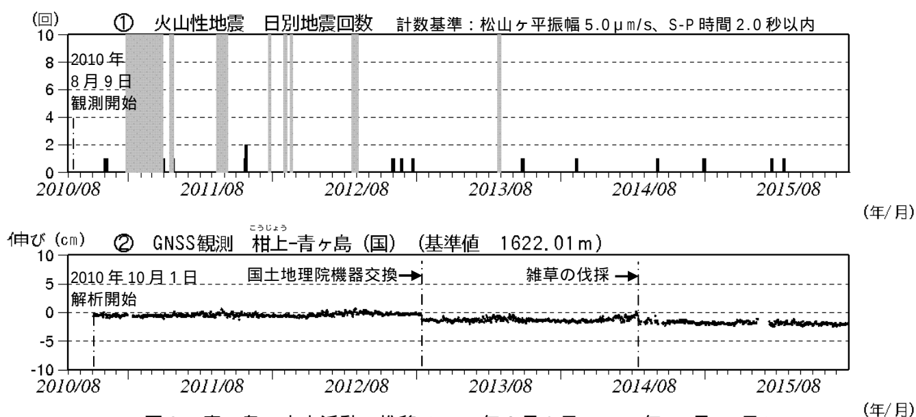
図 2 青ヶ島 火山活動の推移 (2010 年 8 月 9 日～2015 年 12 月 31 日)
