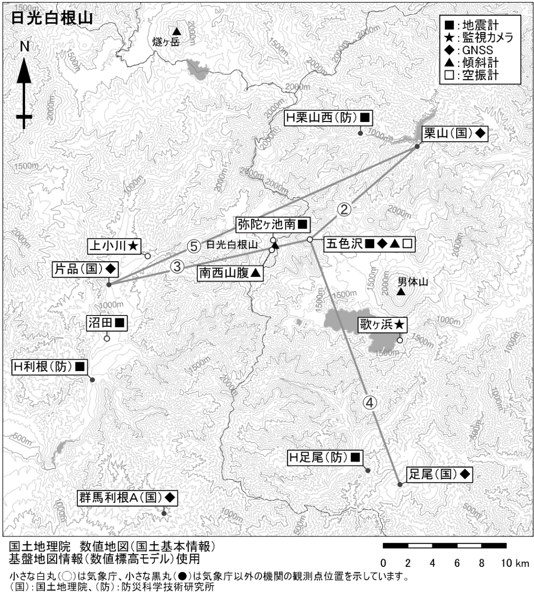
図4 日光白根山 観測点配置 GNSS 基線②～⑤は図2の②～⑤に対応しています。
