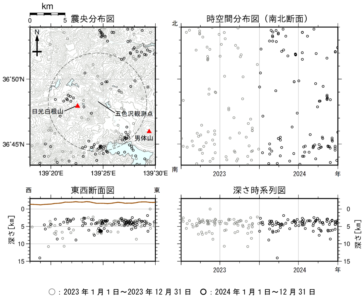
図3 日光白根山 広域地震観測網による山体周辺の地震活動 (2023 年 1 月 1 日～2024 年 12 月 31 日)
