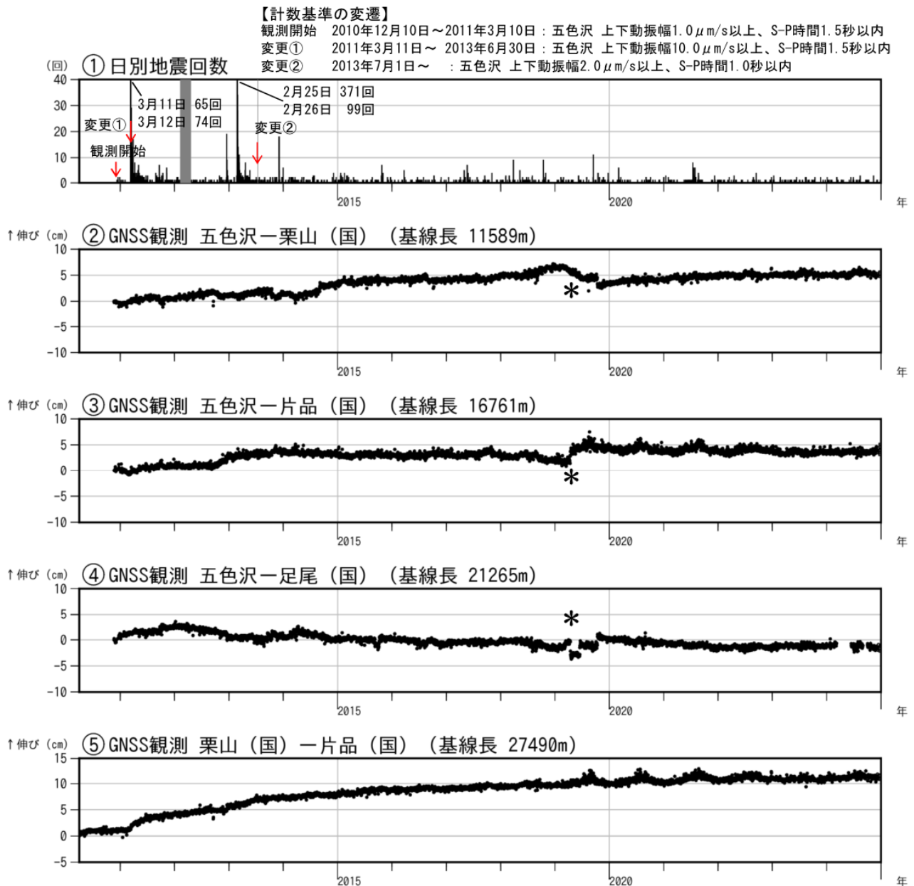
図2 日光白根山 火山活動経過図 (2010年4月1日～2024年12月31日)
