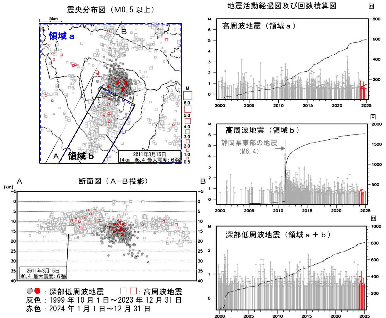
図4 富士山 広域地震観測網による山体及び周辺の地震活動(1999年10月1日～2024年12月31日)
