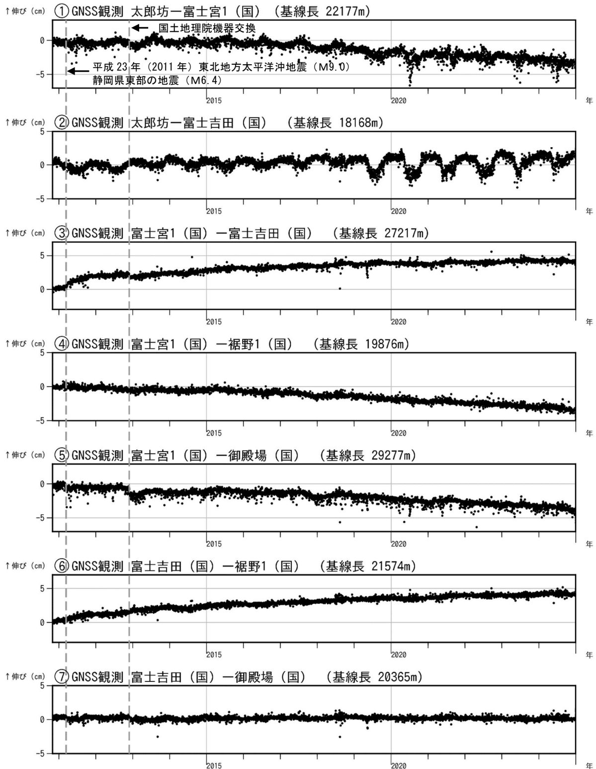
図5 富士山 GNSS 連続観測による基線長変化 (2010 年 10 月 1 日～2024 年 12 月 31 日)
