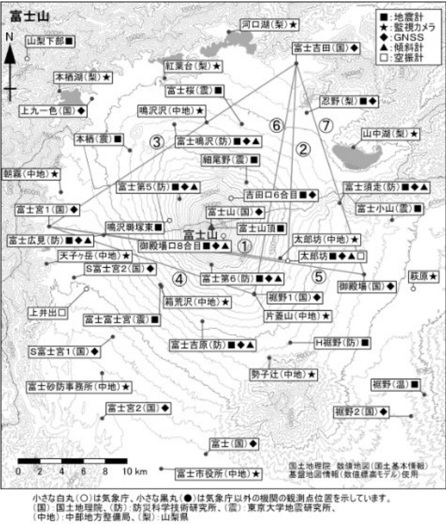
図6 富士山 観測点配置図 GNSS 基線①～⑦は図5の①～⑦に対応しています。
