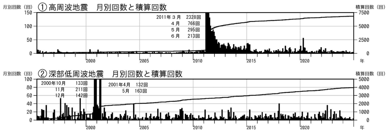
図2 富士山 月別地震回数（1995年6月1日～2024年12月31日）
