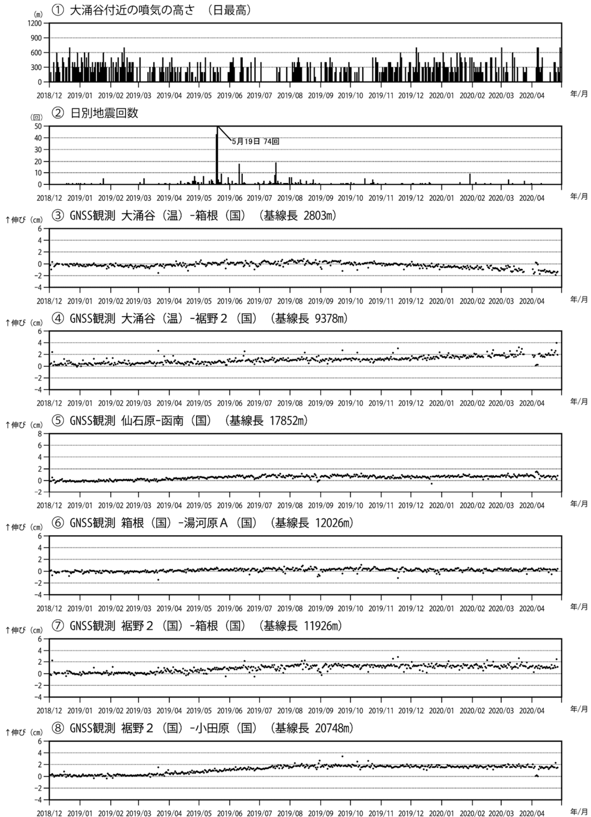
図7 箱根山 火山活動経過図（2018年12月1日～2020年4月30日）
