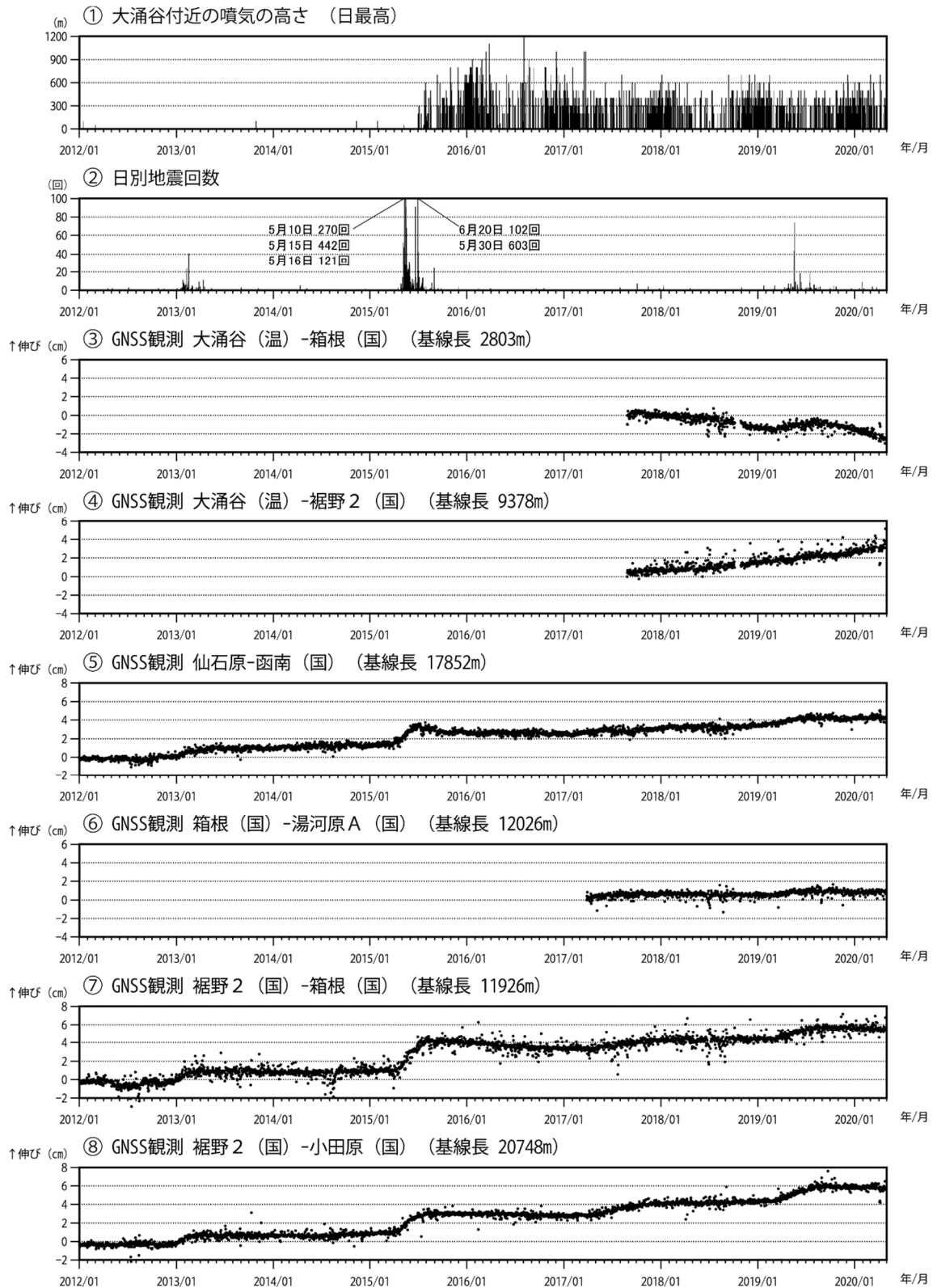
図6 箱根山 火山活動経過図（2012年1月1日～2020年4月30日）
