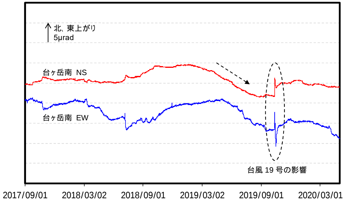
図9 箱根山 台ヶ岳南観測点における傾斜データ（2017年9月1日～2020年4月30日）
