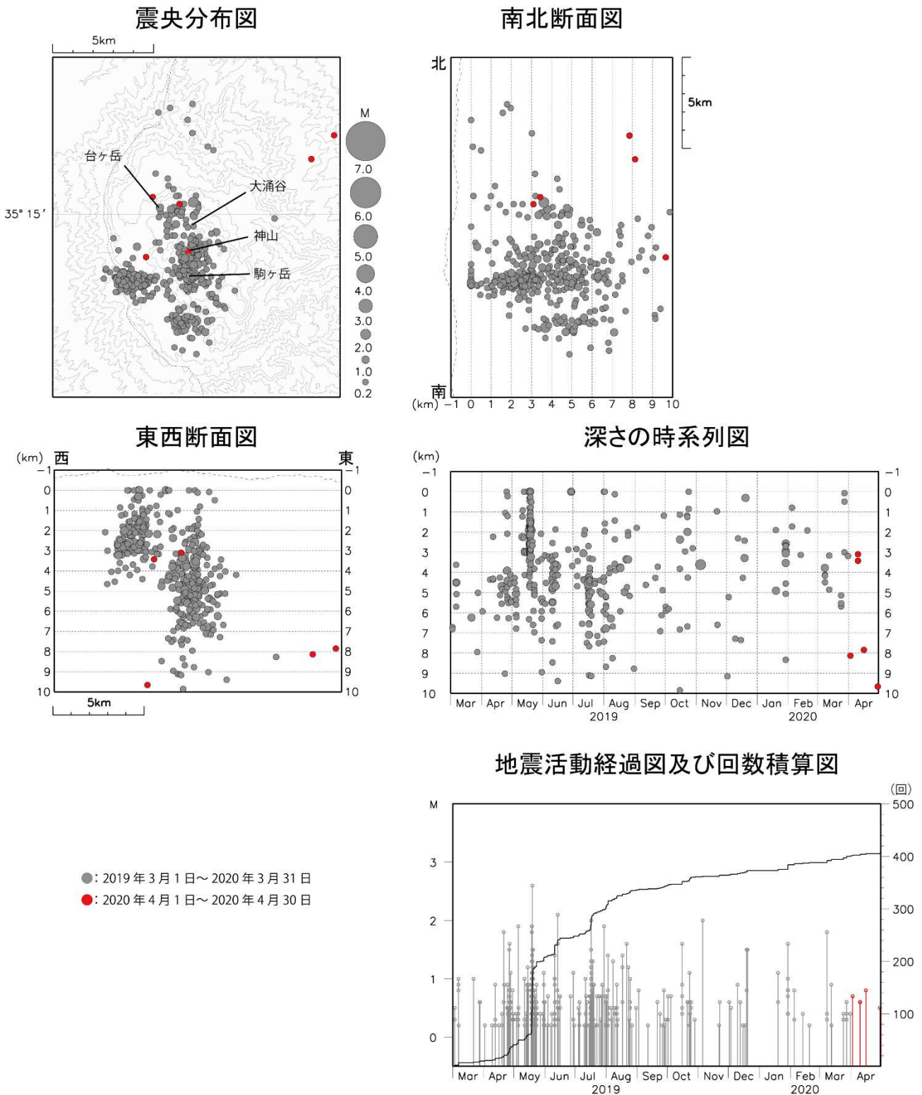
図8 箱根山 広域地震観測網による山体周辺の震源分布図(2019年3月1日～2020年4月30日) M(マグニチュード)は地震の規模を表し、M0.2以上の地震を表示しています。 広域地震観測網により震源決定したもので、深さは全て海面以下として決定しています。 図中の震源要素は一部暫定値が含まれており、後日変更することがあります。 2020年4月18日以降の地震について、暫定的に震源精査の基準を変更しているため、それ以前と比較して微小な地震での震源決定数の変化(増減)が見られます。 地震活動は低調に経過しました。
