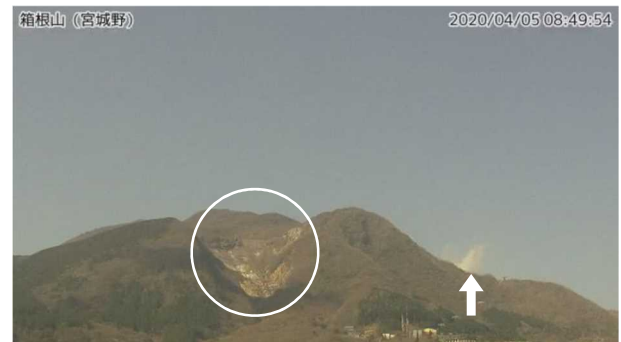
図4 箱根山 早雲地獄の状況 （4月5日、宮城野監視カメラによる） 円内は早雲地獄からの噴気の状況。 宮城野監視カメラでは、大涌谷からの噴気（矢印）は高さ概ね 100m 以上の場合に観測されます。
