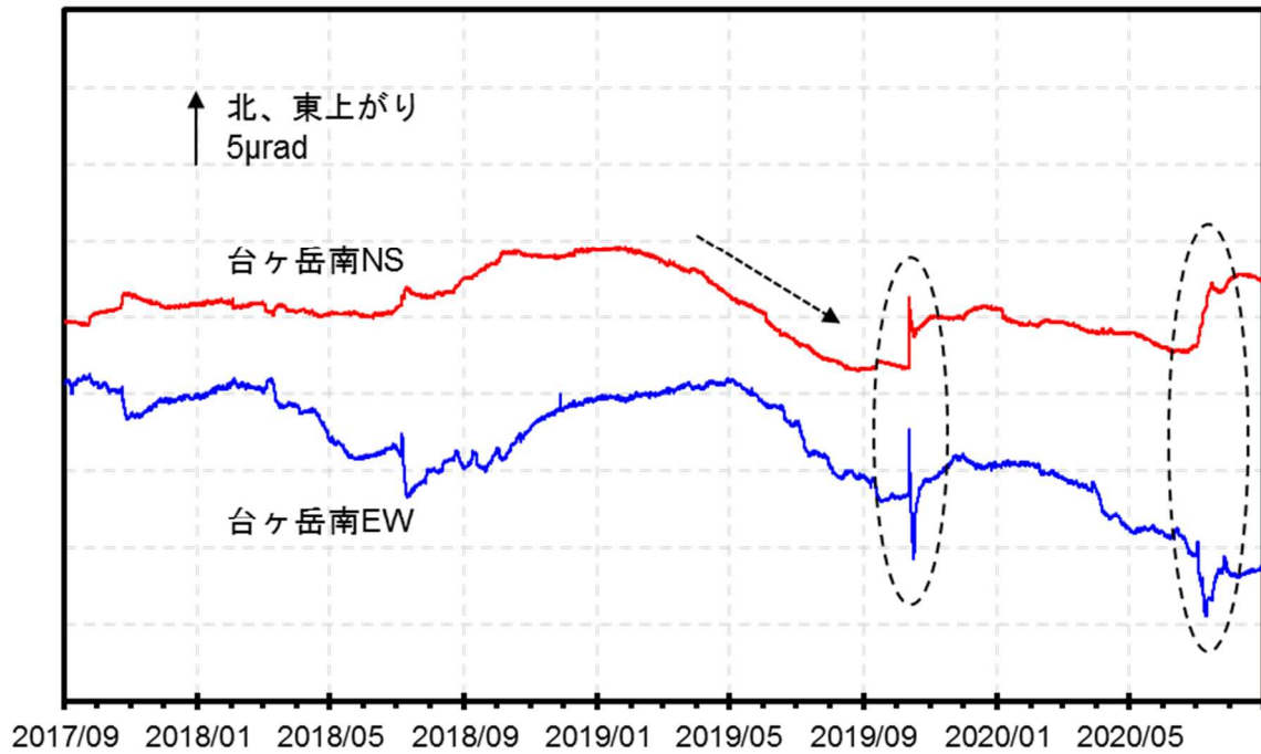
図9 箱根山 台ヶ岳南観測点における傾斜データ（2017年9月1日～2020年8月31日） 破線で囲んだ部分は降水による影響と考えられる変動を示す。
