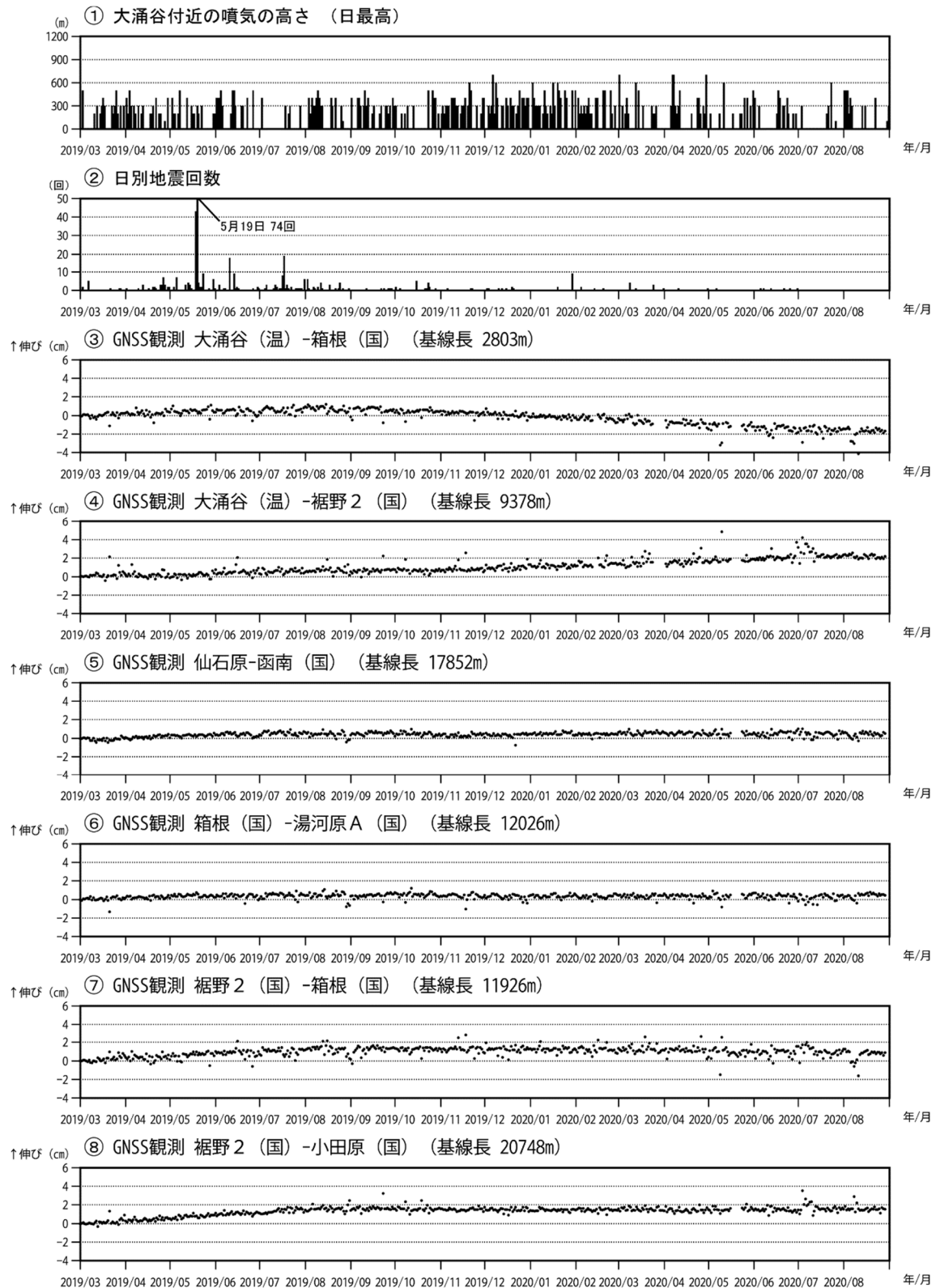
図7 箱根山 火山活動経過図（2019年3月1日～2020年8月31日）
