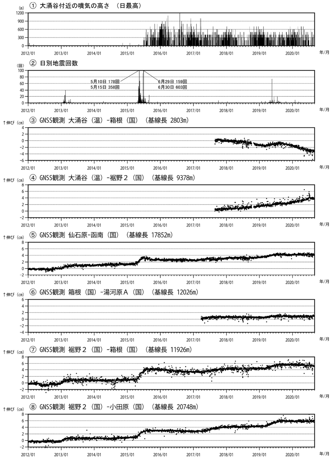
図6 箱根山 火山活動経過図（2012年1月1日～2020年8月31日）
