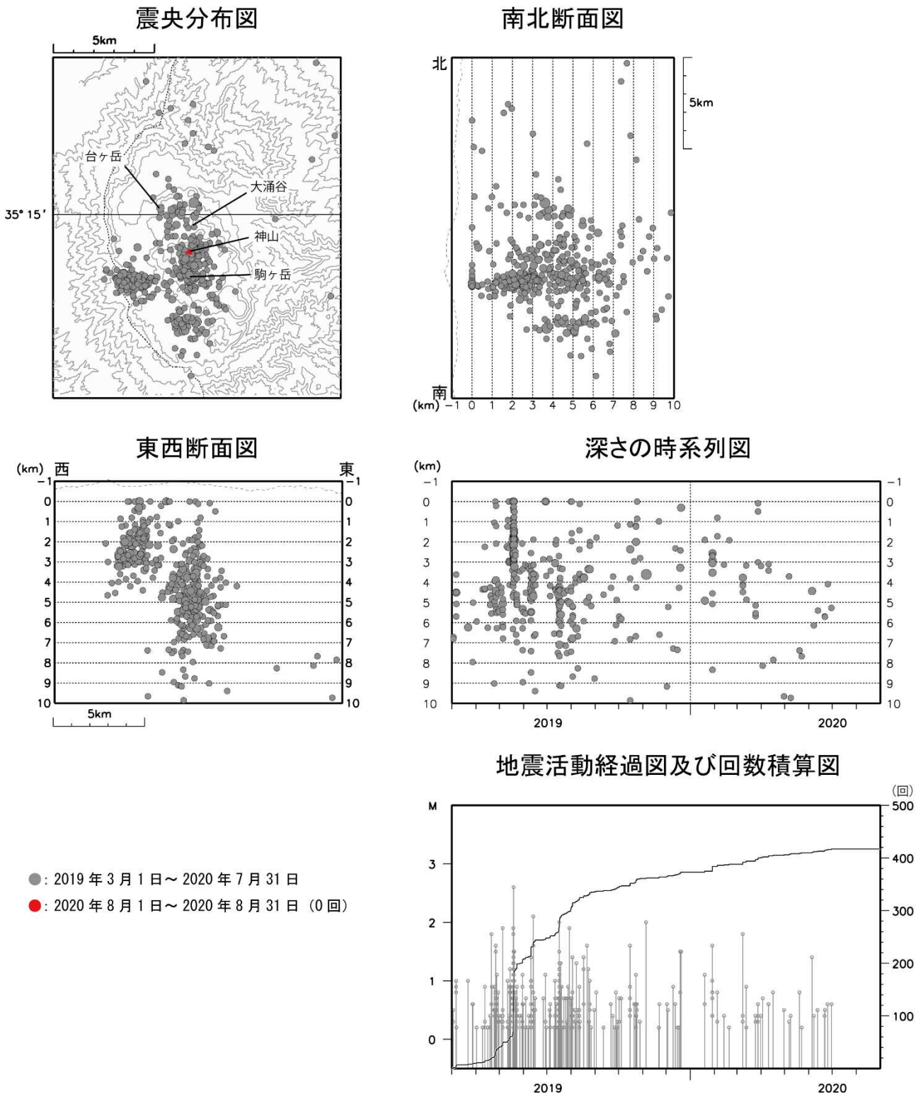
図8 箱根山 広域地震観測網による山体周辺の震源分布図(2019年3月1日～2020年8月31日) M(マグニチュード)は地震の規模を表し、M0.2以上の地震を表示しています。 広域地震観測網により震源決定したもので、深さは全て海面以下として決定しています。 図中の震源要素は一部暫定値が含まれており、後日変更することがあります。 2020年4月18日以降の地震について、暫定的に震源精査の基準を変更しているため、それ以前と比較して微小な地震での震源決定数の変化(増減)が見られます。
