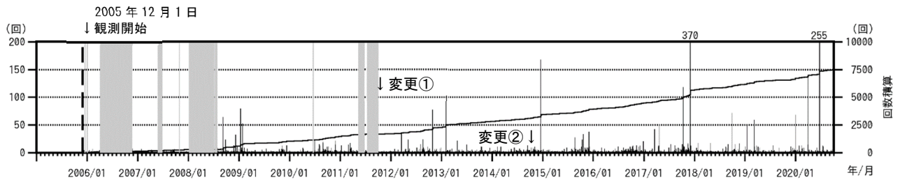
図3 白山 日別地震回数と積算回数（2005年12月1日～2020年9月30日） 図の灰色部分は機器障害による欠測期間
