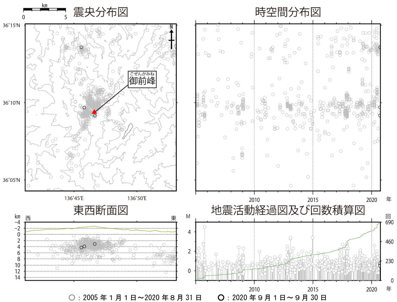
図4 白山 広域地震観測網による山体・周辺の地震活動（2005年1月1日～2020年9月30日）
