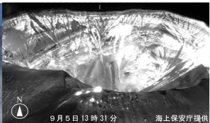
図2 西之島 上空からの観測による噴煙および火口内の状況
