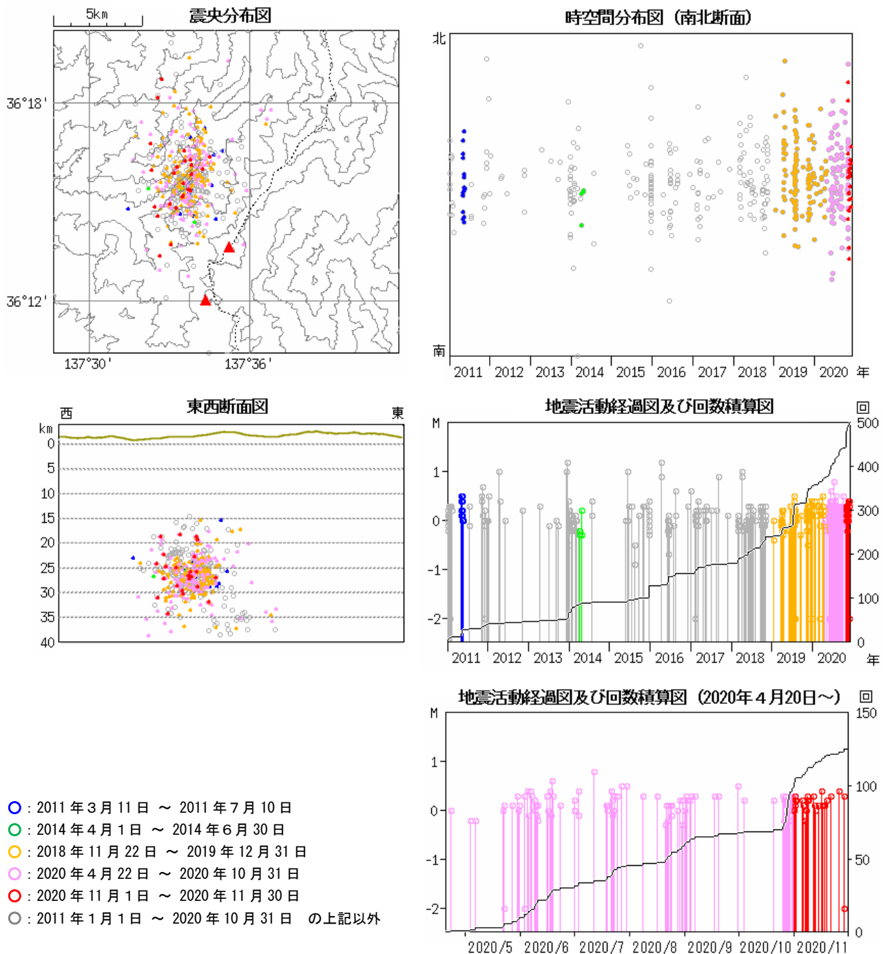
図3 焼岳 深部低周波地震の震源分布図（広域地震観測網による）（2011年1月1日～2020年11月30日）
