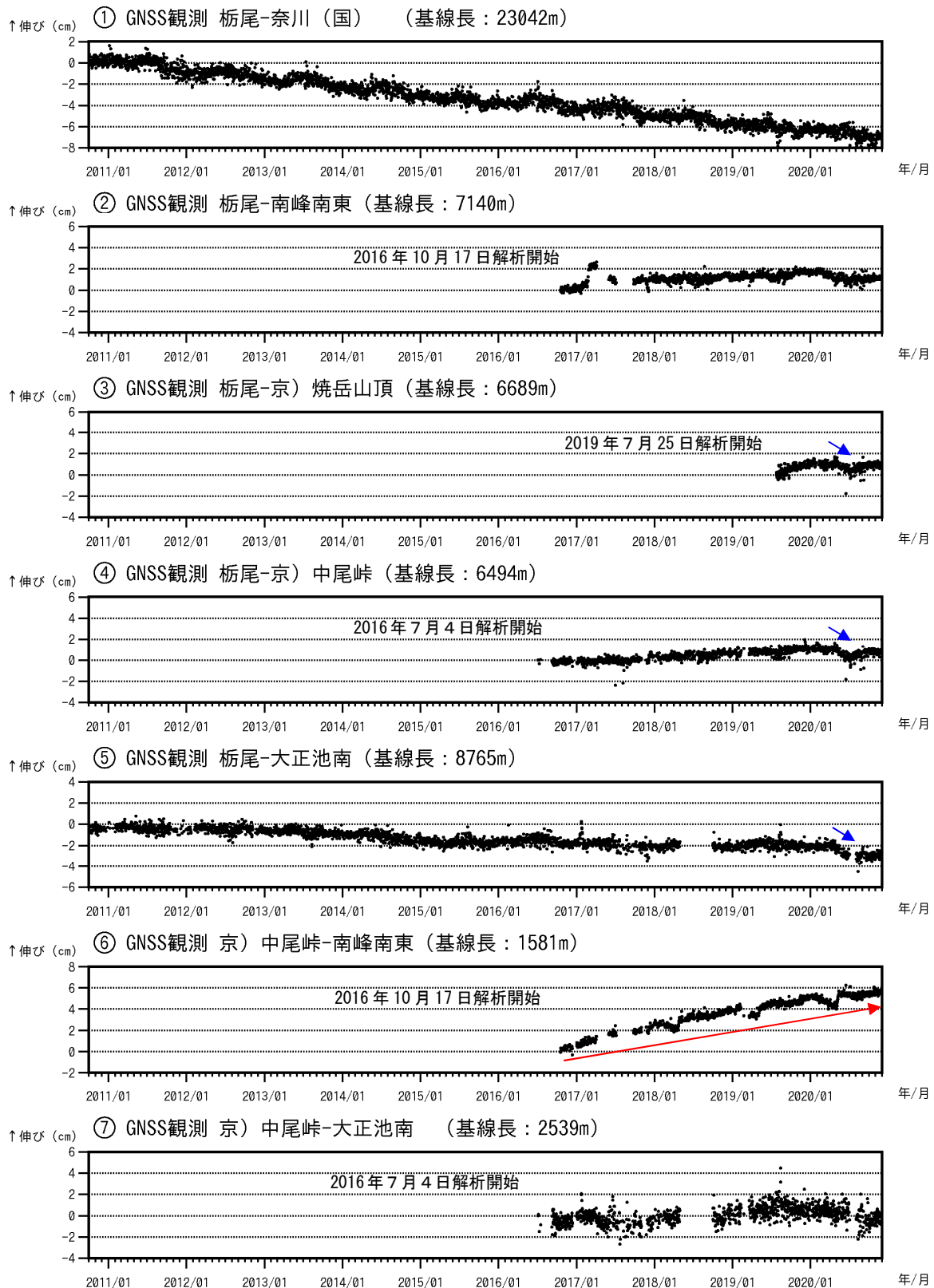
図7 焼岳 GNSS連続観測による基線長変化 (2010年10月1日～2020年11月30日)
