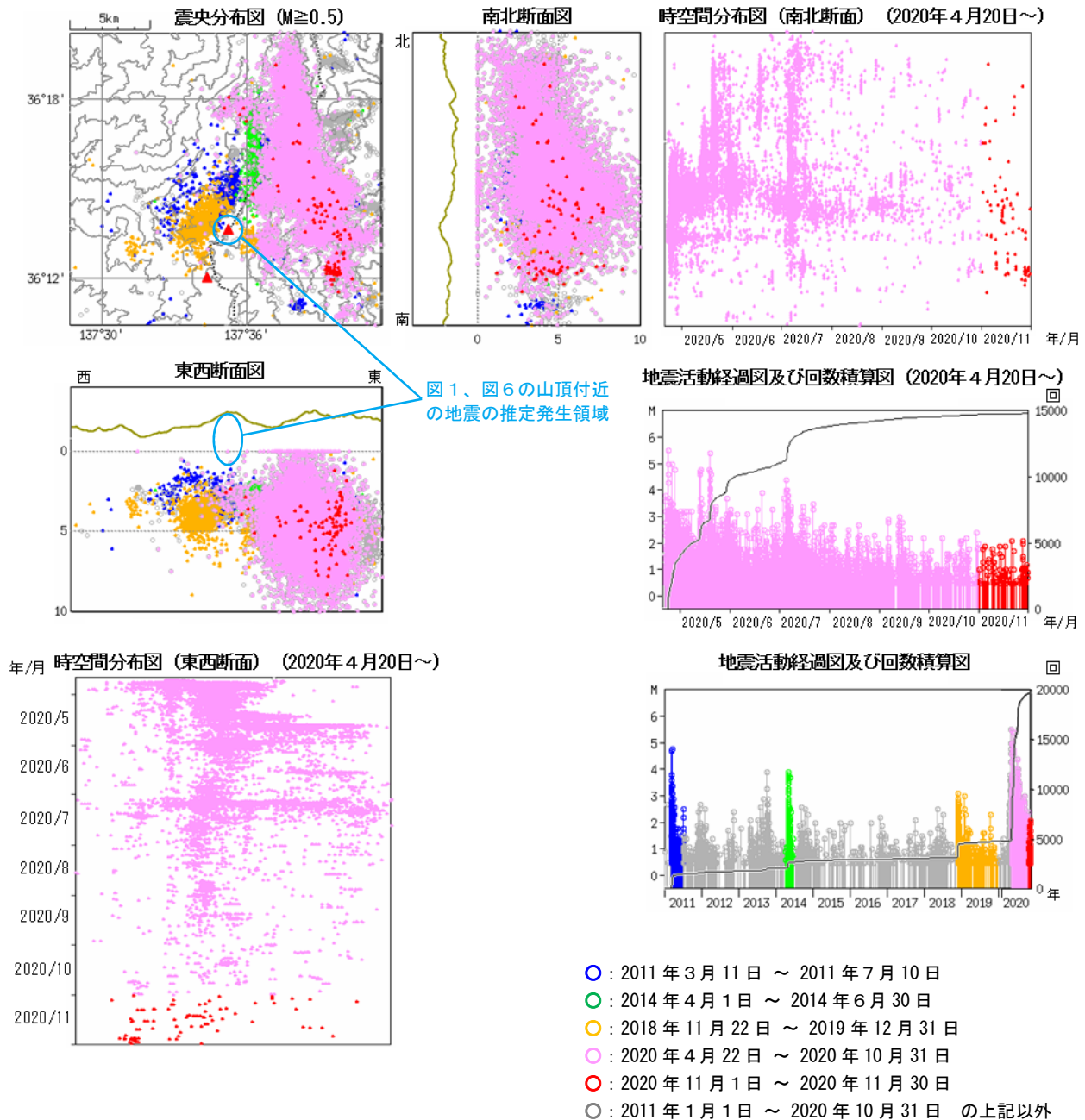
図2 焼岳 広域地震観測網による山体及び周辺の地震活動(2011年1月1日～2020年11月30日)
