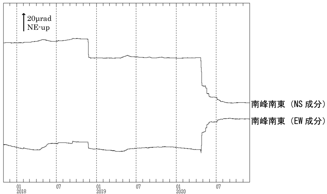
図9 焼岳 南峰南東観測点における傾斜データ（2017年11月1日～2020年11月30日）
