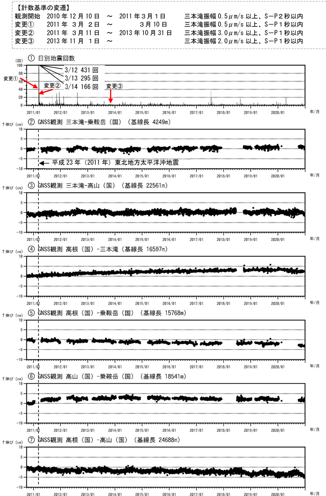
図2 乗鞍岳 火山活動経過図
