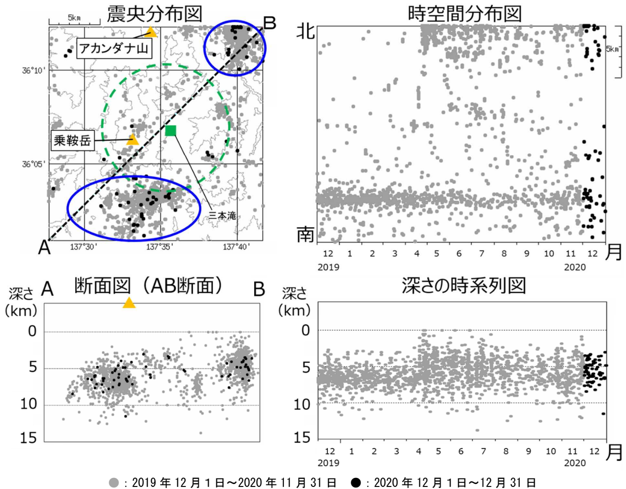
図3 乗鞍岳 広域地震観測網による山体・周辺の地震活動(2019年12月1日~2020年12月31日) 広域地震観測網により震源決定したもので、深さは全て海面以下として決定しています。図中の震源要素は一部暫定値が含まれており、後日変更することがあります。 この図では、関係機関の地震波形を一元的に処理し、地震観測点の標高を考慮する等した新手法で得られた震源を用いています(ただし、2020年8月以前の地震については火山活動評価のための参考震源です)。 2021年1月12日現在、2020年4月18日から10月23日までの地震について、暫定的に震源精査の基準を変更しているため、その前後の期間と比較して微小な地震での震源決定数の変化(増減)が見られます。 震央分布図中の緑点線円は、図2①で計数される地震のおおよその範囲を示します。
