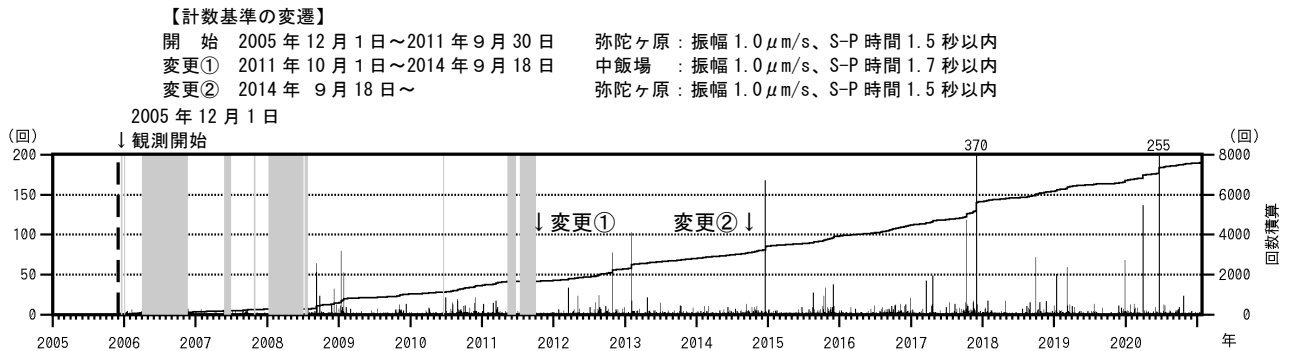
図3 白山 日別地震回数と積算回数（2005年12月1日～2021年1月31日）
