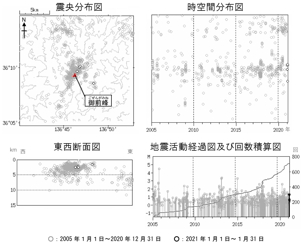
図4 白山 広域地震観測網による山体・周辺の地震活動（2005年1月1日～2021年1月31日）
