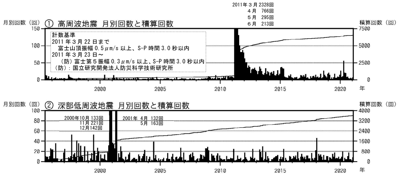
図2 富士山 月別地震回数（1995年6月1日～2021年1月31日）
