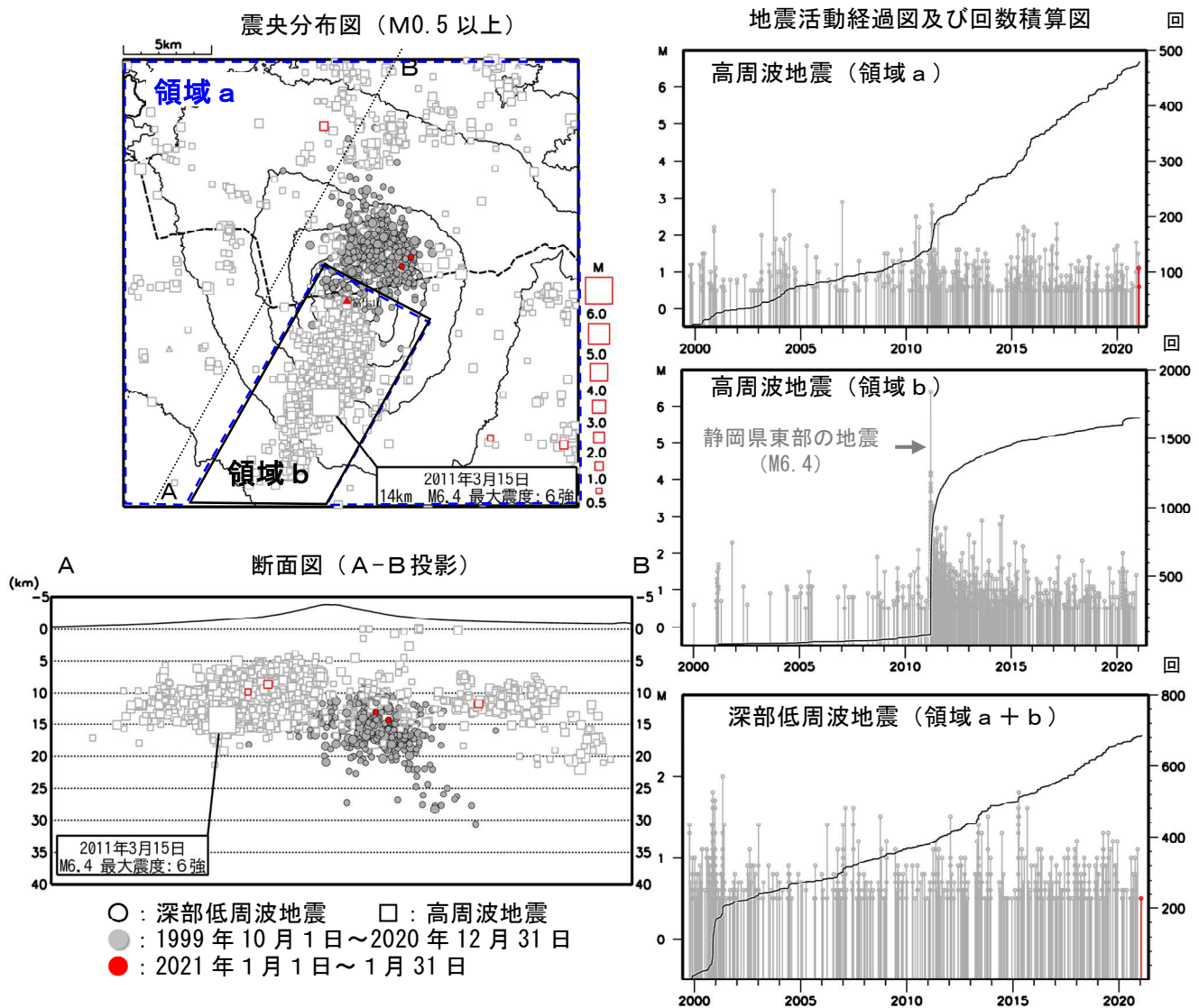
図3 富士山 広域地震観測網による山体及び周辺の地震活動(1999年10月1日～2021年1月31日)
