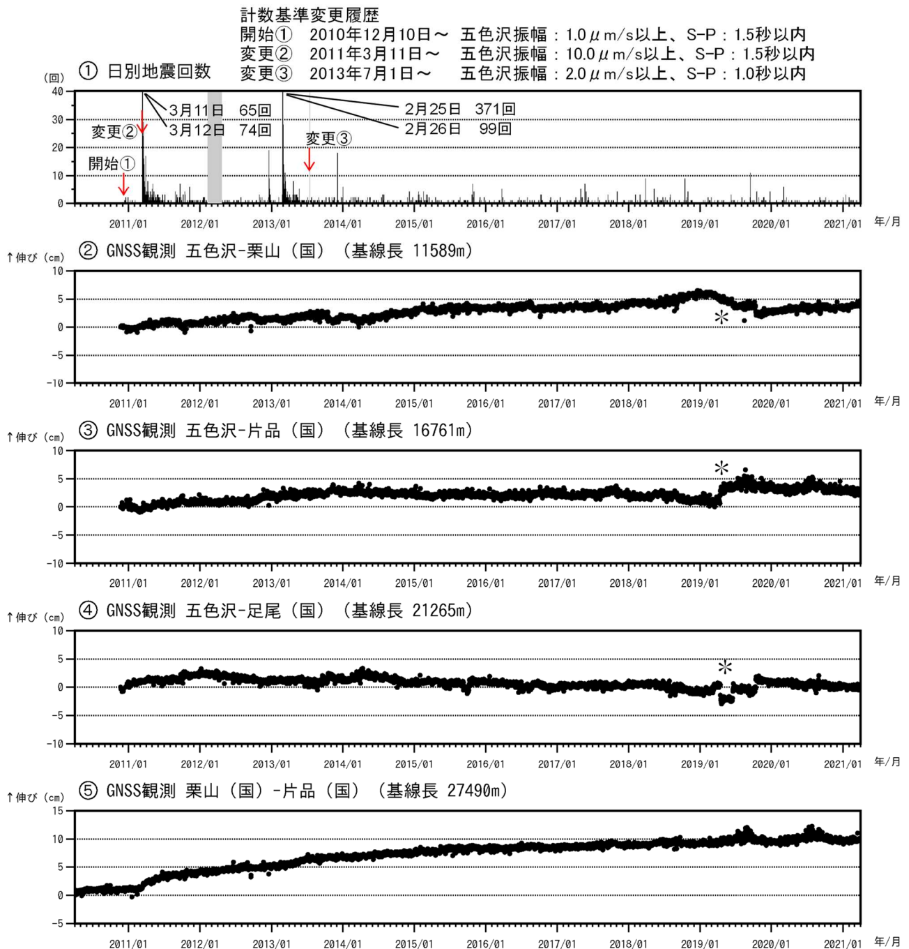
図2 日光白根山 火山活動経過図（2010年4月1日～2021年3月31日）
