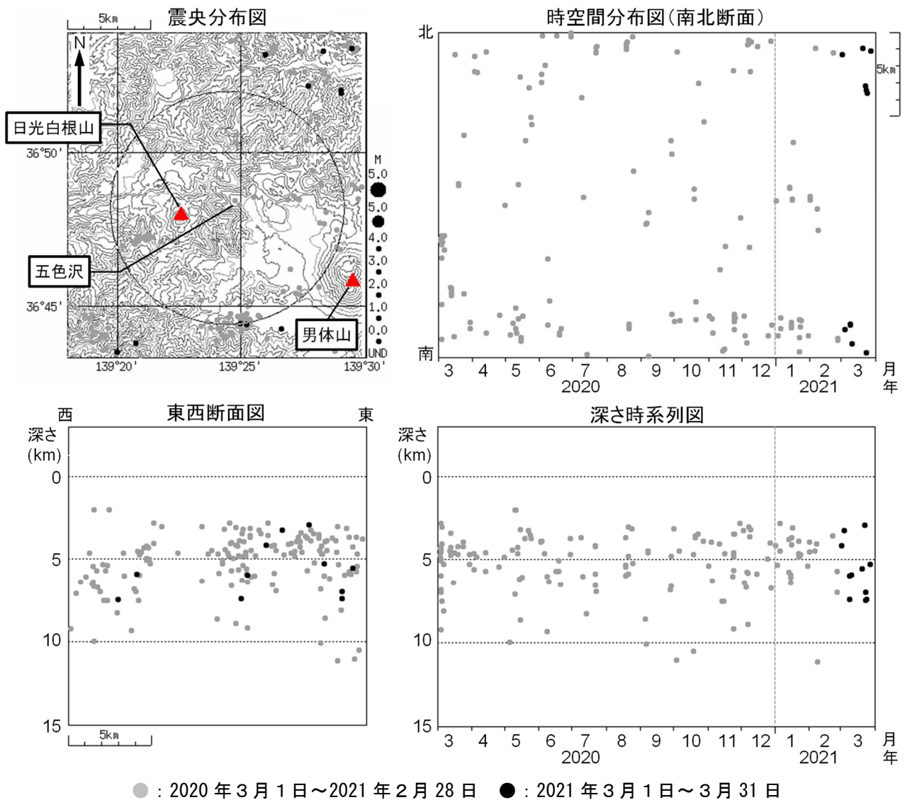
図3 日光白根山 広域地震観測網による山体・周辺の地震活動
